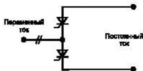
Пример однофазного моста Гретца
