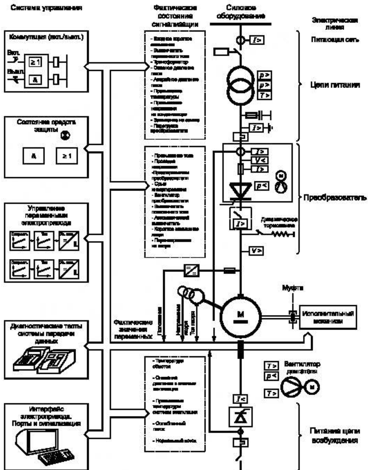
Рисунок 1 — Функциональная схема электропривода постоянного тока
