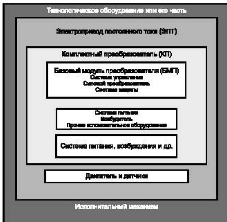
Рисунок 2 — Аппаратные составляющие ЗПТ
