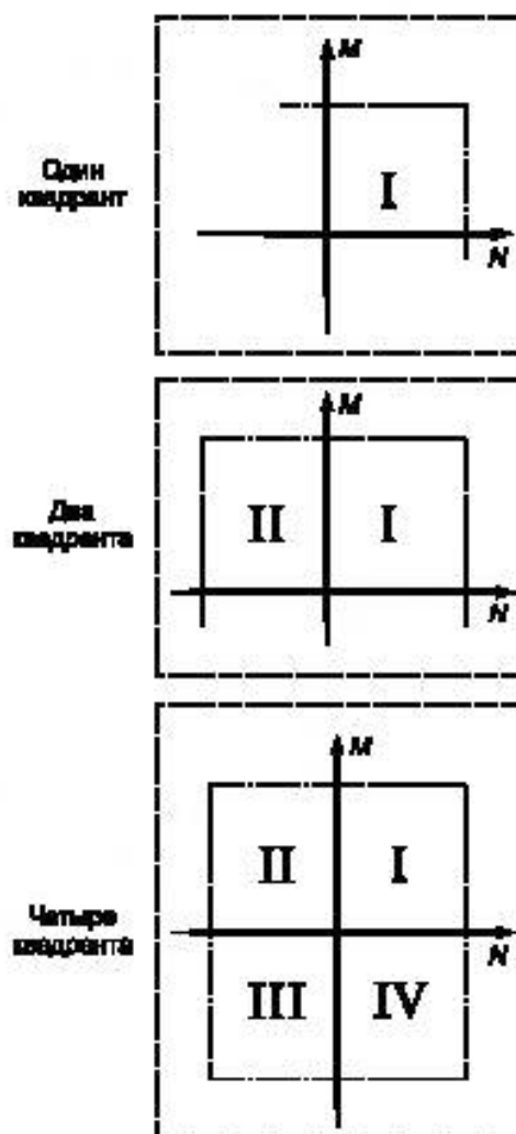
Рисунок 3 — Рабочие квадранты работы электропривода
