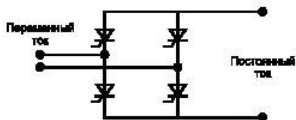
Пример однофазного моста Гретца
