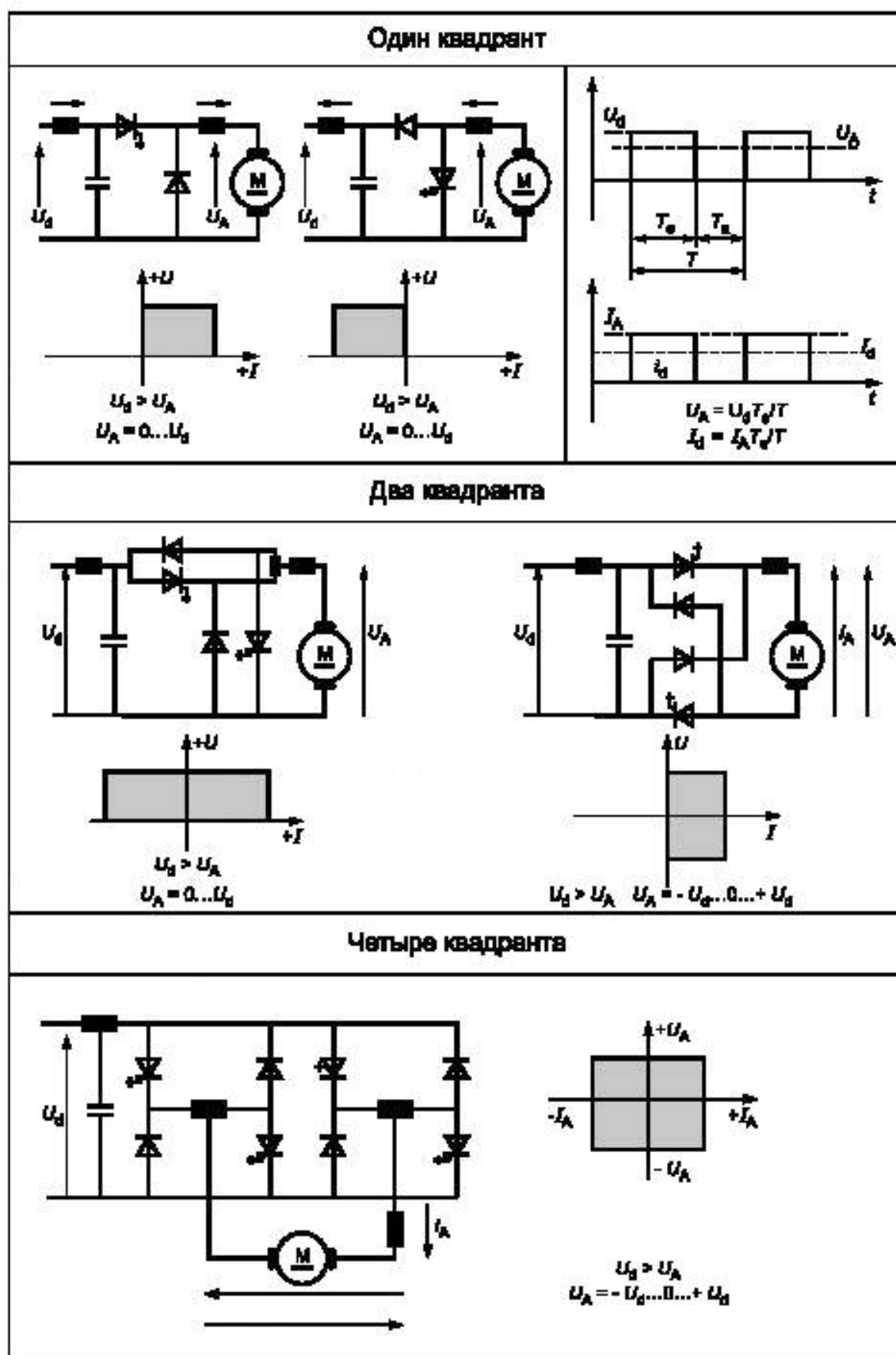
Рисунок F.2 — Преобразователи с внутренней коммутацией (прерыватели)
