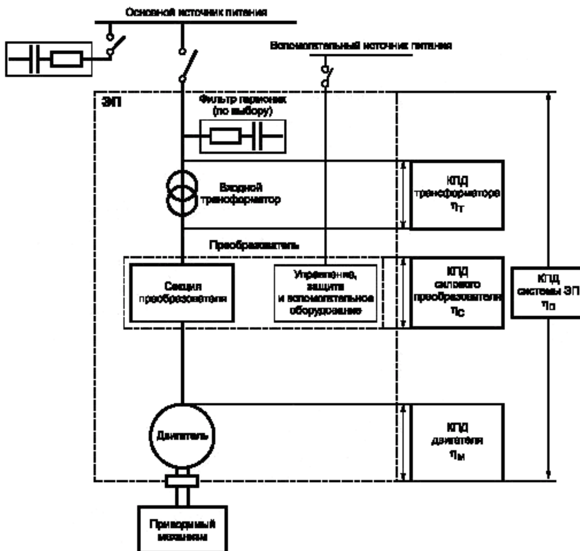
Рисунок 25 — Элементы системы силового ЭП и их КПД
