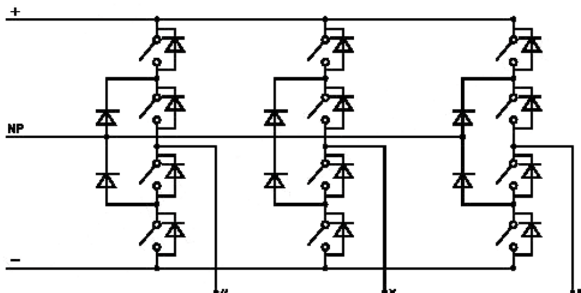
Рисунок A.7 — Схема инвертора с выведенной нейтралью
