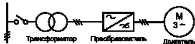
Рисунок 4 — Общая структура системы привода с непосредственным преобразователем
