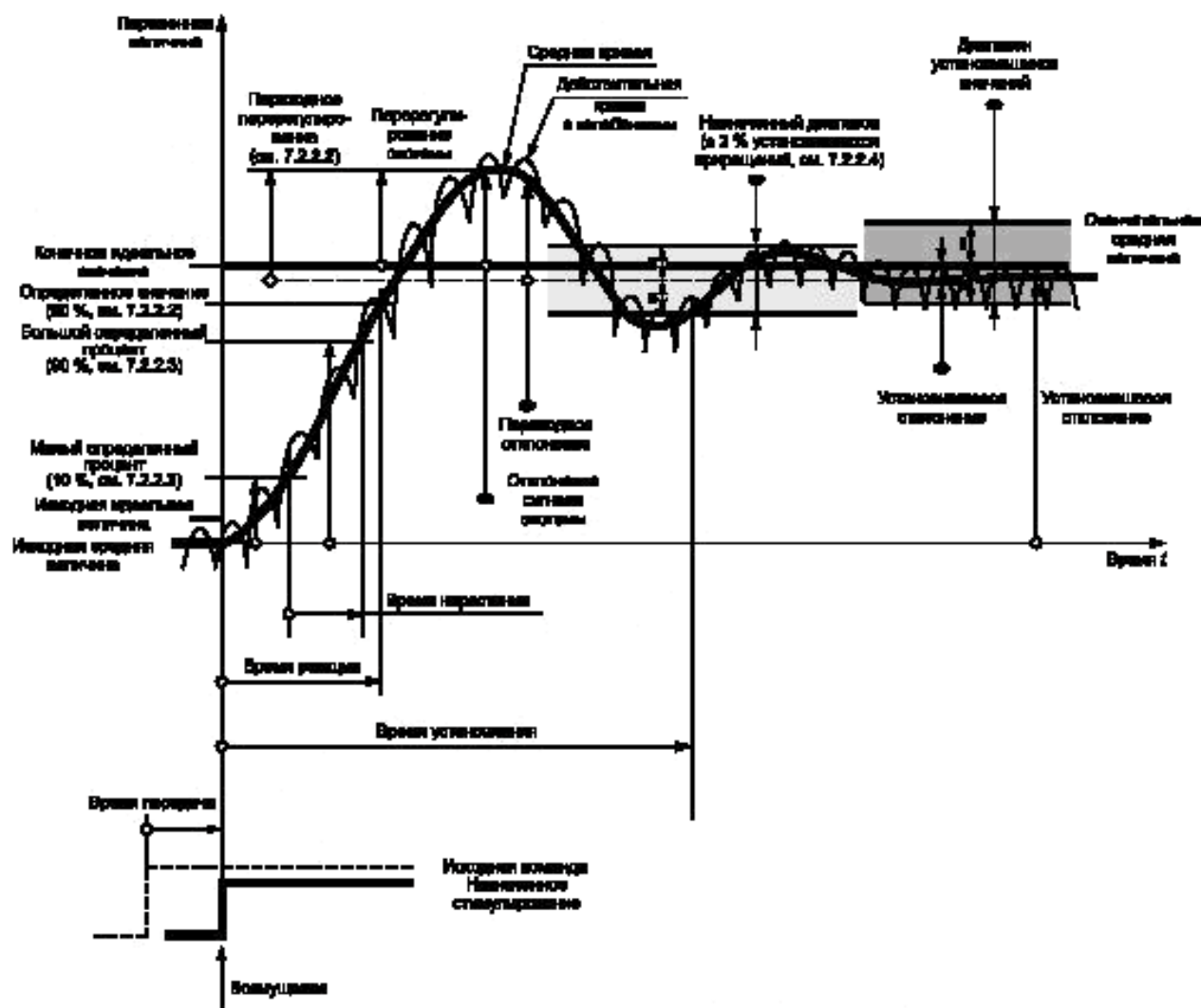
Рисунок 12 — Реакция во времени на скачкообразное изменение типового входа — рабочие показатели не изменяются
