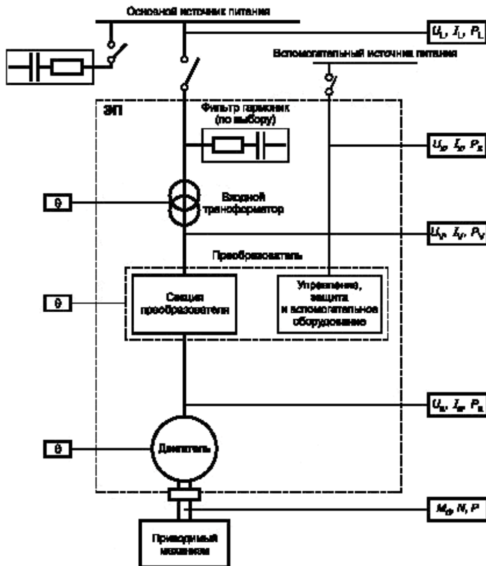
Рисунок 23 — Точки измерения для испытания системы ЭП
