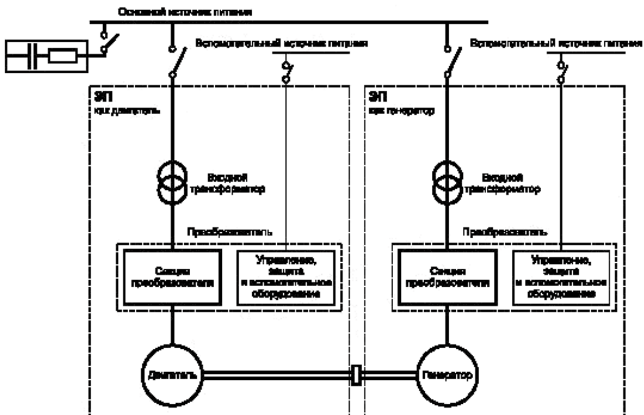
Рисунок 24 — Опыт взаимной нагрузки
