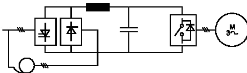
Рисунок A.10 — Трехфазный инвертор в режиме источника напряжения с реверсивным преобразователем на стороне питающей сети
