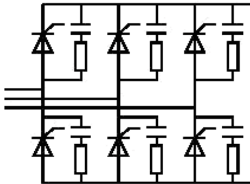
Рисунок С.3 — Трехфазная мостовая схема включения тириستоров
