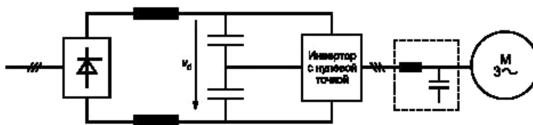
Рисунок A.6 — Система привода с инвертором — источником напряжения, имеющим вывод нейтрали
