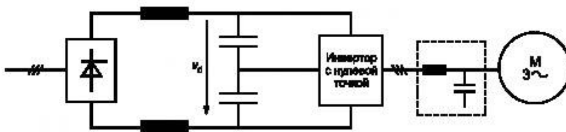
Рисунок А.6 — Система привода с инвертором — источником напряжения, имеющим вывод нейтрали
