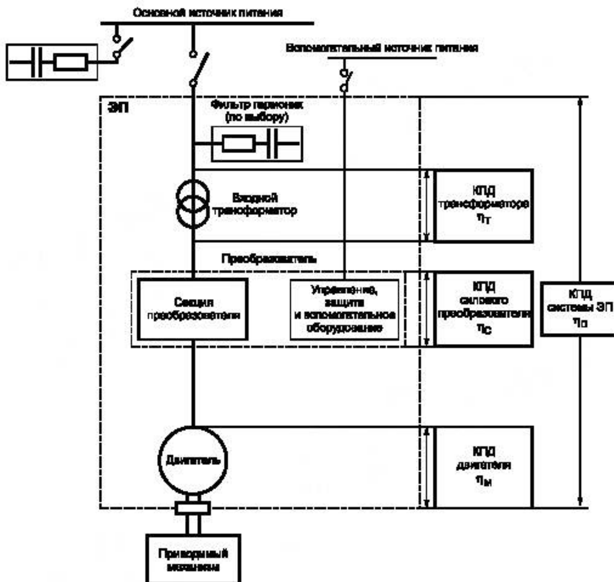
Рисунок 25 — Элементы системы силового ЭП и их КПД
