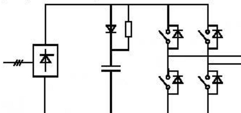
Рисунок С.4 — Снаббер в звене постоянного тока
