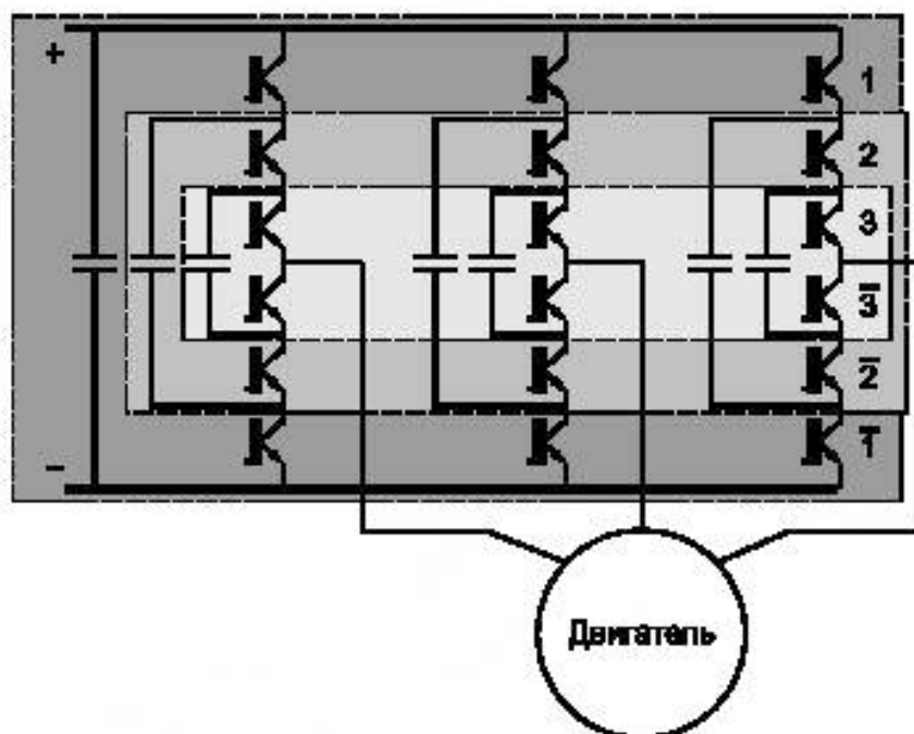
Рисунок A.9 — Схема многоуровневого инвертора
