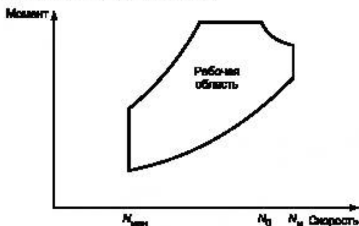
Рисунок 2 — Пример нагрузочной диаграммы
