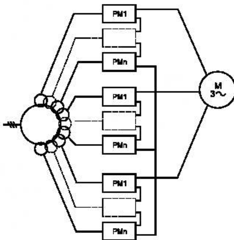
Рисунок A.12 — Система привода с многоуровневым инвертором — источником напряжения
