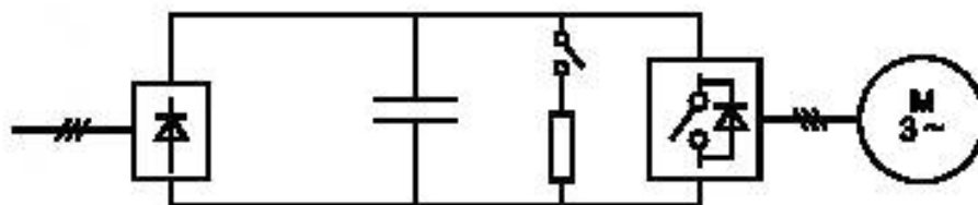
Рисунок 8 — Пример динамического торможения
