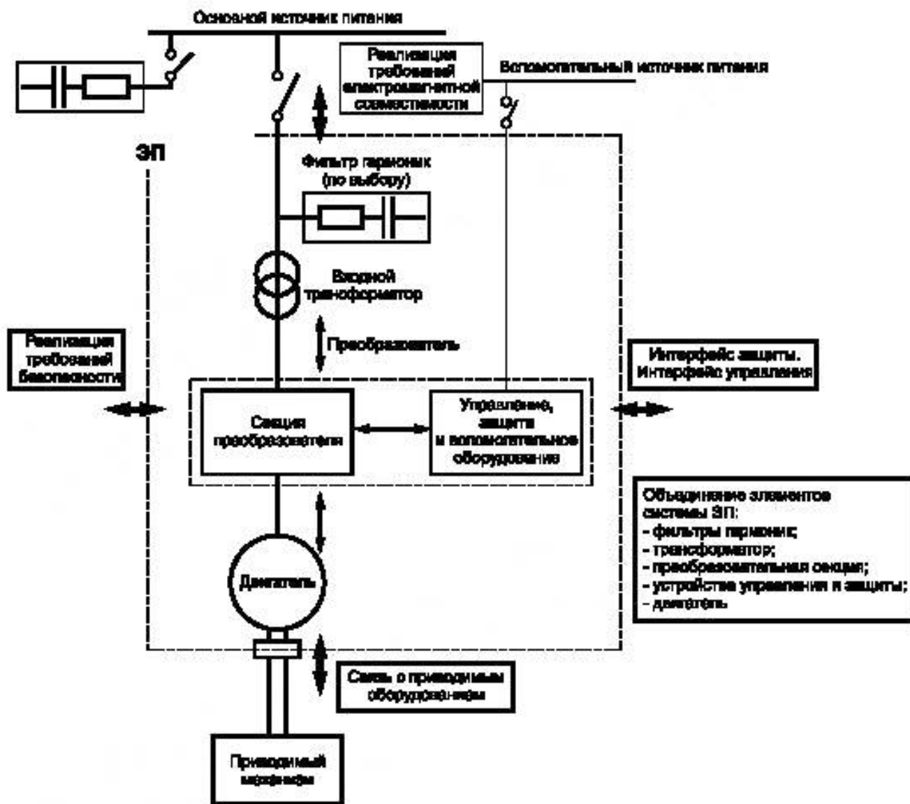
Рисунок 20 — Система силового электропривода — напряжение свыше 1000 В
