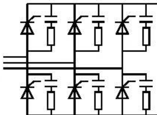
Рисунок С.3 — Трехфазная мостовая схема включения тиристоров
