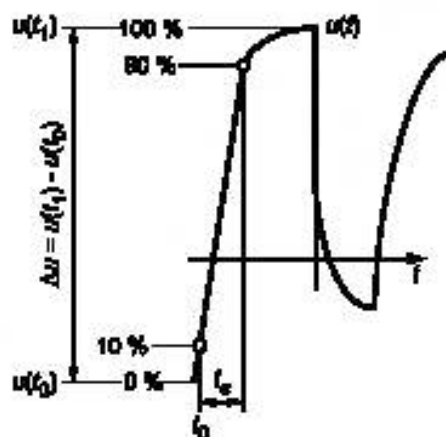
Рисунок 18 — Скачок напряжения при питании от ШИМ-инвертора
