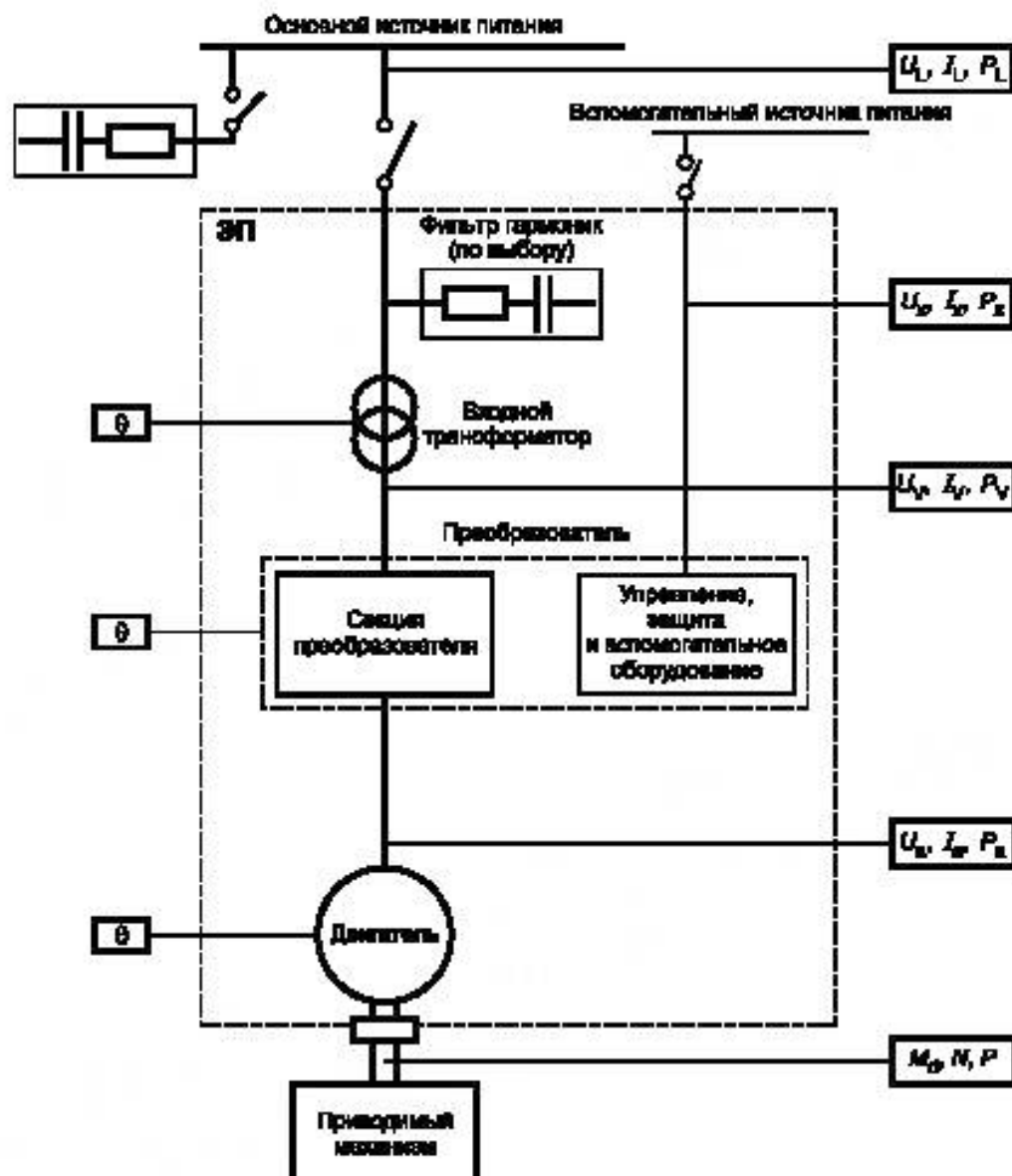
Рисунок 23 — Точки измерения для испытания системы ЭП
