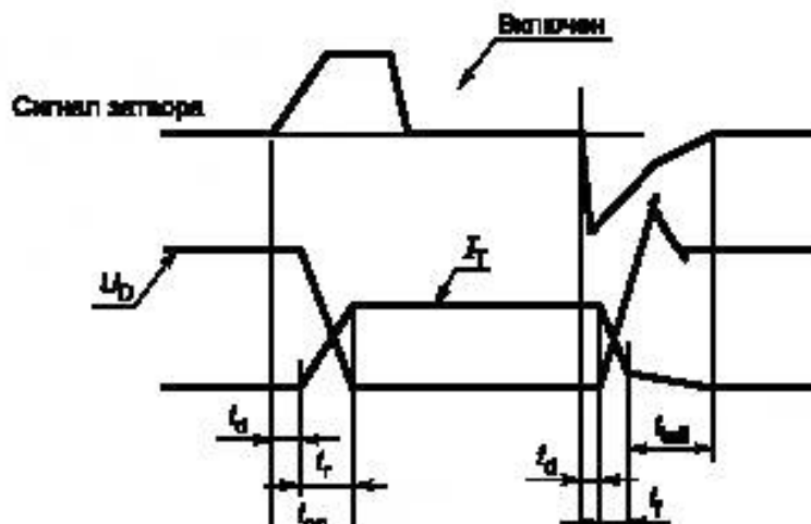
Рисунок С.1 — Формы кривых при коммутации GTO/GCT
