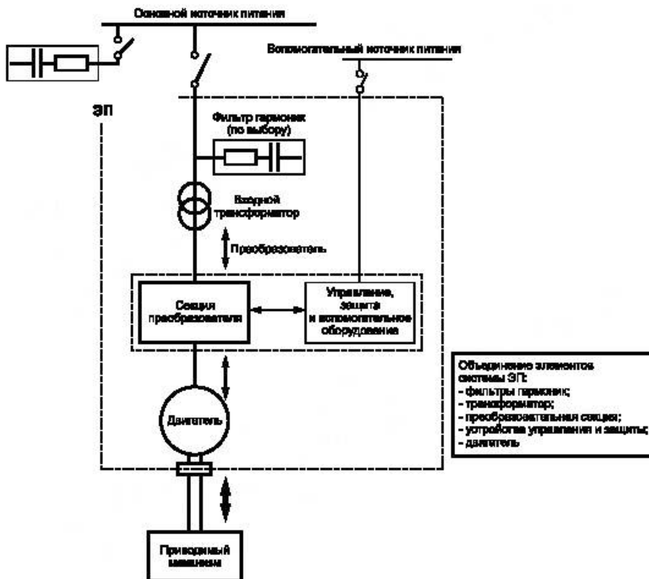
Рисунок 21 — Система силового электропривода
