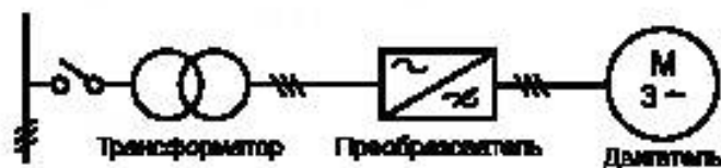
Рисунок 4 — Общая структура системы привода с непосредственным преобразователем
