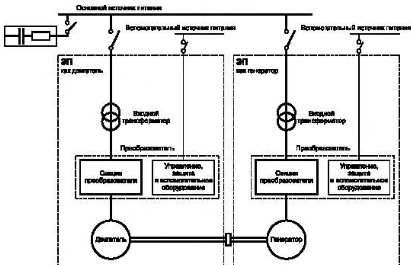
Рисунок 24 — Опыт взаимной нагрузки
