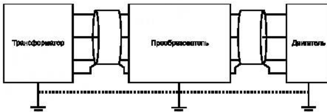
Рисунок 22 — Пример защитного заземления и соединения основных компонентов
