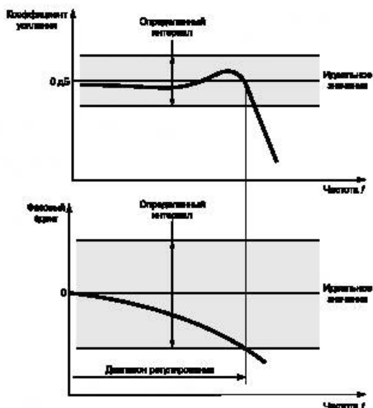
Рисунок 15 — Частотные характеристики при управлении — базовое значение возмущения
