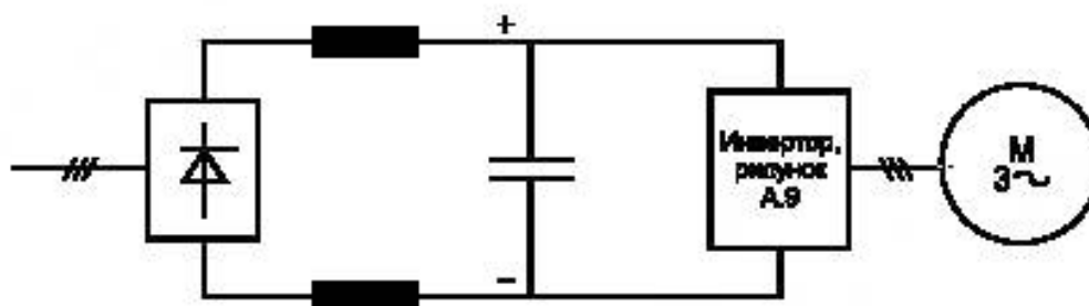
Рисунок A.8 — Система электропривода с многоуровневым инвертором в режиме источника напряжения
