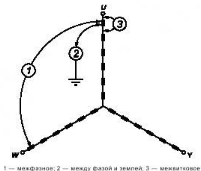
Рисунок 17 — Виды перенапряжений на изоляции
