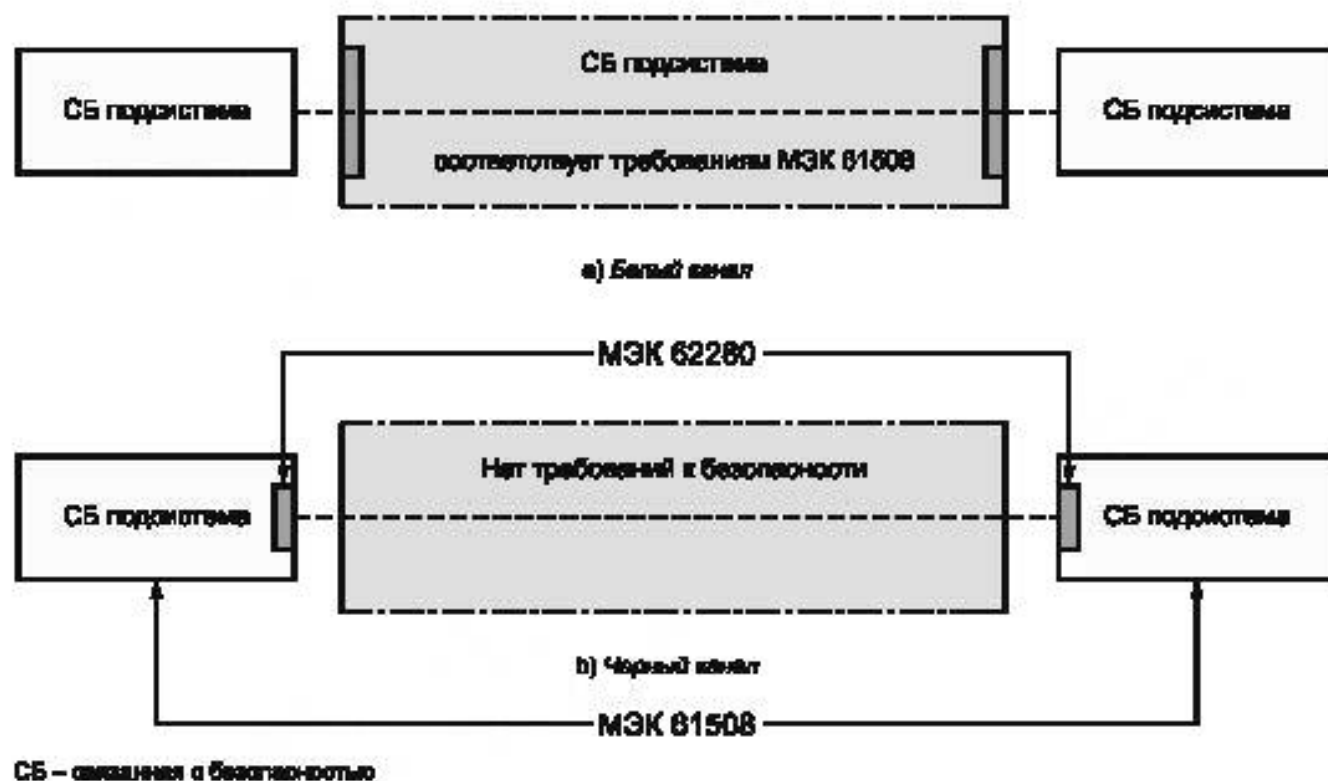
Рисунок 3 — Архитектуры для передачи данных
