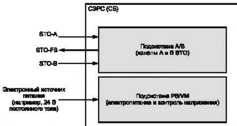
Рисунок В.2 — Подсистемы СЭРС (СБ)
