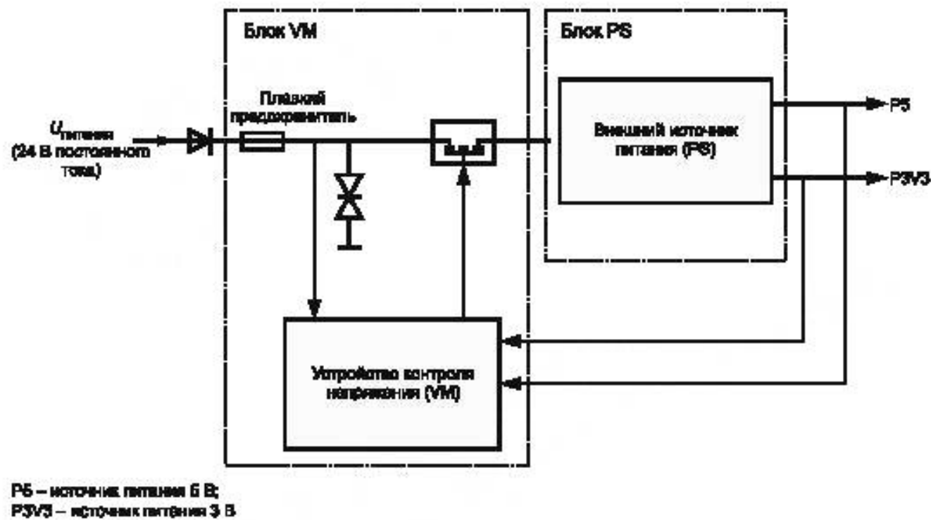
Рисунок В.5 — Функциональные блоки подсистемы PS/VM
