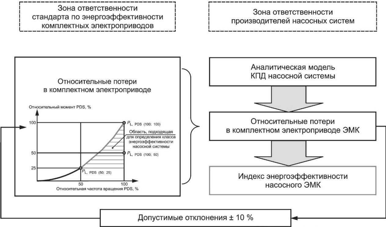
Рисунок А.2 — Пример совместного использования квазианалитических моделей комплектного преобразователя и насосной системы для оценки индекса энергоэффективности насосного ЭМК
