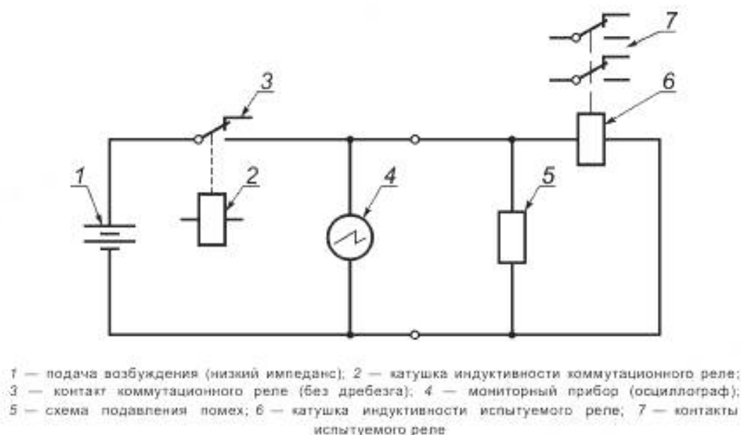
Рисунок 1 — Типичная схема измерения подавления переходных помех катушки
