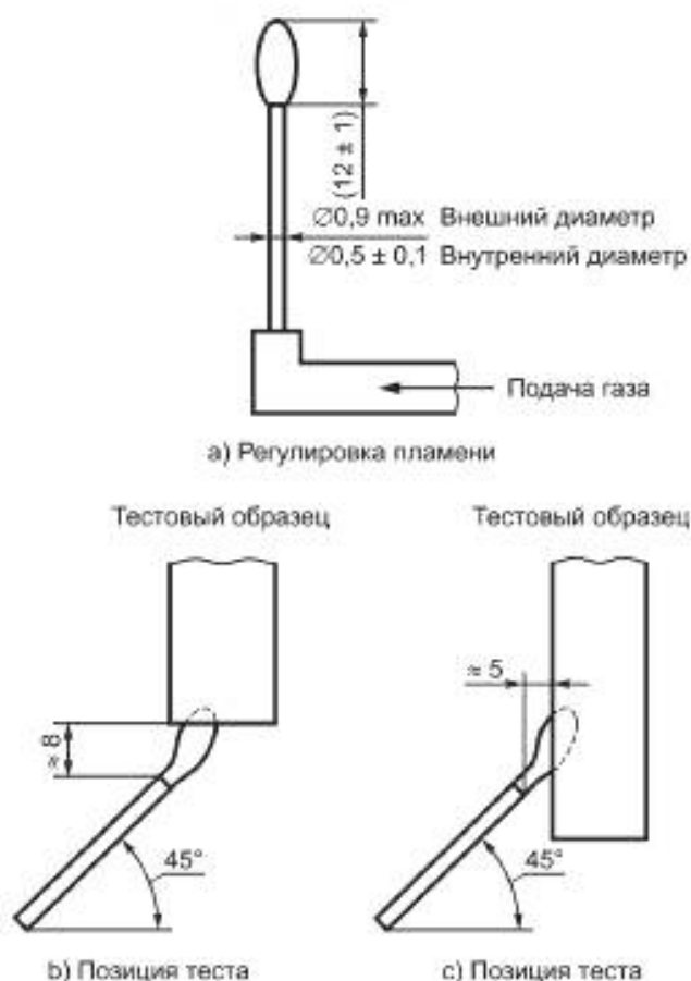
Рисунок В.3 — Детали испытания игольчатым пламенем
