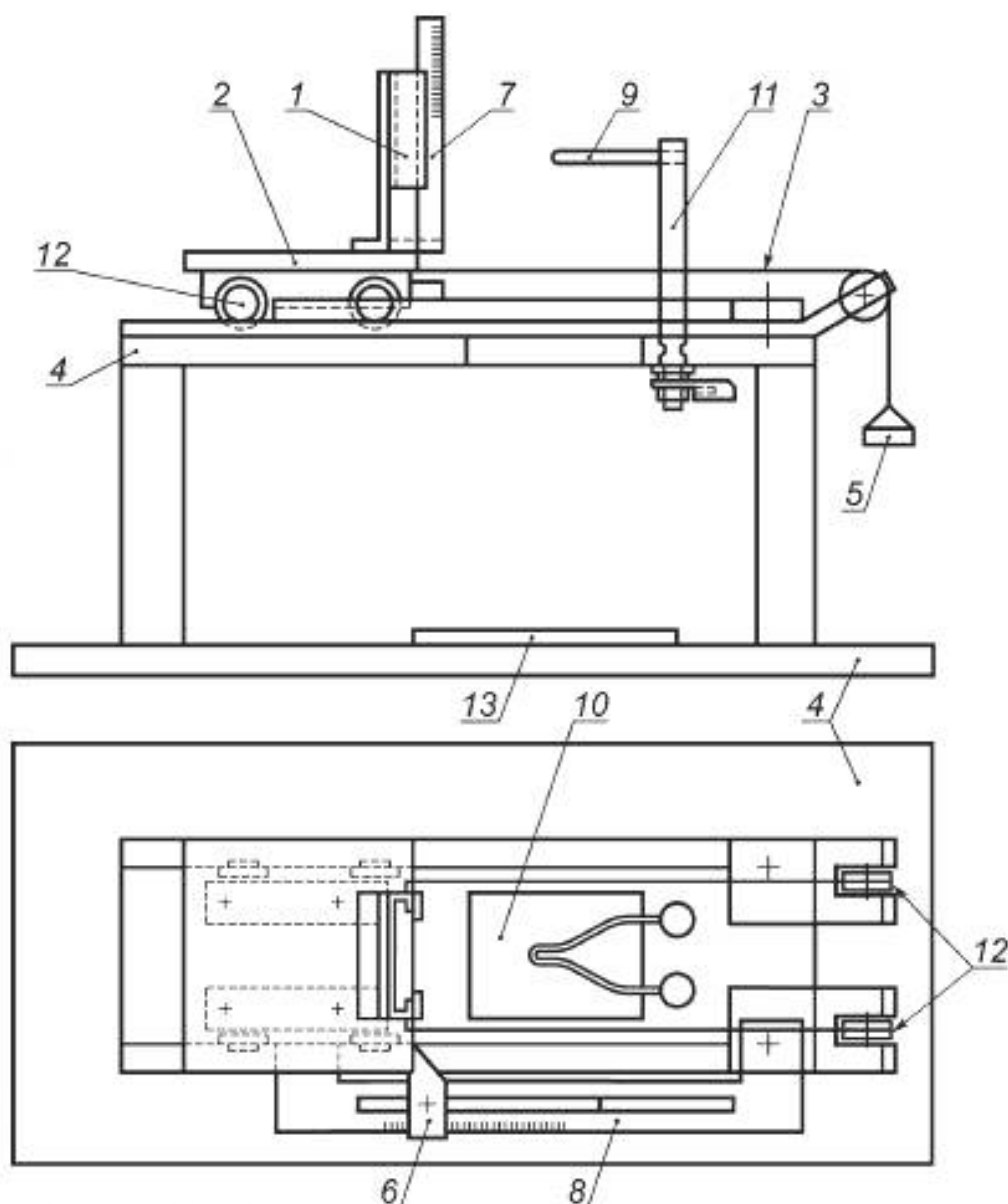
1 — опора тестового образца; 2 — каретка; 3 — опорный корд; 4 — базовая плата; 5 — вес; 6 — регулируемый стопор; 7 — шкала для измерения высоты пламени; 8 — настройка проникновения; 9 — раскаленная проволока; 10 — срез базовой платы для падающих частиц; 11 — штырь для монтажа раскаленной проволоки; 12 — роллеры с низким трением; 13 — управлятель
