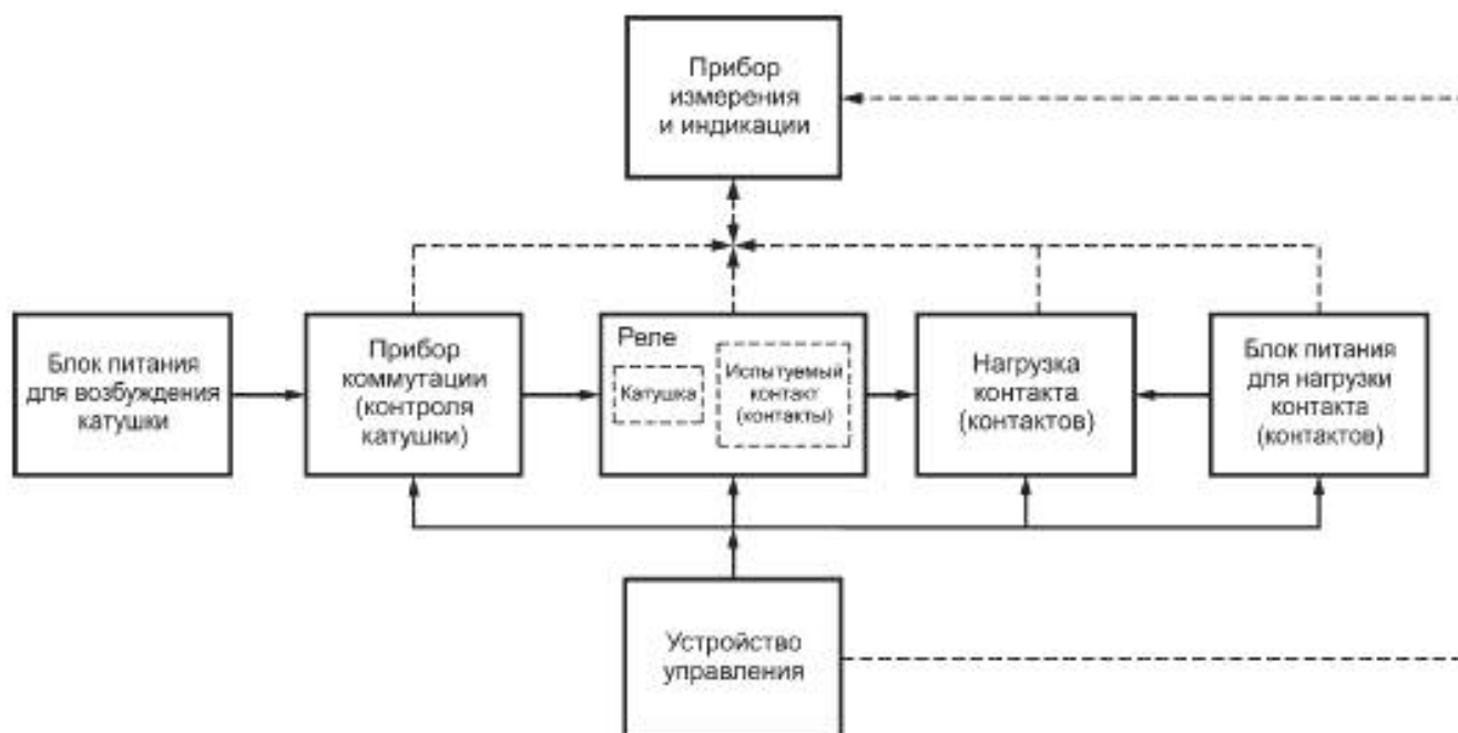
Рисунок С.2 — Функциональная блок-схема
