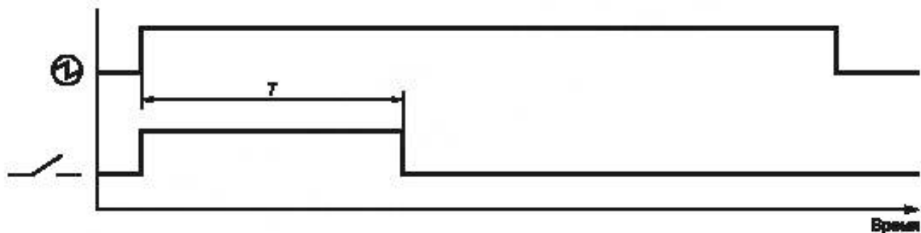
Рисунок 12 — Реле интервала
