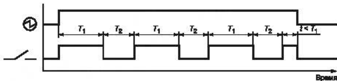
Рисунок 7 — Проблесковое реле
