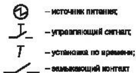
Рисунок 2 — Определение символов
