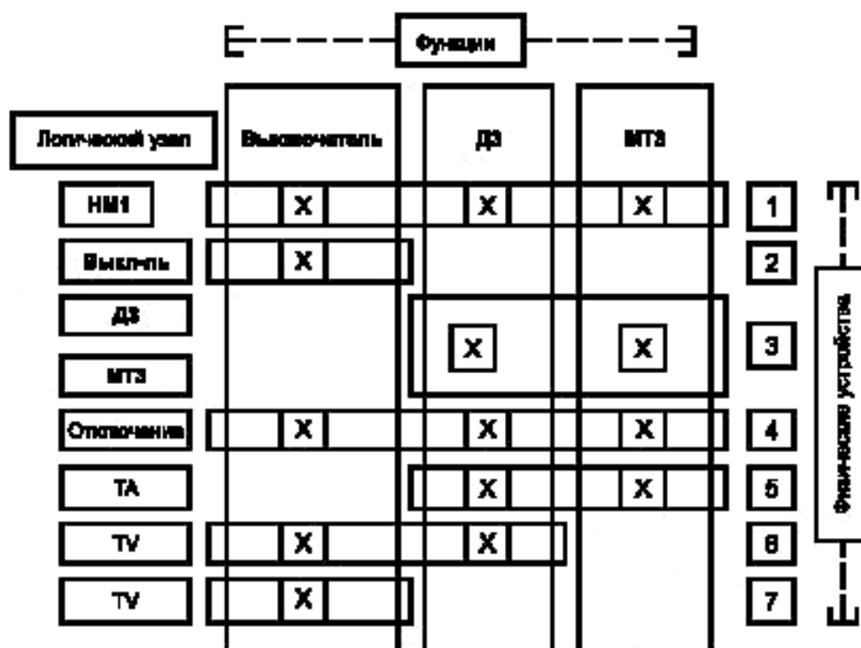
Рисунок 4 — Примеры применения концепции логического узла
