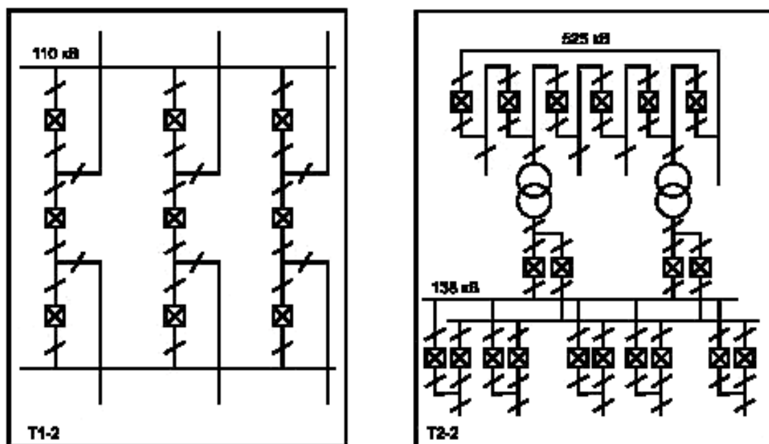
Рисунок 1.2 — Магистральная подстанция малого размера T1-2 с полуторной схемой и магистральная подстанция большого размера T2-2 с кольцевой системой сборных шин
