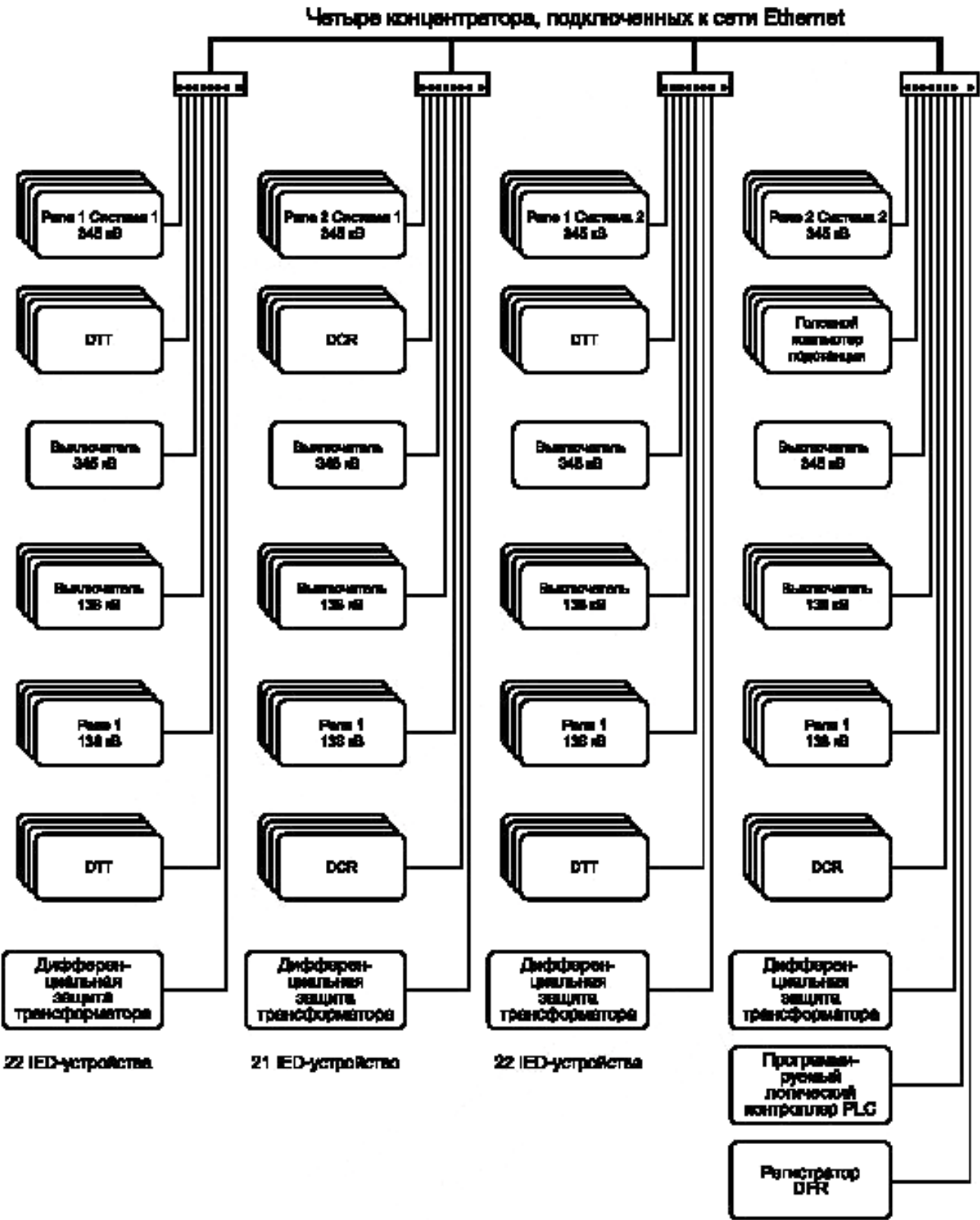
Рисунок 1.10 — Конфигурация сети Ethernet с коммутируемым концентратором
