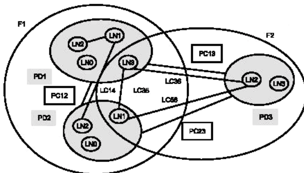
Рисунок 3 — Концепция логического узла и связи
