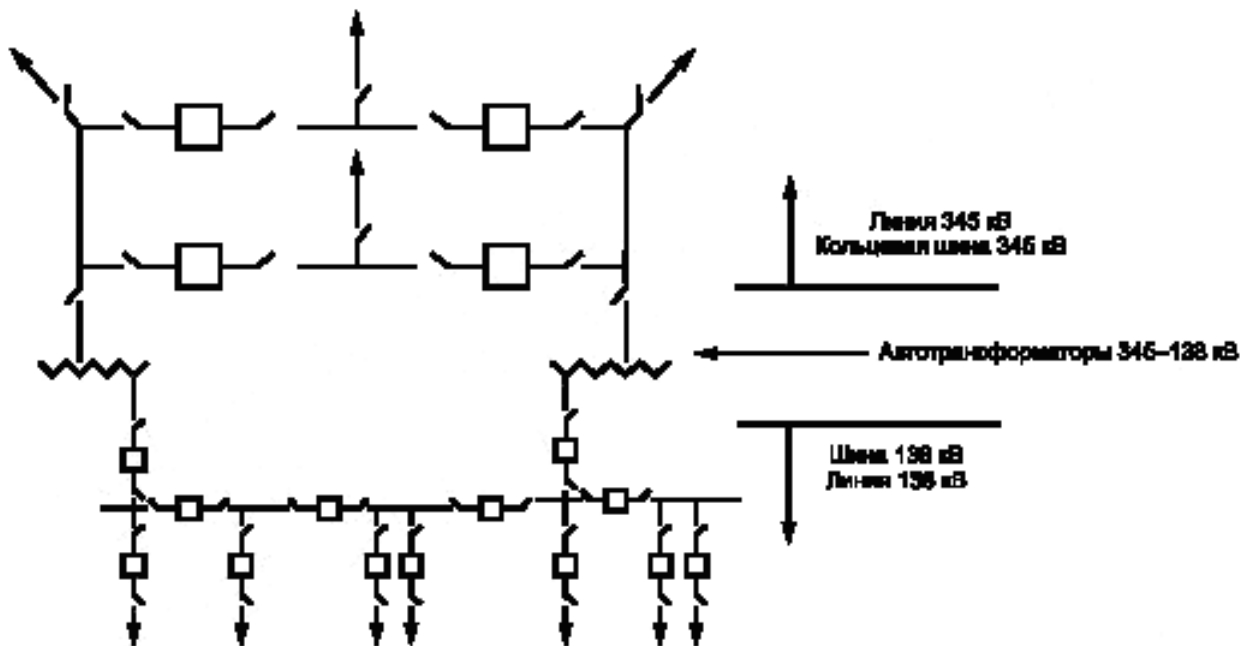
Рисунок I.8 — Подстанция магистральной сети большой мощности с кольцевой топологией, аналогичная T2-2
