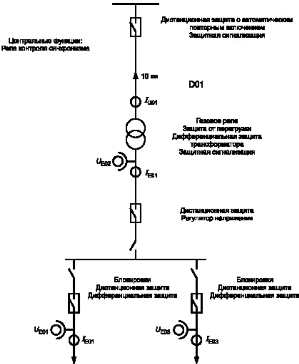
Рисунок I.3 — Подстанция типа T1-1 с распределением функций
