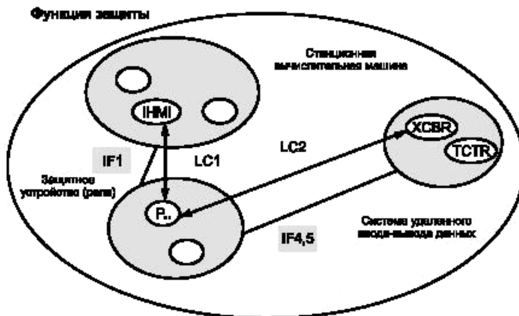
Рисунок 5 — Функция защиты, состоящая из трех LN
