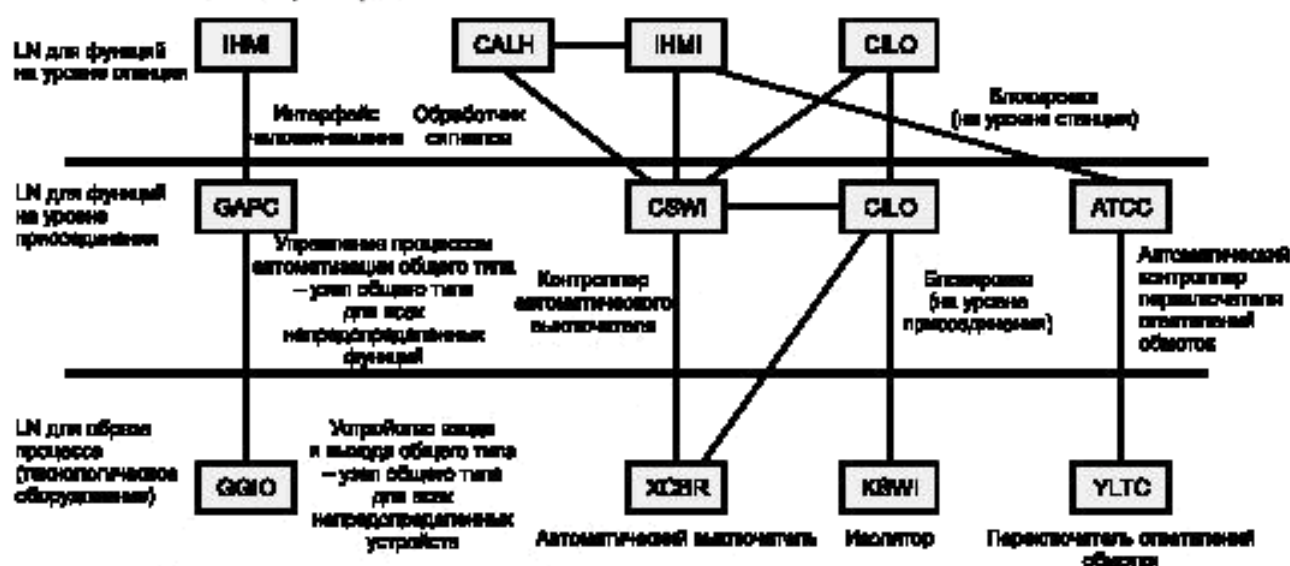
Рисунок 7 — Разложение функций на взаимодействующие LN на различных уровнях: примеры функции общего вида для автоматизации, функция управления выключателем и функция управления напряжением
