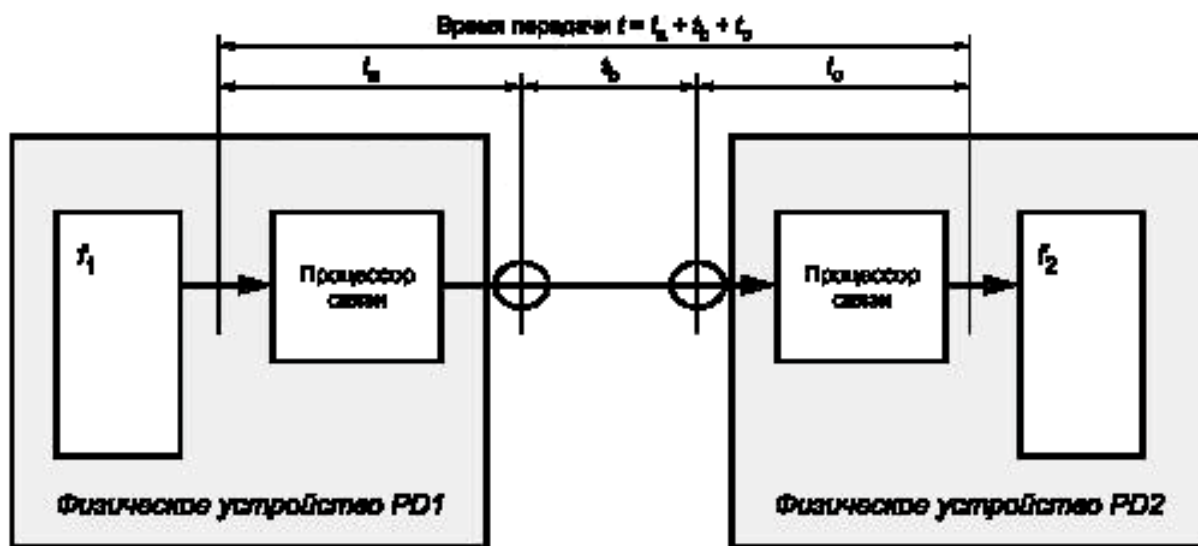
Рисунок 16 — Определение времени передачи
