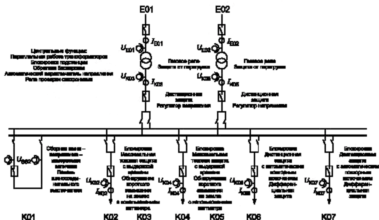
Рисунок I.4 — Подстанция типа D2-1 с распределением функций
