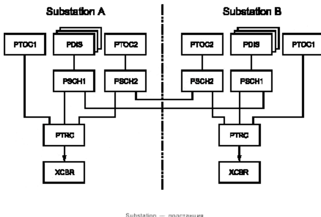
Рисунок В.2 — Использование логических узлов PSCH и PTRC
