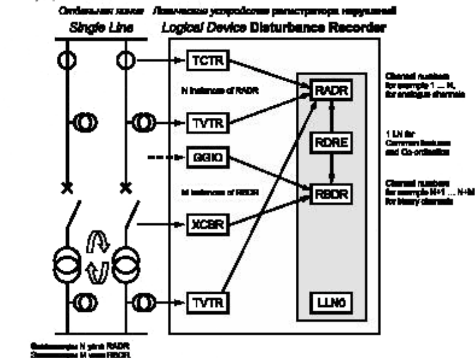
Рисунок В.4 — Моделирование регистратора нарушений
