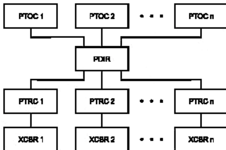
Рисунок B.6 — Использование логического узла PDIR
