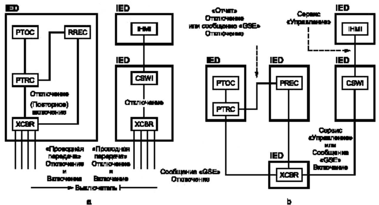
Рисунок В.7 — Использование логического узла RREC
