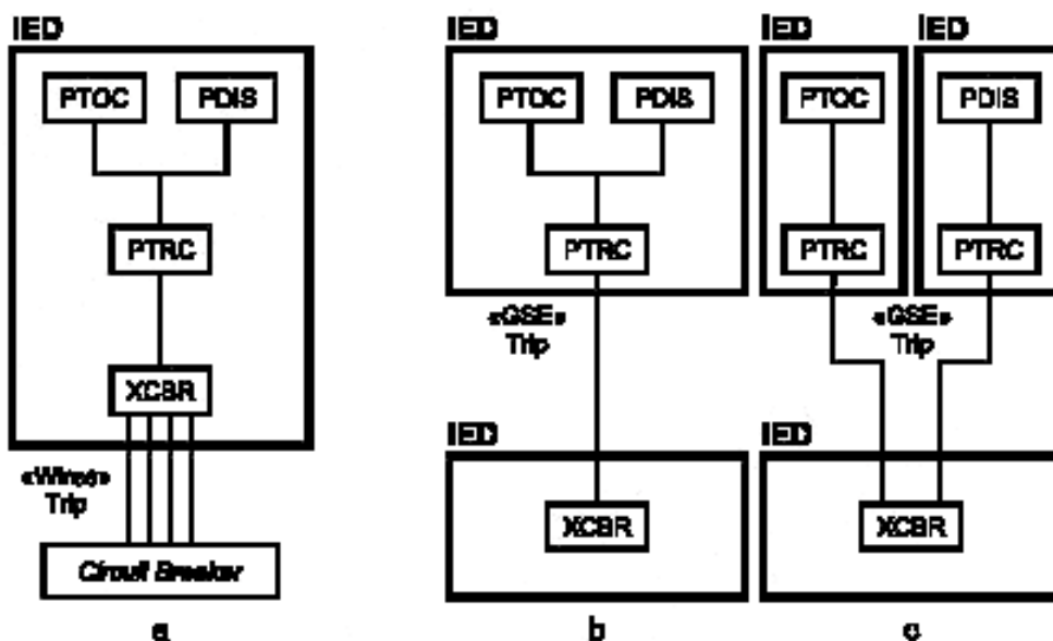
Рисунок B.5 — Пример назначения логических узлов IED-устройствам
