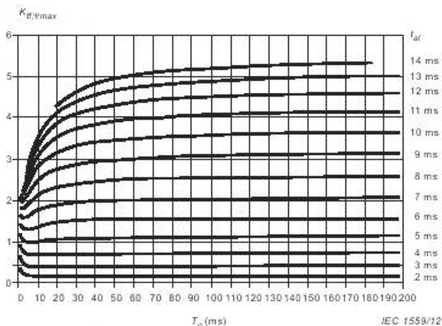
Рисунок 2В.4 — Определение K_{If} в диапазоне времени 1 при 50 Гц для T_s = 1,8 с
