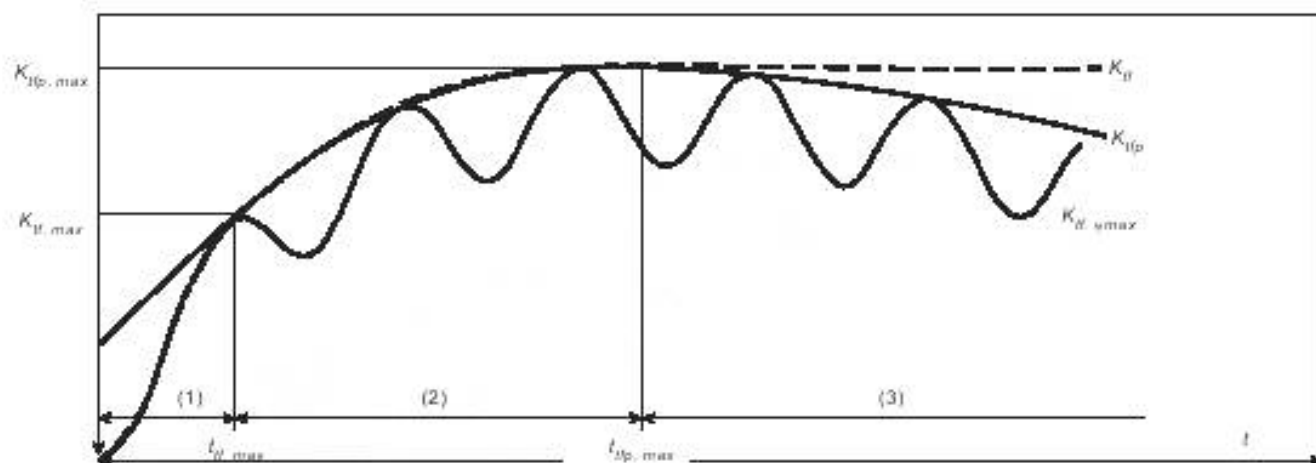
Рисунок 2В.3 — Соответствующие диапазоны времени для расчета коэффициента
