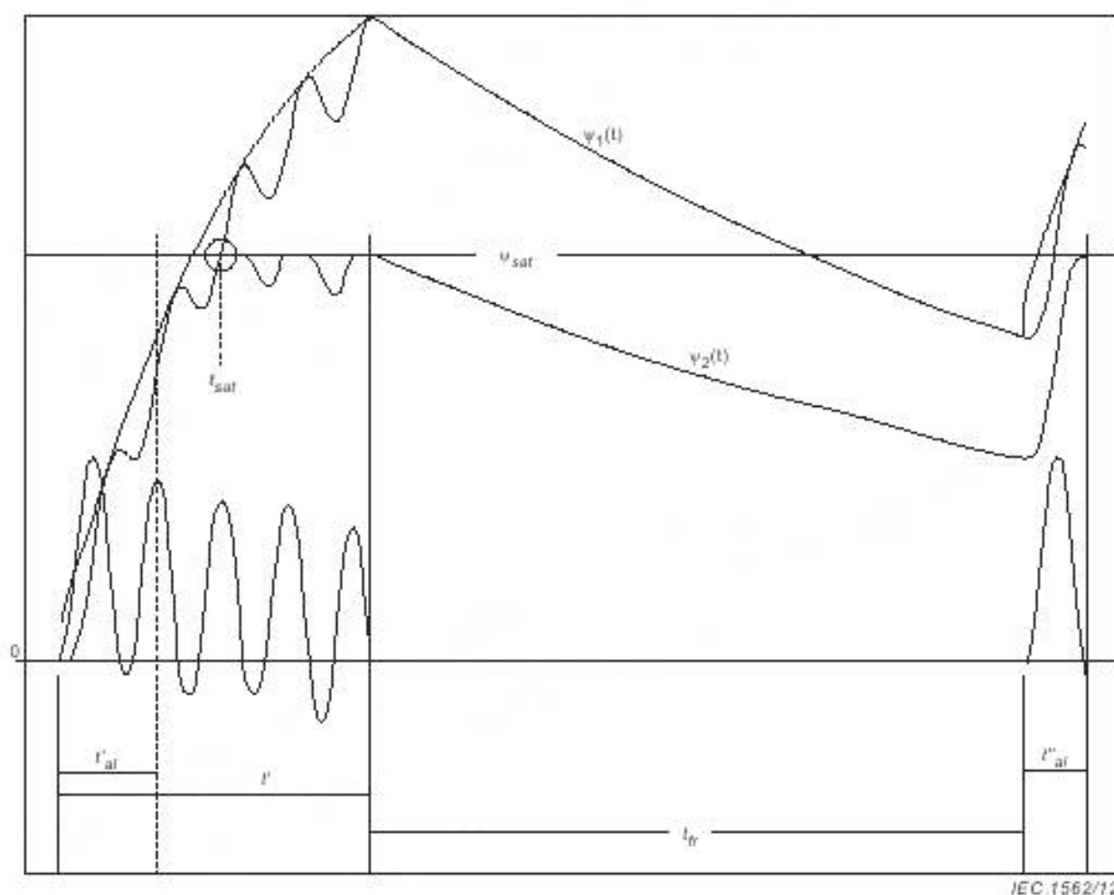
Рисунок 2B.7 — Ограничение магнитного потока, с учетом насыщения катушки
