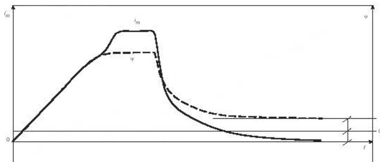
Рисунок 2B.12 — Зарегистрированные значения со смещенными исходными значениями потока
