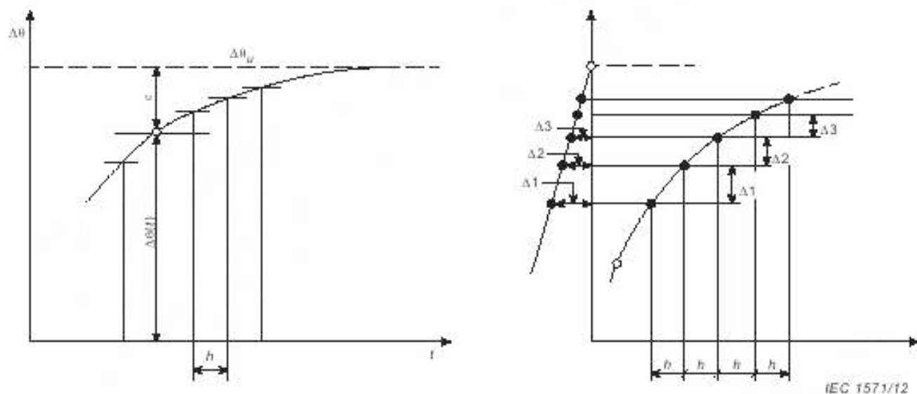
Рисунок 2D.1 — Графическая экстраполяция к окончательному превышению температуры
