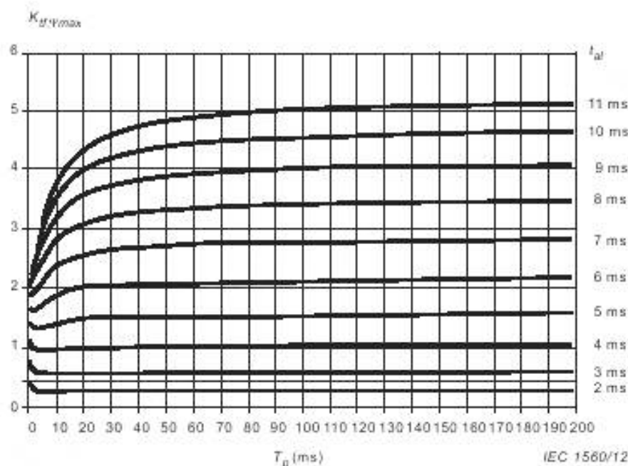
Рисунок 2B.5 — Определение K_U в диапазоне времени 1 при 60 Гц для T_s = 1,5 с
