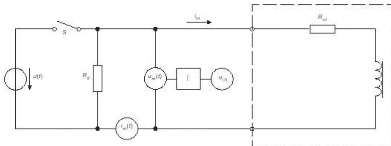
Рисунок 2В.10 — Схема метода постоянного тока
