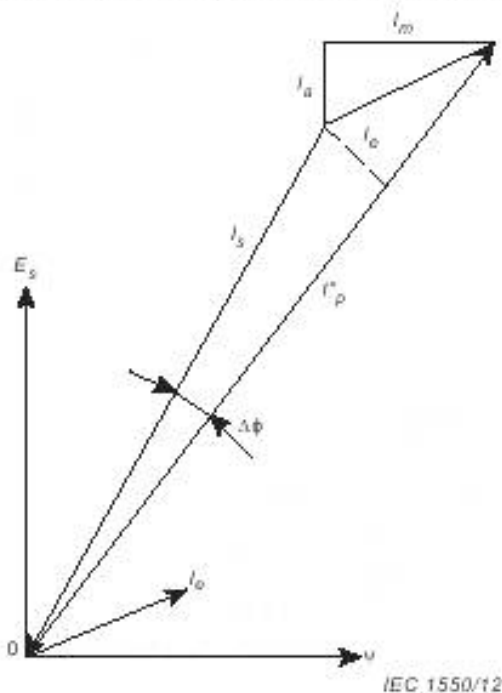
Рисунок 2А.1 — Векторная диаграмма
