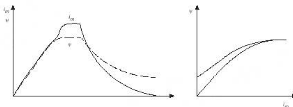
Рисунок 2B.11 — Диаграмма потоков и токов насыщения
