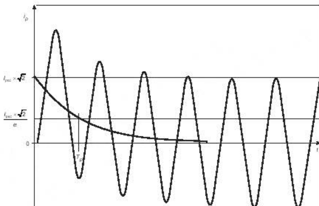
Рисунок 202 — Первичная постоянная времени T_p
