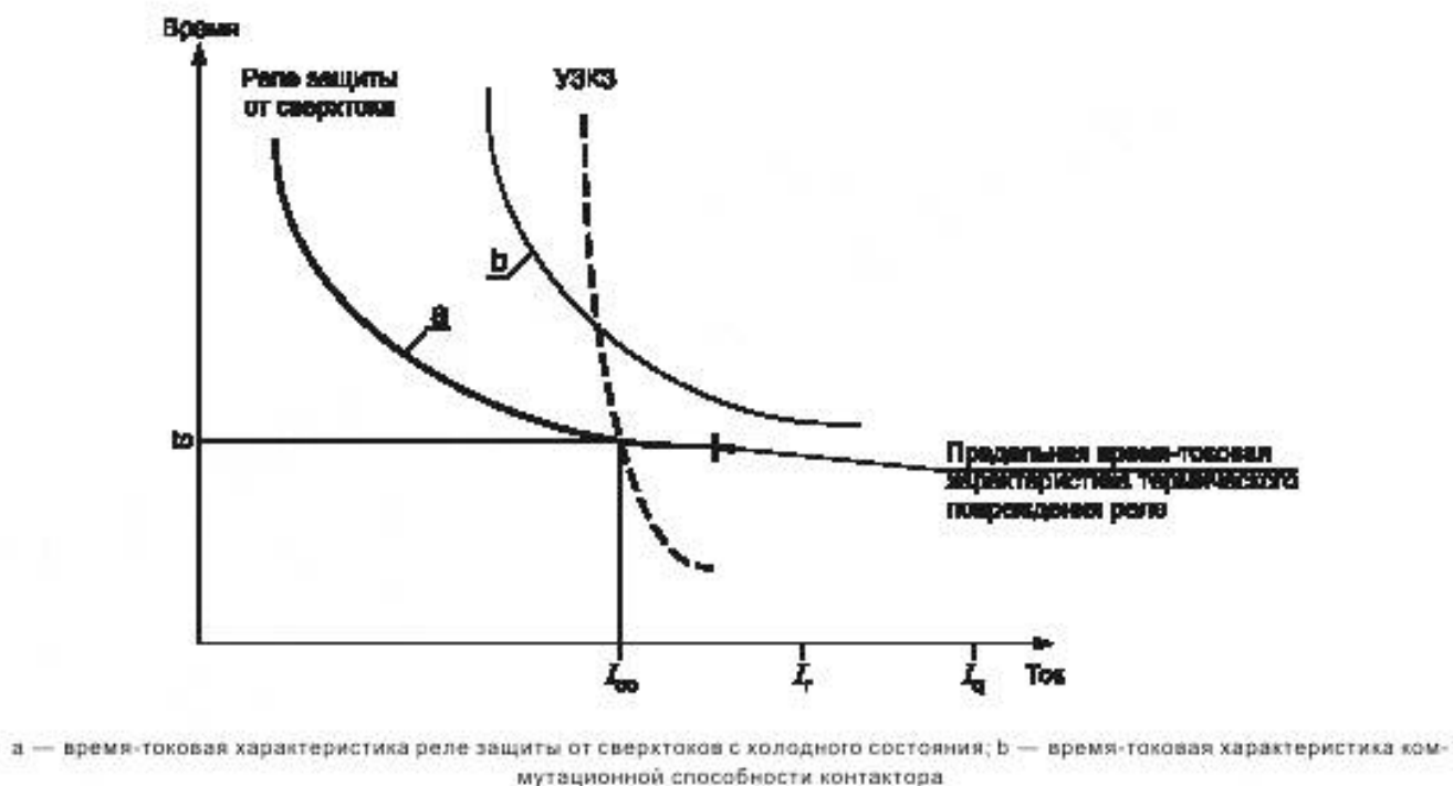
Рисунок 5а — Координация пускателя с предохранителем
