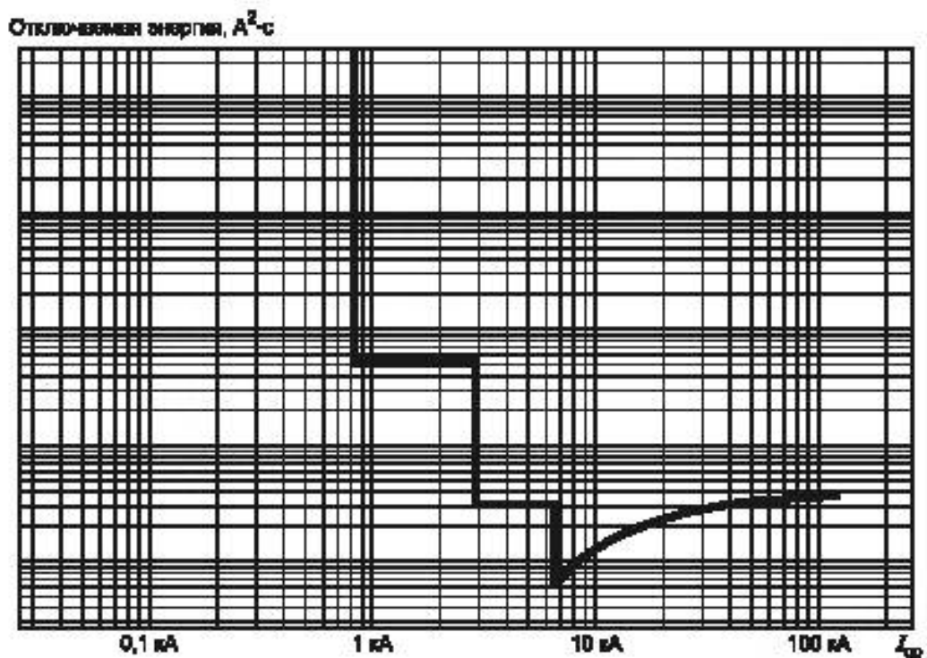
Рисунок 2 — Пример характеристики интеграла Джоуля ( I^2t ) автоматического выключателя
