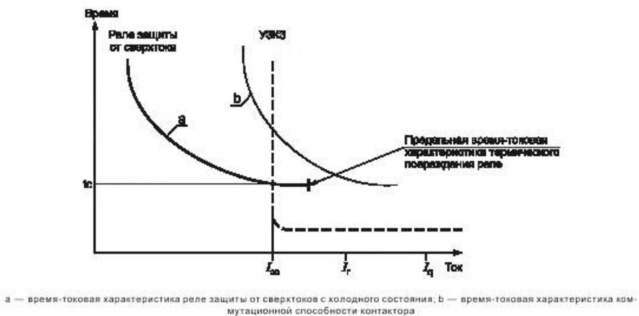
Рисунок 5б — Координация пускателя с автоматическим выключателем
