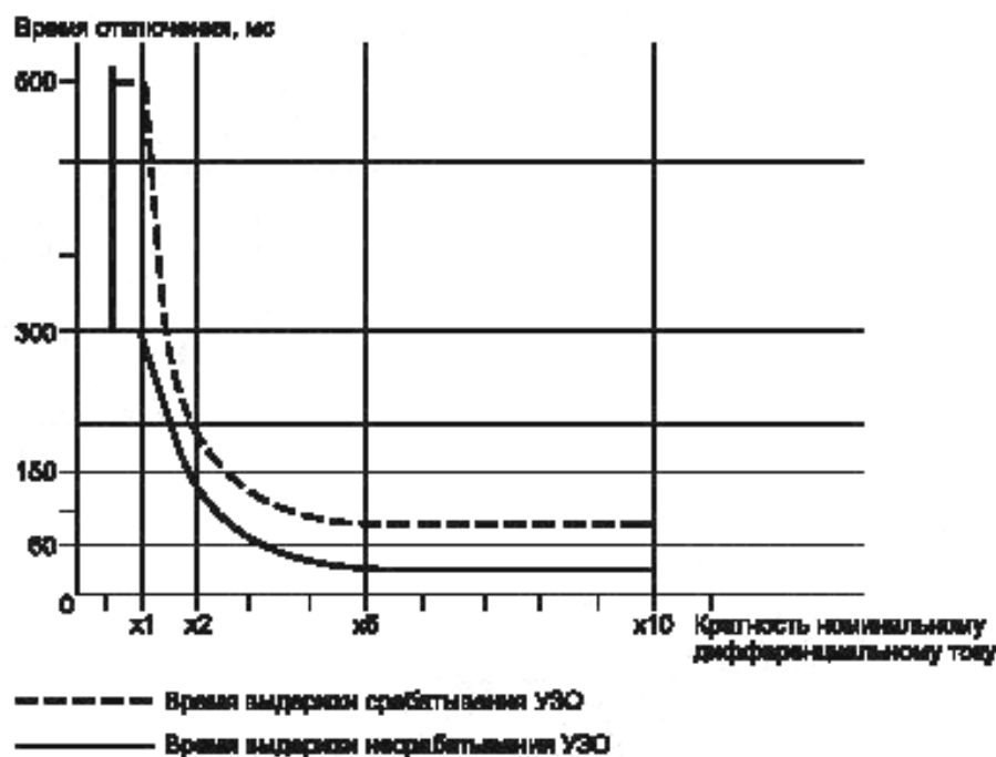
Рисунок 9 — Характеристики УЗО, представляющие селективность при утечке, — характеристика времени выдержки срабатывания типа S
