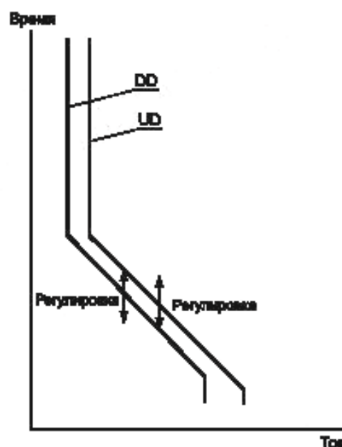
Рисунок 1б — Сравнение время-токовых характеристик электронных расцепителей в зоне сверхтоков
