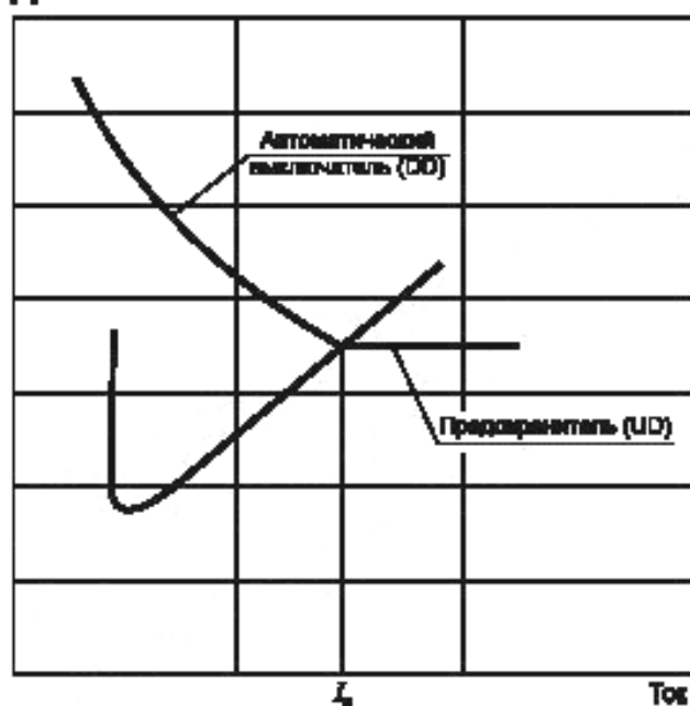
Рисунок 7 — Проверка селективности между предохранителем и автоматическим выключателем для времени срабатывания t < 0,1 с
