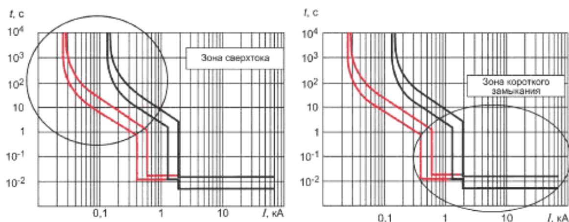
Рисунок В.1 — Зоны сверхтоков и короткого замыкания
