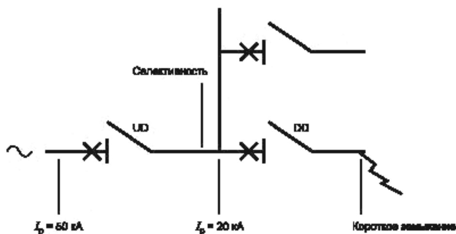
Рисунок А.4 — Пример координации автоматических выключателей с максимальным уровнем тока короткого замыкания 50 кА и уровнем тока повреждения 20 кА
