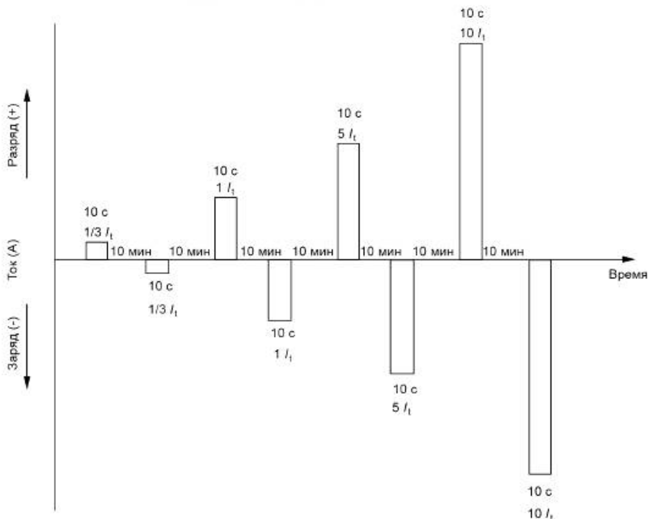
Рисунок А.3 — Порядок получения вольт-амперной характеристики (пример с испытуемыми аккумуляторами с нормированной емкостью менее 20 А·ч)
