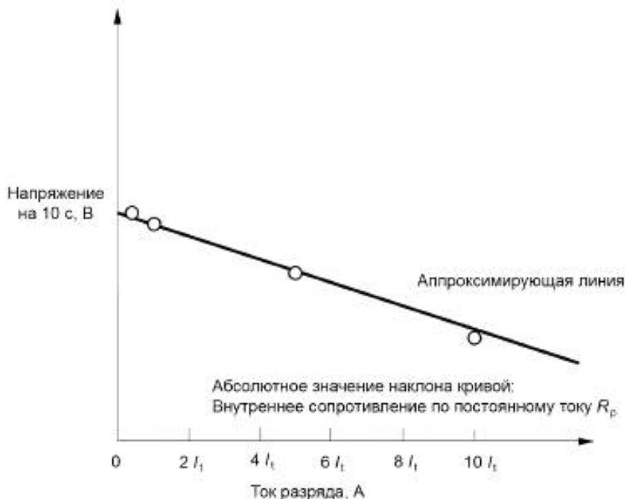
Рисунок А.6 — Метод получения значения внутреннего сопротивления по постоянному току при разряде
