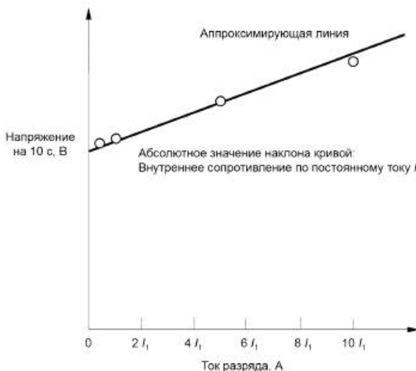
Рисунок А.7 — Метод получения значения внутреннего сопротивления по постоянному току при заряде
