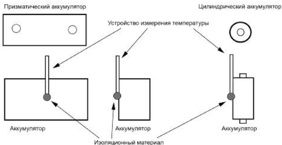
Рисунок А.1 — Пример измерения температуры аккумулятора
