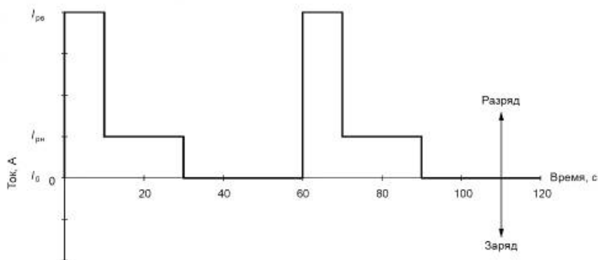
Рисунок 1 — Профиль испытания без рекуперации
