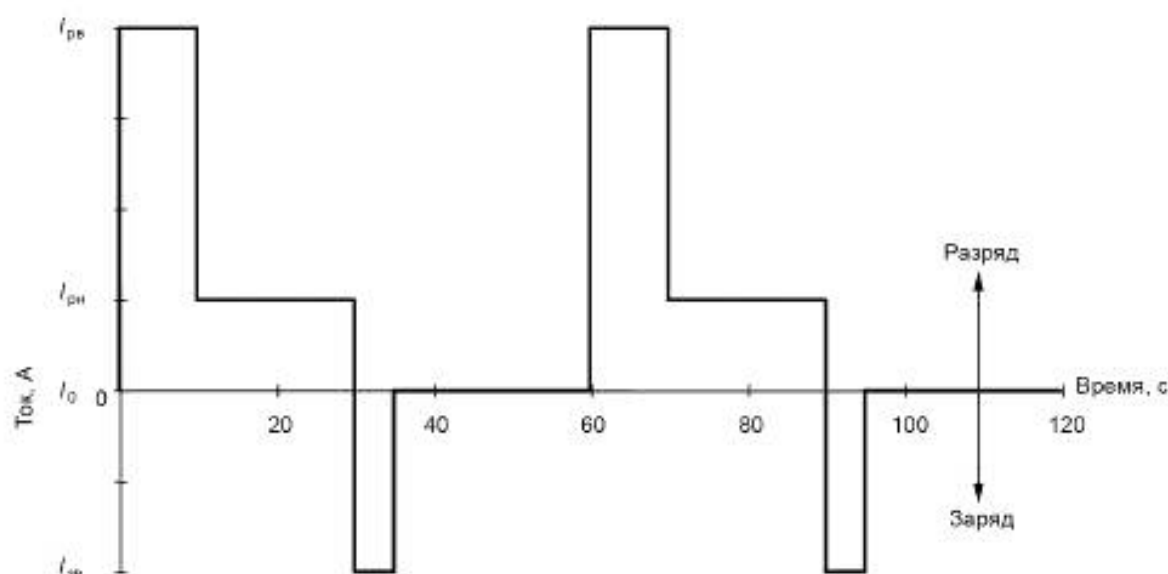
Динамический режим разряда с рекуперацией
