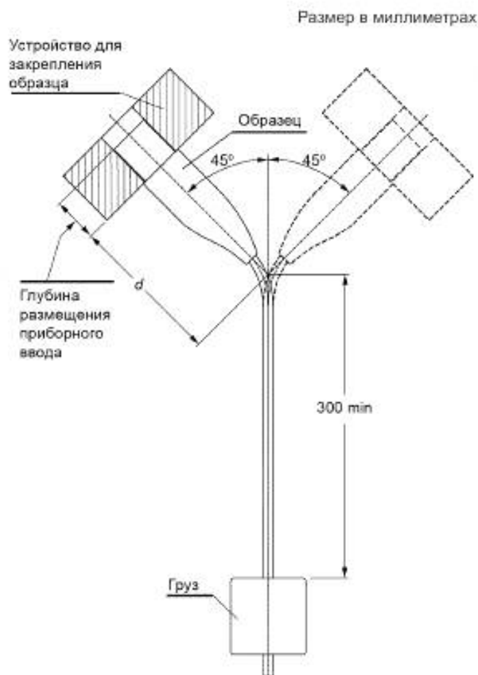
Рисунок 2 — Устройство для испытания на изгиб
