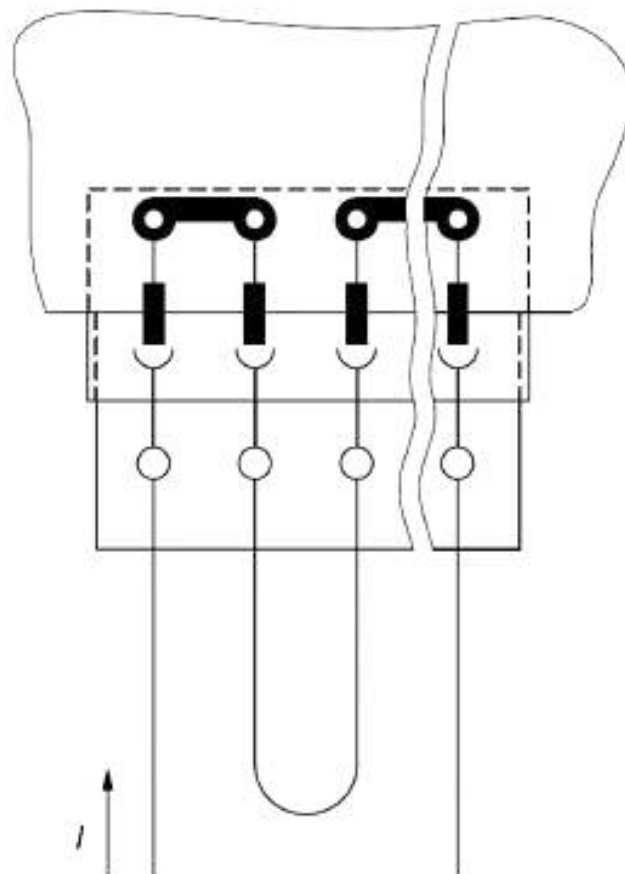
Рисунок 1b — Схема подключения двух частей соединителя на печатной плате для испытания на превышение температуры
