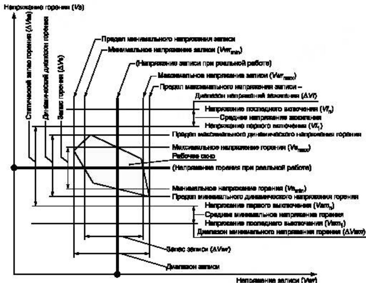
Рисунок А.6 — Взаимосвязь между запасами и подаваемыми напряжениями
