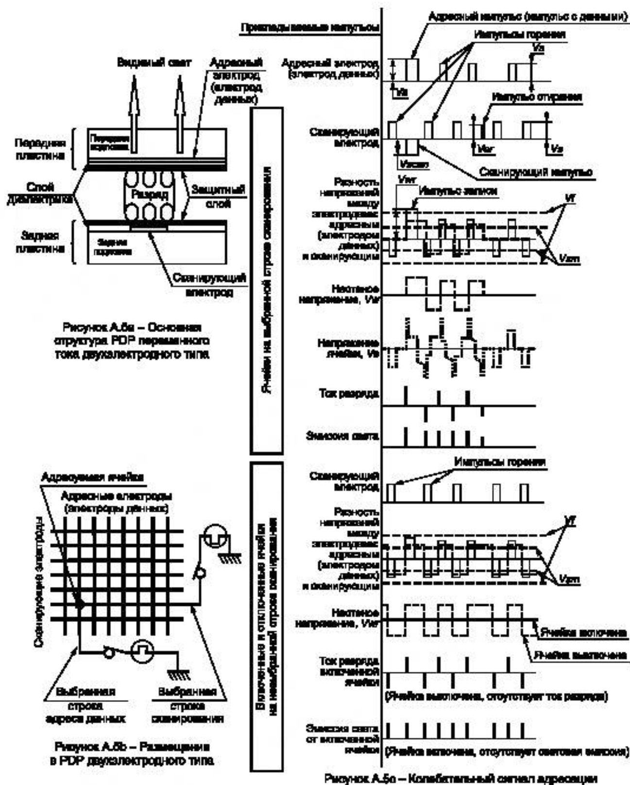
Рисунок А.5 — Работа АС PDP двухэлектродного типа
