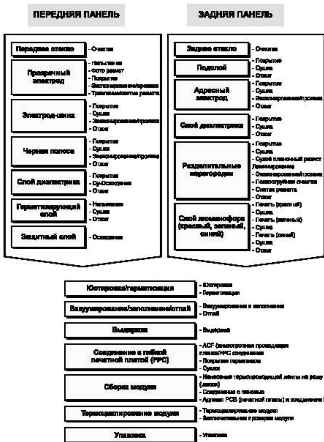
Рисунок D.1 — Алгоритм производства (изготовления) PDP
