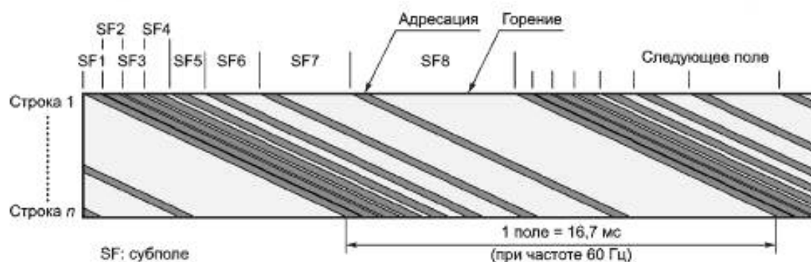
Рисунок А.10 Метод адресации при отображении (AWD)
