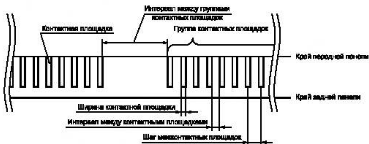
Рисунок Е.2 — Размеры контактных площадок
