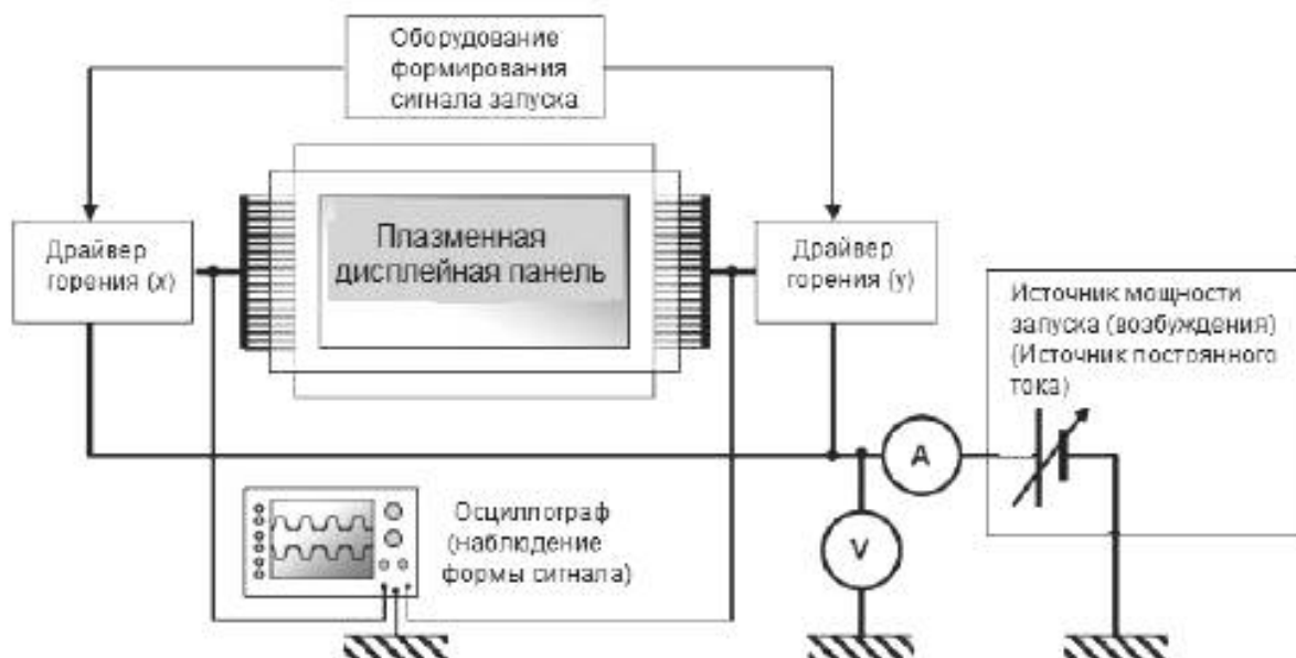
Рисунок 8 – Схема системы измерения мощности запуска (горения)
