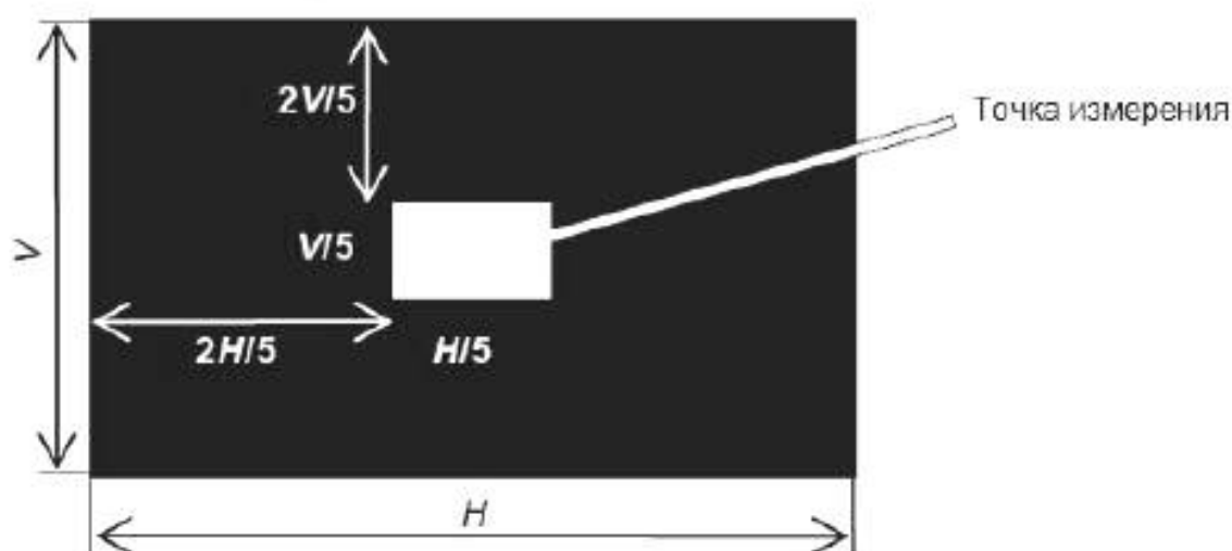
Рисунок 3 – Схема измерения яркости 4 %-ного окна
