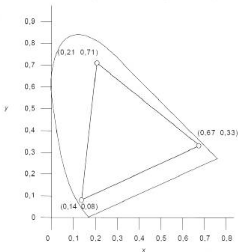
Рисунок 6 — Пример измерения цветовой гаммы
