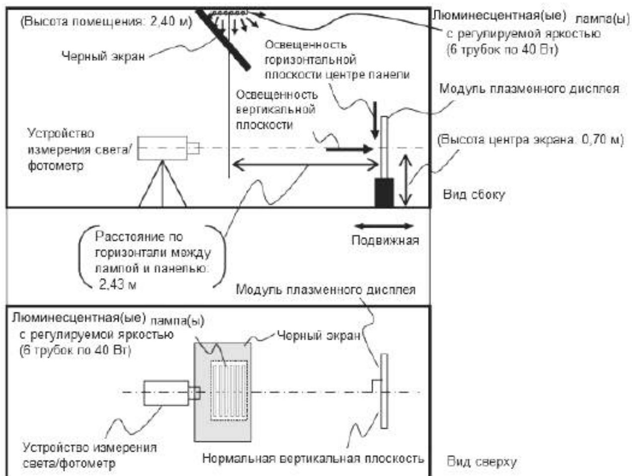
Рисунок 2 — Пример условий освещенного помещения
