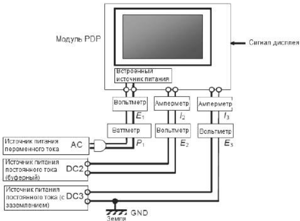
Рисунок 7 – Пример схемы измерения мощности и тока
