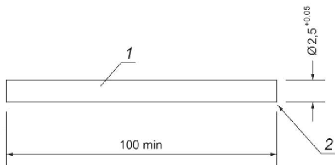
1 — испытательный стержень (металлический); 2 — прямоугольные острые края
