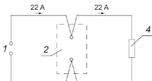
Рисунок 3б — Схема цепи для испытания 2
