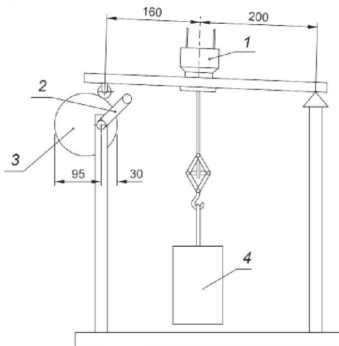
1 — образец; 2 — кривошип; 3 — эксцентрик; 4 — груз
