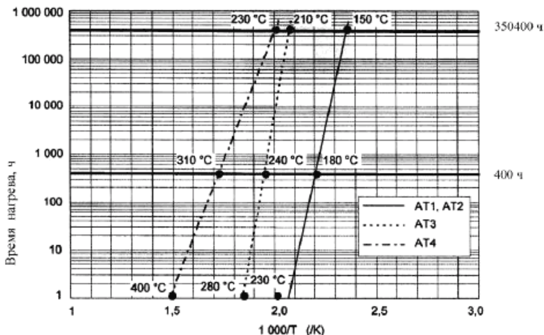
Рисунок А.1 — График Аррениуса (остаточное напряжение 90 %)
