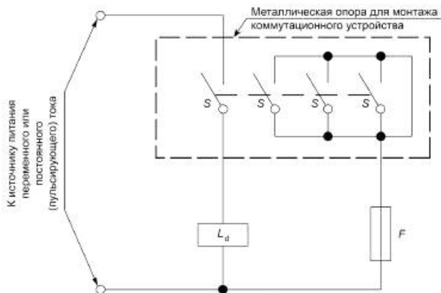
Рисунок 2б — Контактные элементы противоположной полярности, электрически разделенные
