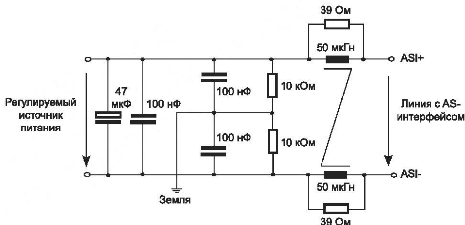
Рисунок 79 — Схема развязки испытательной схемы
