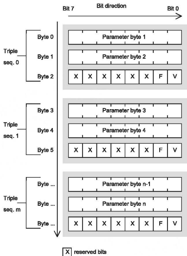
Рисунок А.5 — Структура данных строки параметров (S-7.4)
