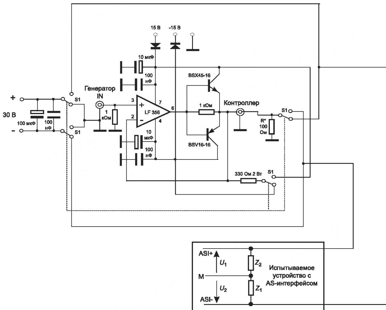
Рисунок 100 — Подключение мастера для измерения симметрии
