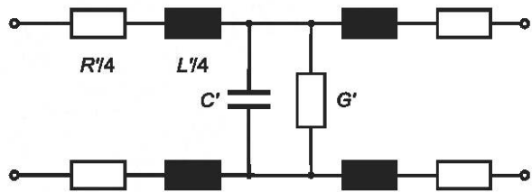
Рисунок 6 — Модель среды передачи AS-i
