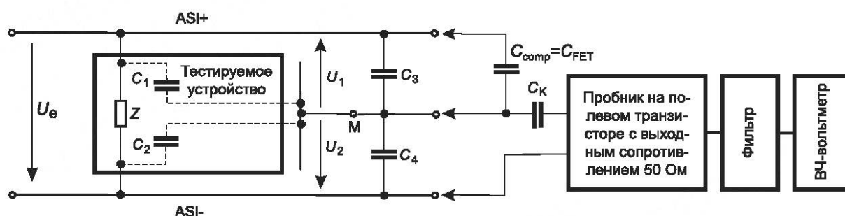
Рисунок 101 — Схема измерения симметрии ведущего устройства ASI-i
