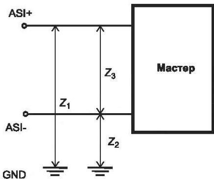
Рисунок 56 — Импедансы мастера
