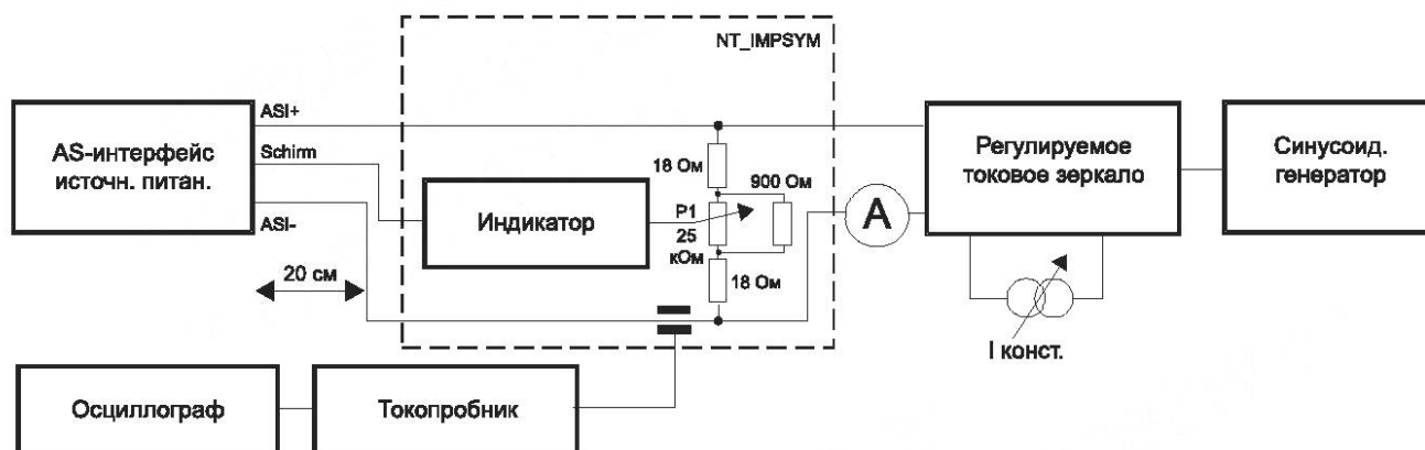
Рисунок 64 — Испытательная установка для измерения симметрии
