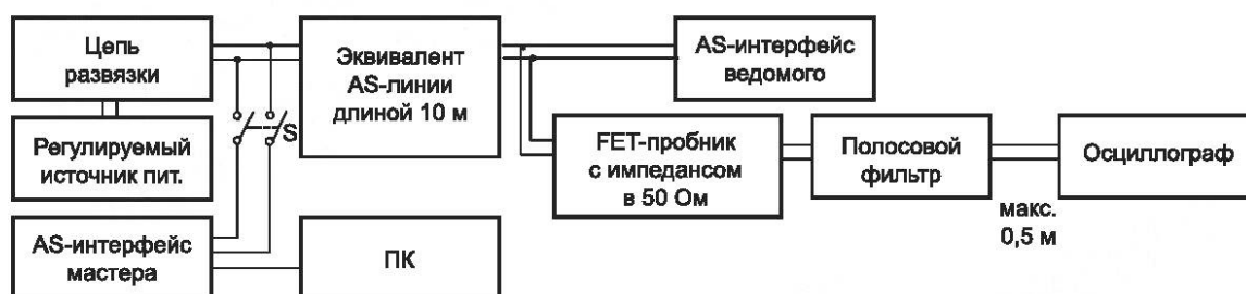
Рисунок 80 — Схема испытаний
