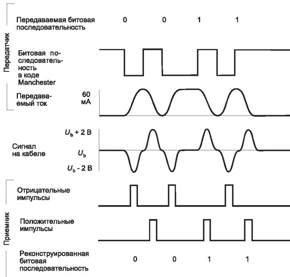
Рисунок 2 — Кодирование передачи
