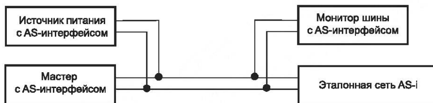
Рисунок 111 — Схема испытаний
