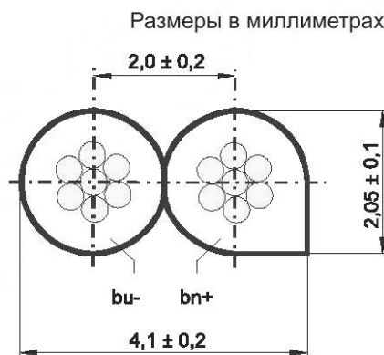
Рисунок 47 — Кабель шкафа AS-i
