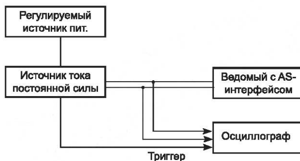
Рисунок 84 — Испытательная схема
