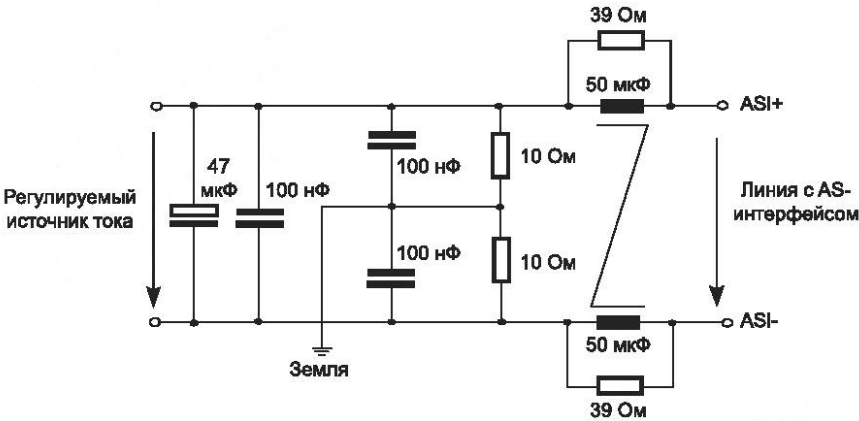
Рисунок 96 — Схема развязки
