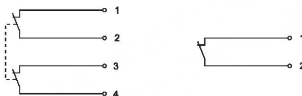
Рисунок A.7 — Подключение механических переключателей
