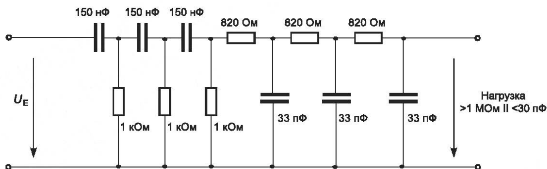
Рисунок 67 — Фильтр В (полосовой фильтр от 10 до 500 кГц)
