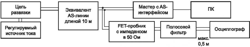
Рисунок 95 — Излучение шума тестовой схемы AS-i мастер
