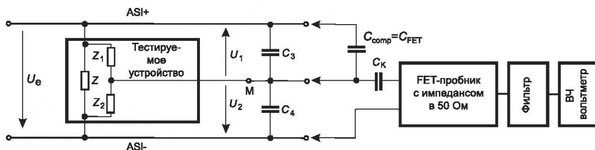
Рисунок 88 — Схема испытаний (часть 1)
