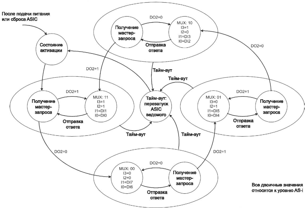
б) Диаграмма состояний ведомого для комбинированной транзакции типа 3 (8I/8O)
