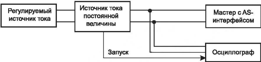
Рисунок 106 — Блок-схема измерения тока, потребляемого AS-i-мастером
