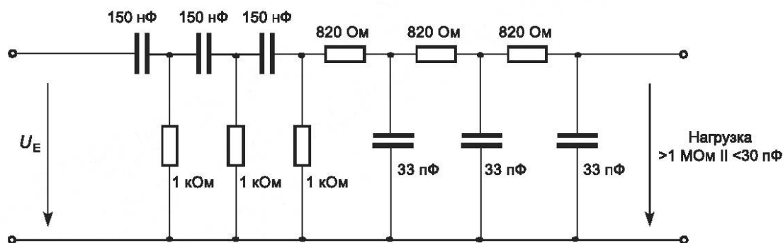
Рисунок 73 — Полосовой фильтр (10 ... 500 кГц)
