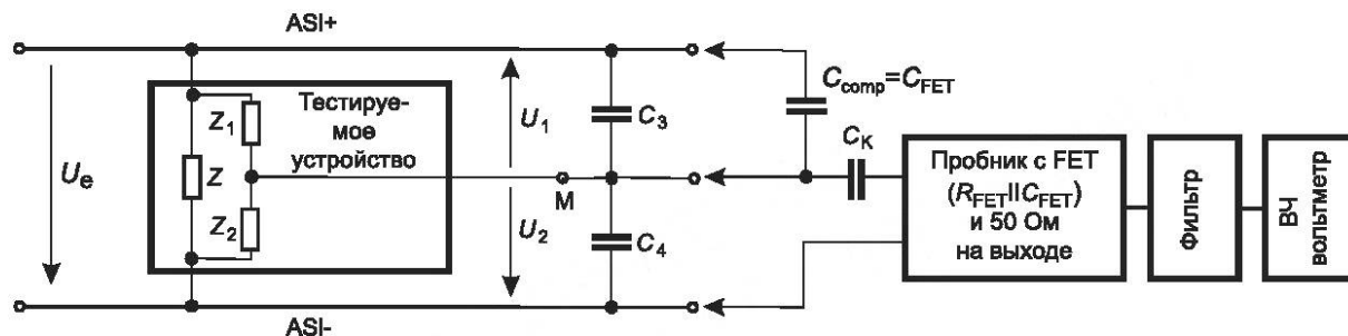
Рисунок 71 — Схема испытаний (часть 1)
