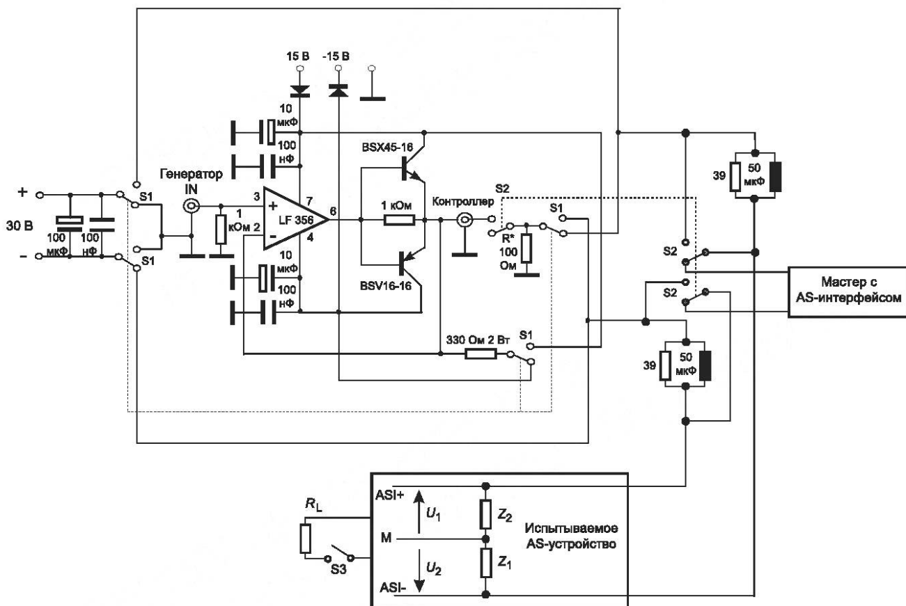
Рисунок 87 — Схема испытаний
