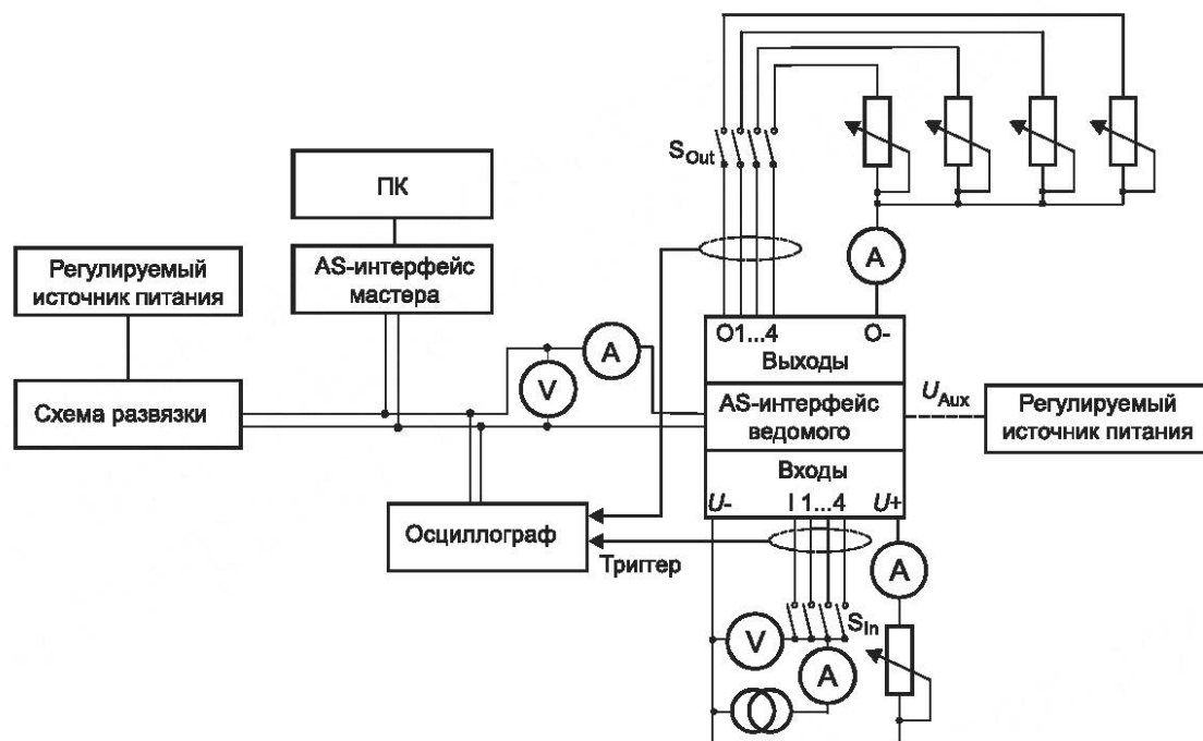
Рисунок 78 — Испытательная схема
