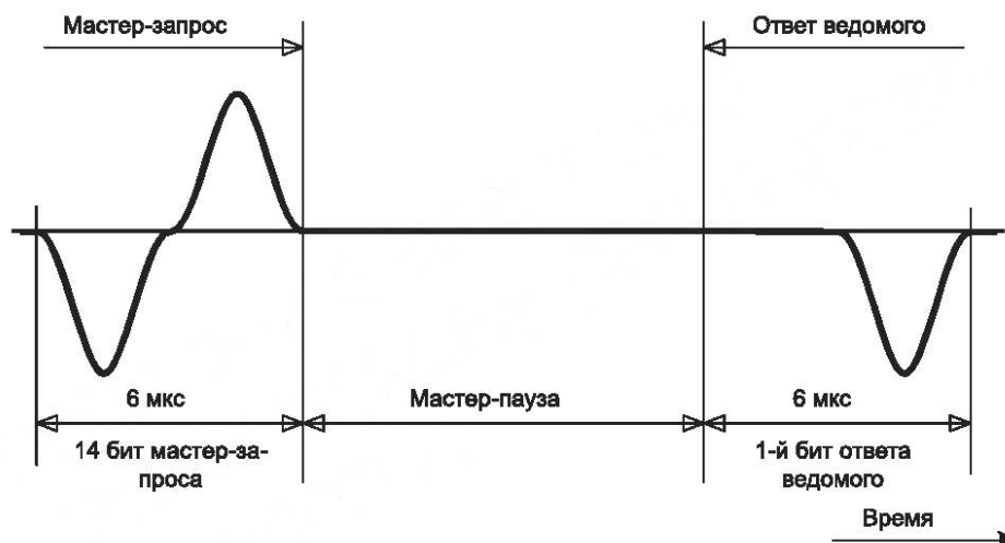
Рисунок 9 — Схема мастер-паузы
