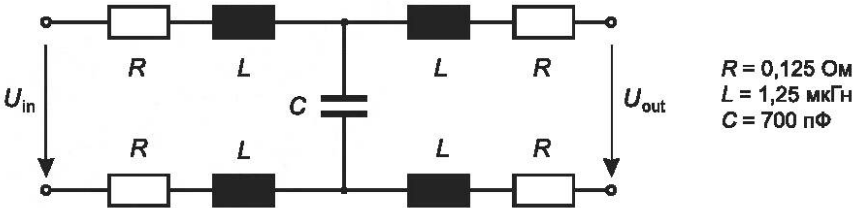
Рисунок 98 — Эквивалентная схема 10-метровой линии AS-i
