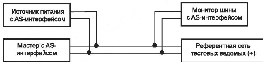
Рисунок 110 — Схема испытаний для проверки функционирования в нормальном режиме
