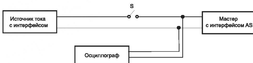
Рисунок 104 — Схема испытаний задержки включения
