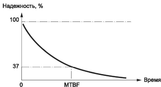
Рисунок К.1 — График зависимости надежности, %, от времени
