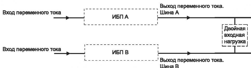
Рисунок A.6 — ИБП с двумя шинами
