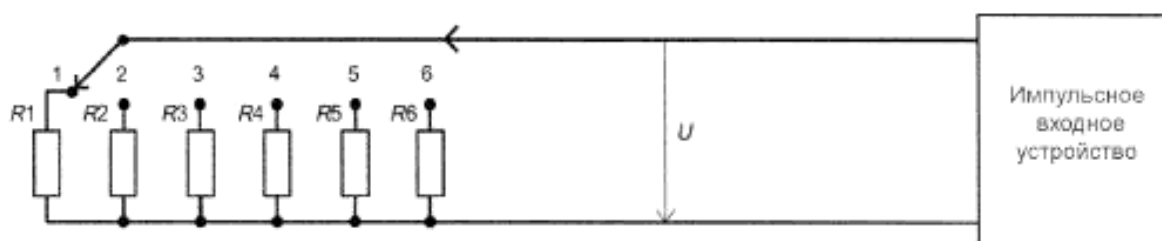
Рисунок E.3 – Испытательная схема импульсного входного устройства
