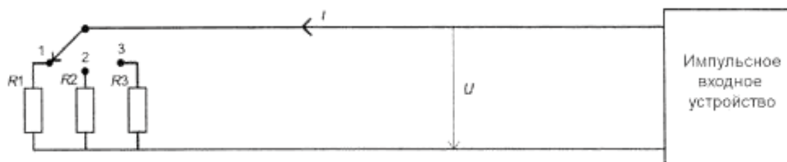
Рисунок D.1 – Испытательная схема импульсного входного устройства
