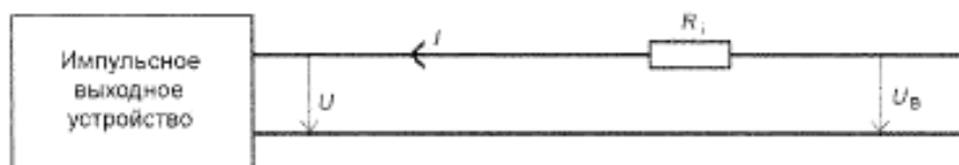
Рисунок С.1 – Испытательная схема импульсного выходного устройства
