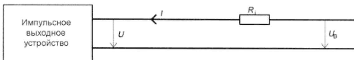
Рисунок E.2 – Испытательная схема импульсного выходного устройства
