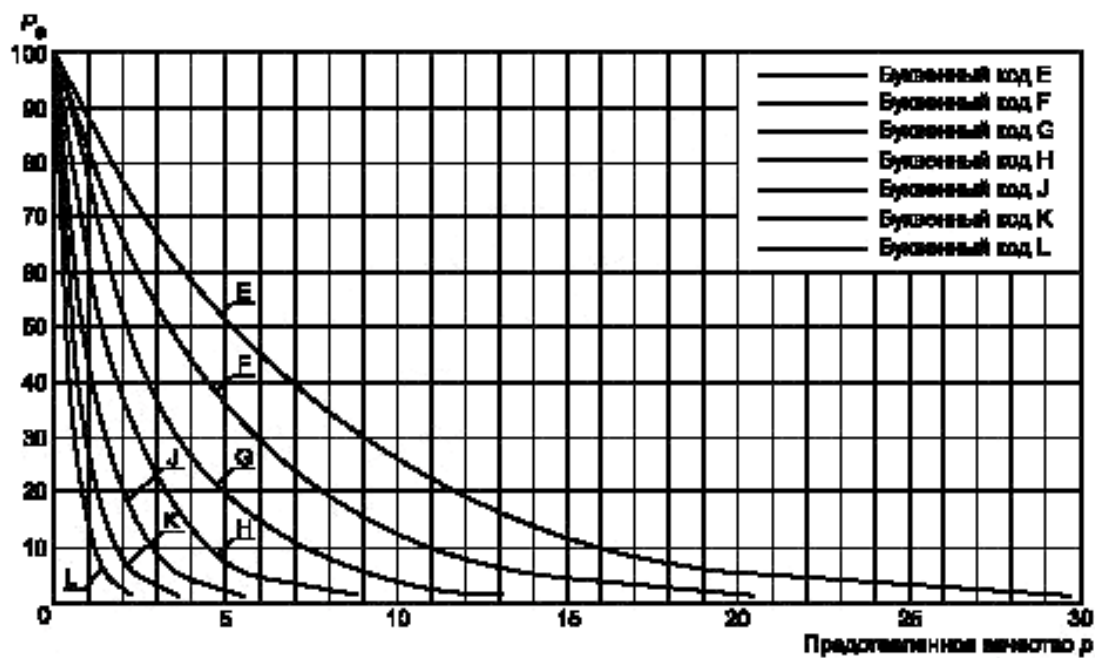
Рисунок 5 — Кривые ОС (PX) для планов однократного выборочного контроля, A_s=0
