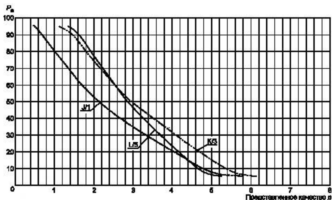
Рисунок 6 — Кривые рабочих характеристик ОС (РХ) для планов однократного выборочного контроля на некритичные несоответствия, процедура В
