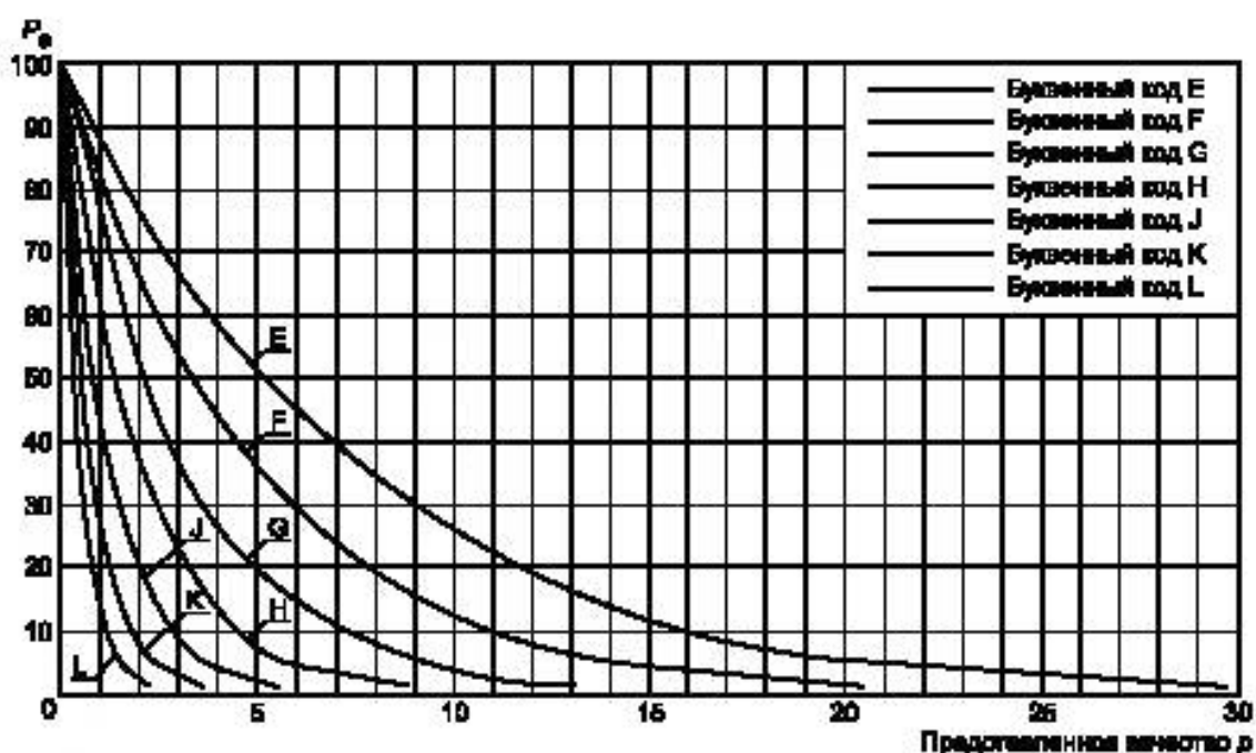
Рисунок 5 — Кривые ОС (PX) для планов однократного выборочного контроля, A_{sc}=0
