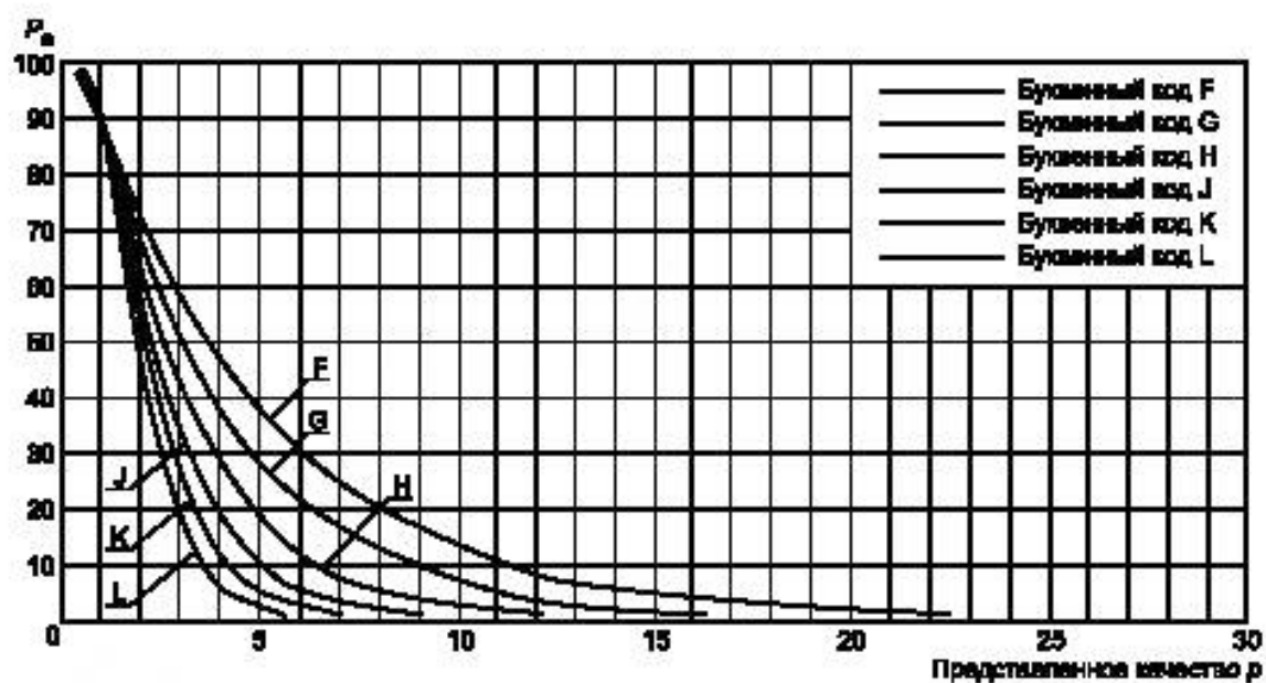
Рисунок 8 — Кривые ОС (PX) для ужесточенного контроля, AQL (ППК) = 1,0
