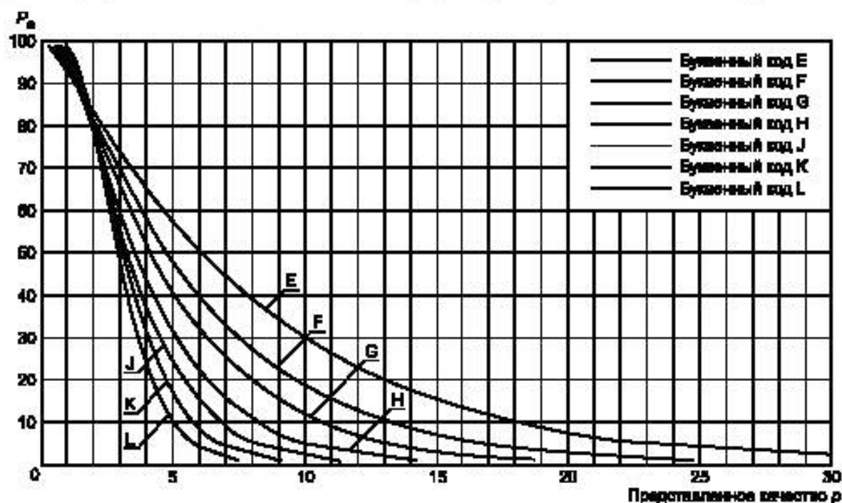
Рисунок 7 — Кривые ОС (РХ) для нормального контроля, AQL (ППК) = 1,0
