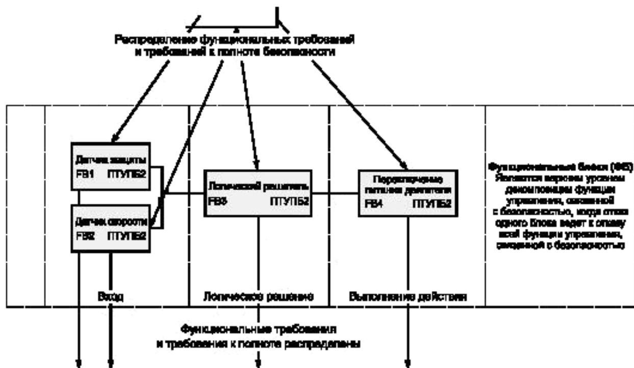
Рисунок В.5 — Начальная концепция архитектуры СБФУ
