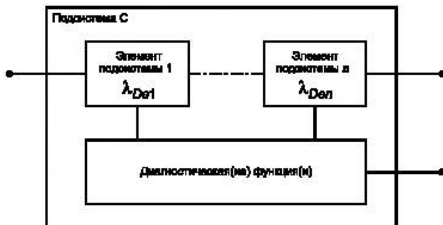
Рисунок 8 — Логическое представление подсистемы типа С
