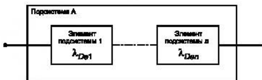
Рисунок 6 — Логическое представление подсистемы типа А
