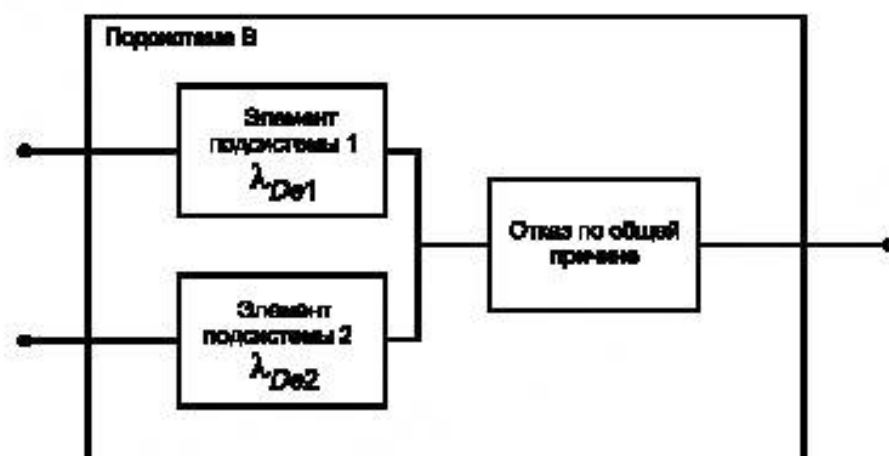
Рисунок 7 — Логическое представление подсистемы типа В
