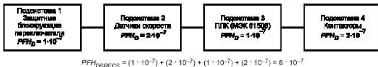
Рисунок В.8 — Оценка PFH_D для СБЗСУ
