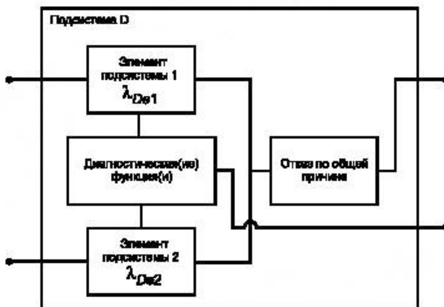
Рисунок 9 — Логическое представление подсистемы типа D
