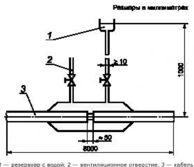
Рисунок Е.1 — Схема устройства для испытания на водонепроницаемость
