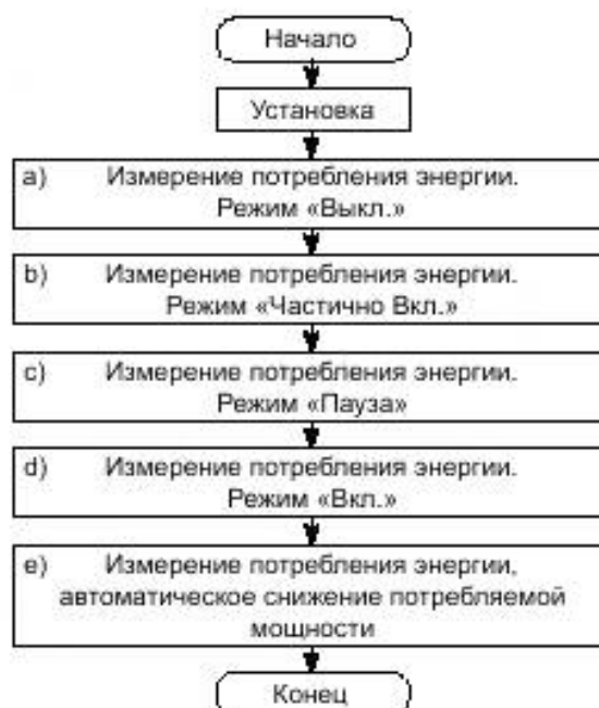
Рисунок 1 — Последовательность измерений
