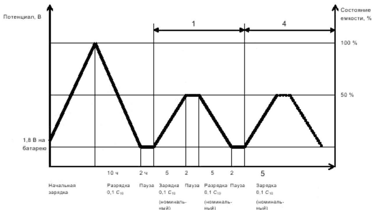
Рисунок 2 — Циклические условия эффективности метода испытаний
