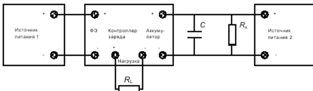
Рисунок 3 — Схема проверки без подключения измерительных приборов
