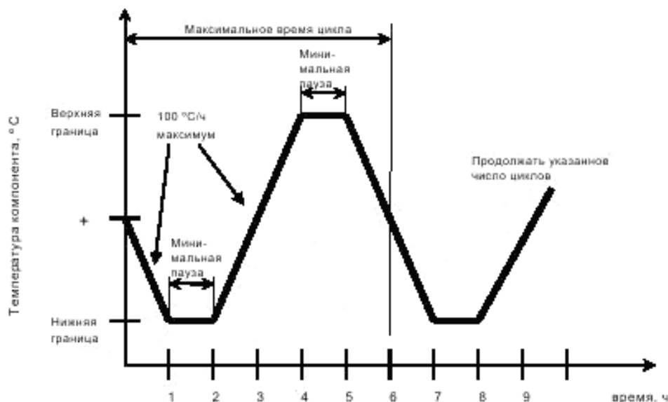
Рисунок 4 — Термоциклирование
