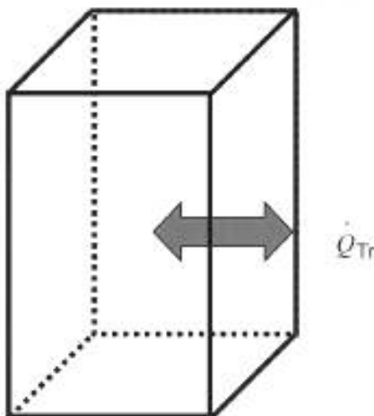
Рисунок 4 — Теплопередача через стенки корпуса
