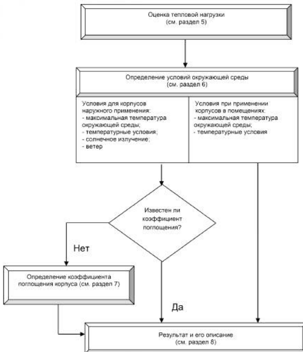
Рисунок 2 — Технологическая схема для определения коэффициента поглощения
