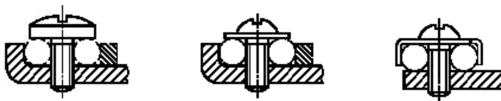
Рисунок 9b и 9с — Винтовые выводы
