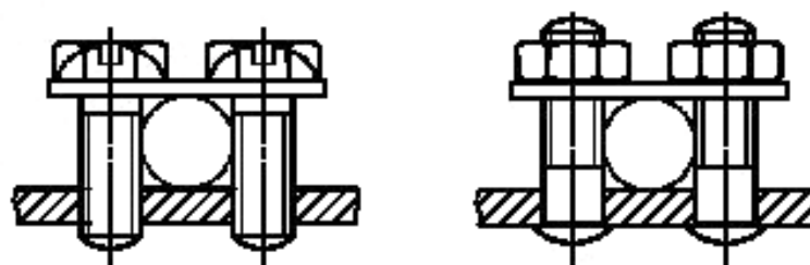
Рисунок 9е — Пластина́тые выводы
