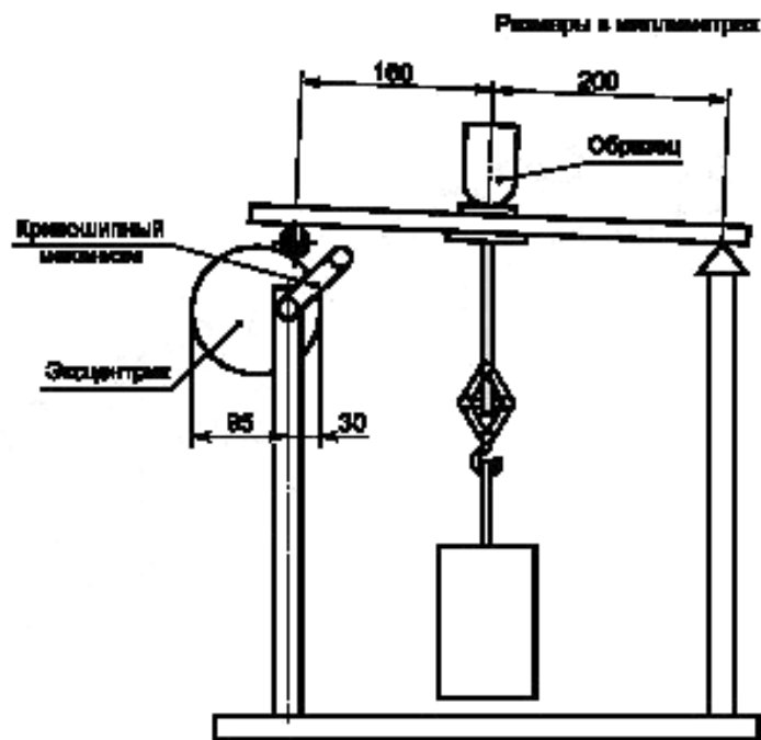
Рисунок 4 — Установка для испытания кабельного крепления
