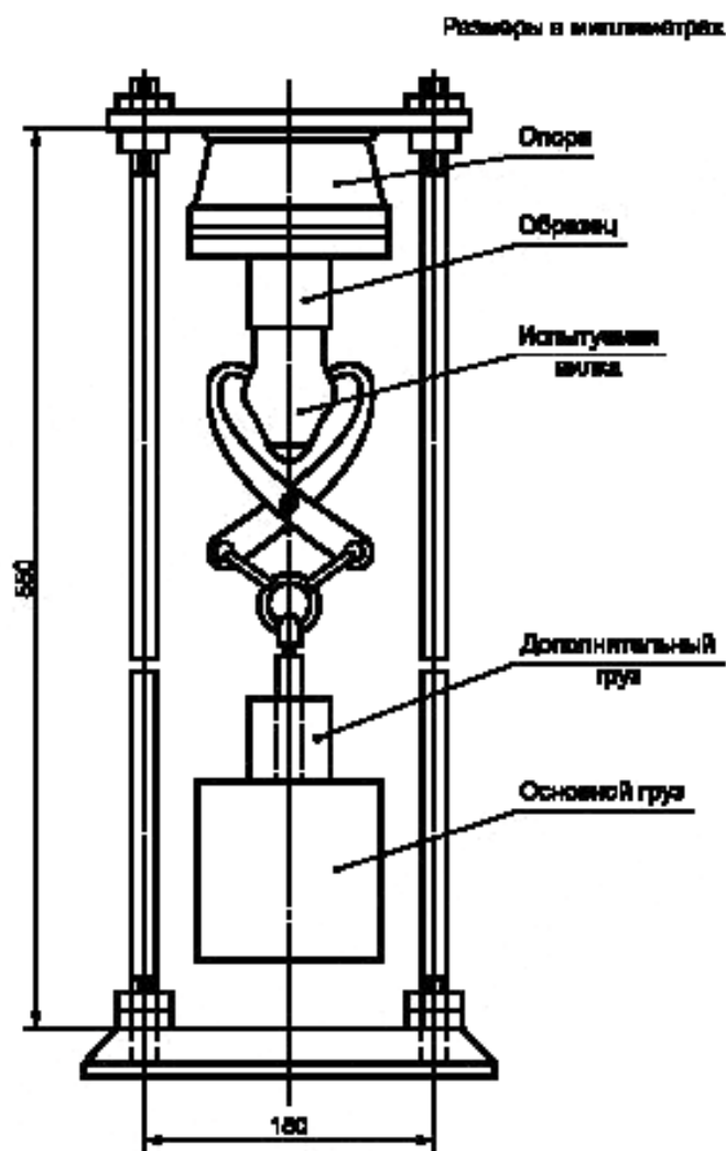
Рисунок 16 — Устройство для проверки расщепляющего усилия
