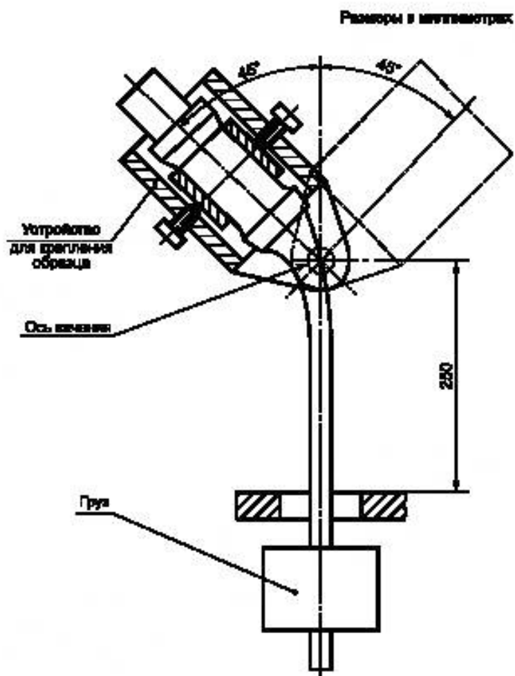
Рисунок 7 — Установка для испытания на изгиб
