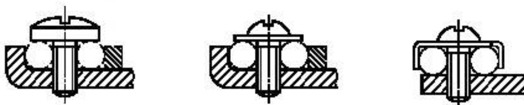
Рисунок 9b и 9c — Винтовые выводы
