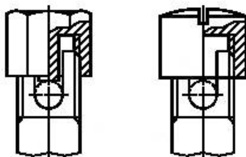
Рисунок 9g — Закрытые резьбовые выводы с прижимной гайкой
