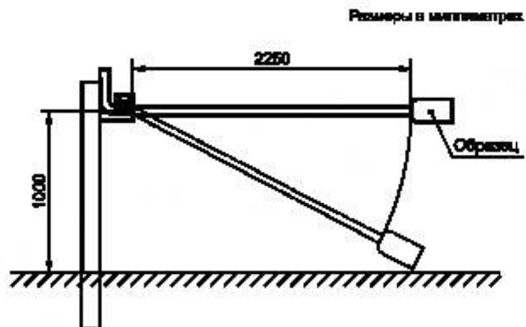
Рисунок 6 — Устройство для испытания на механическую прочность вилки и переносных розеток
