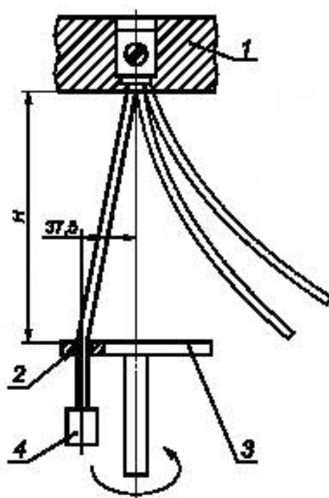
1 — панель; 2 — гильза; 3 — диск; 4 — груз
