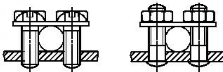
Рисунок 9e — Пластиначные выводы
