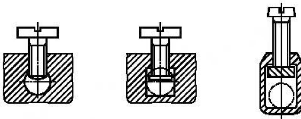
Рисунок 9a — Столбчатые выводы
