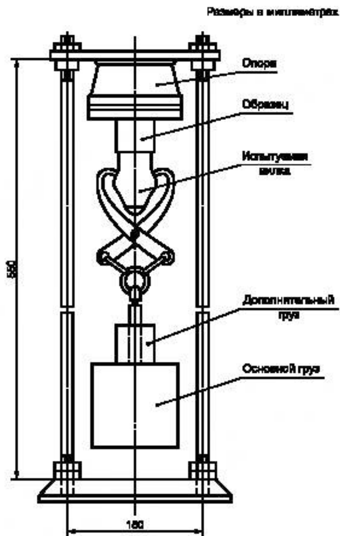
Рисунок 16 — Устройство для проверки расчленяющего усилия
