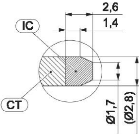
Деталь F(PE) с IC
