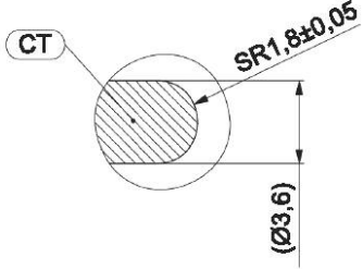
Деталь D(L1, L2/N) дополнительная форма
