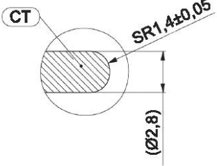
Деталь F(PE) дополнительная форма
