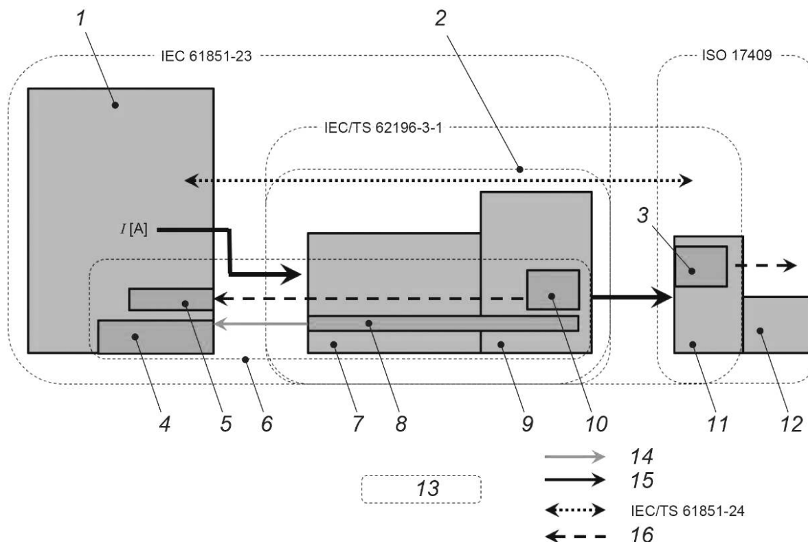
Рисунок 102 — Оборудование для питания постоянного тока электромобиля с измерением температуры, теплопередачей и теплообменом
