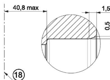
Деталь R
