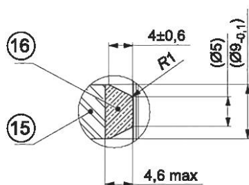
Деталь N
