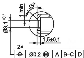
Деталь G (2:1)
