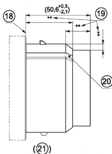
Деталь Q
