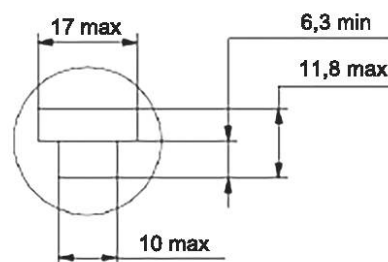
Деталь Z
