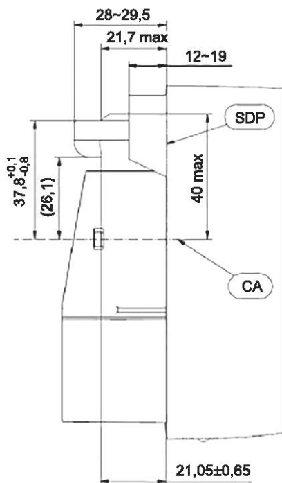
Деталь Y
