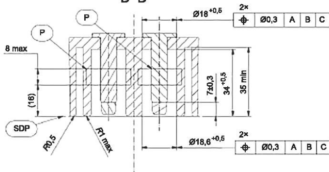
D-D
