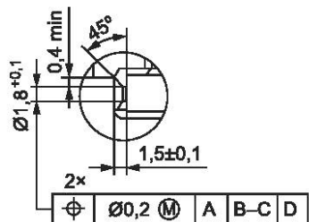
Деталь F (2:1)
