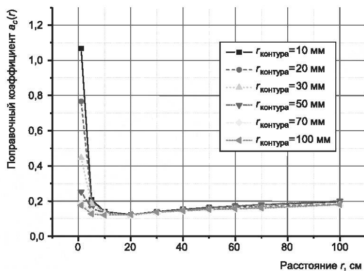
Рисунок С.5 — Поправочный коэффициент a_c(r_1) для полей с удельной электропроводностью 0,1 См/м и датчиком площадью A_{\text{датчика}} = 100 \text{ см}^2 для модели тела человека (применяются шкалы значений пределов согласно ICNIRP [11])
