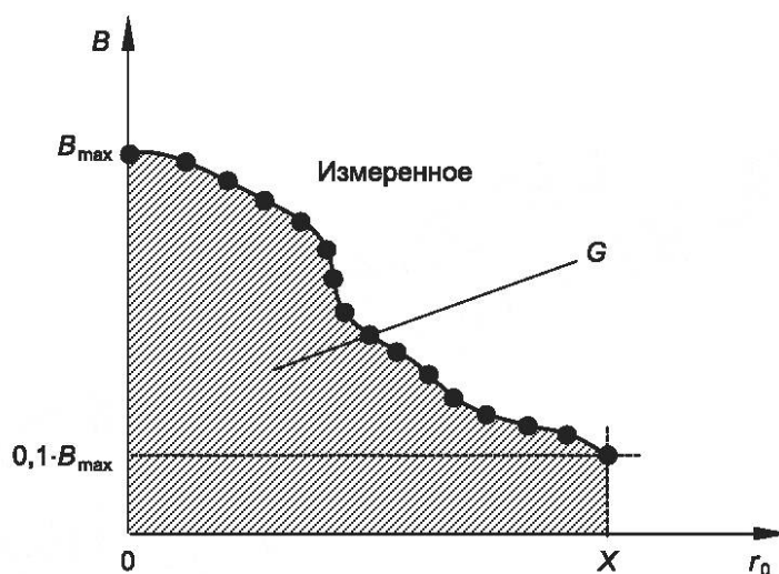
Рисунок С.2 — Градиент плотности магнитной индукции
