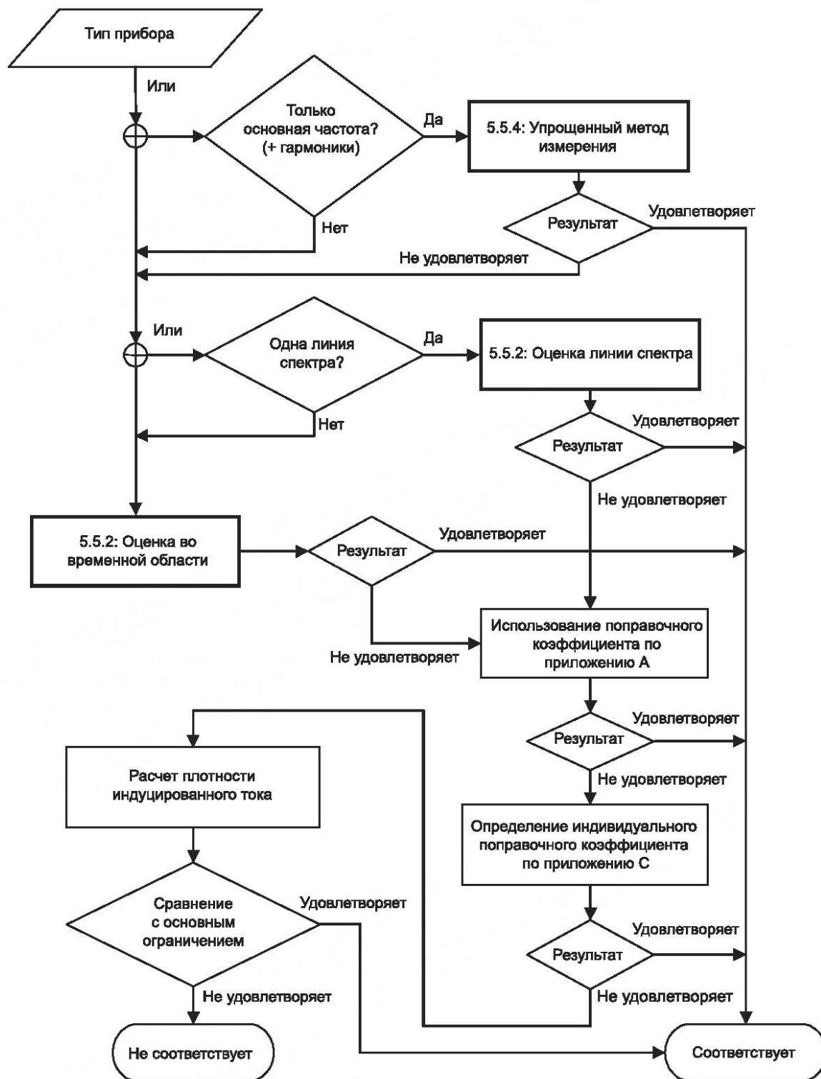
Рисунок 1 — Рекомендации по выбору метода испытания начиная с оценки контрольных уровней
