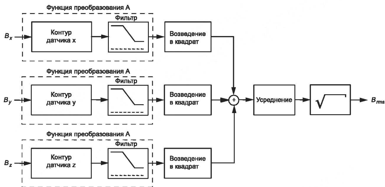
Рисунок Z2 — Блок-схема эталонного метода
