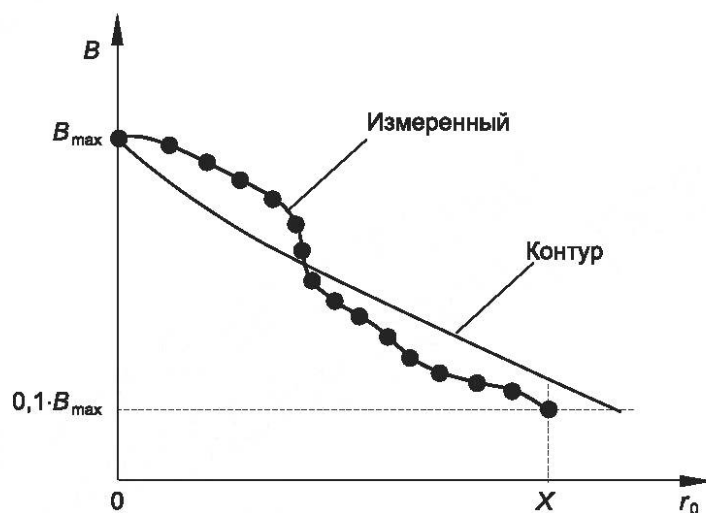
Рисунок С.4 — Градиент измеренной магнитной индукции и магнитной индукции, создаваемой контуром с током
