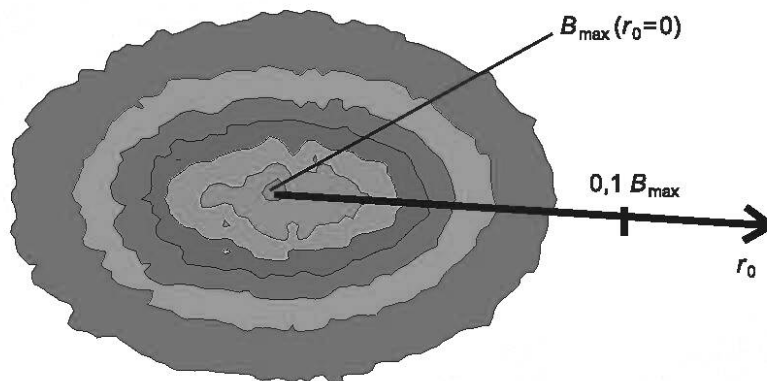
Рисунок С.1 — Точка максимальной интенсивности поля
