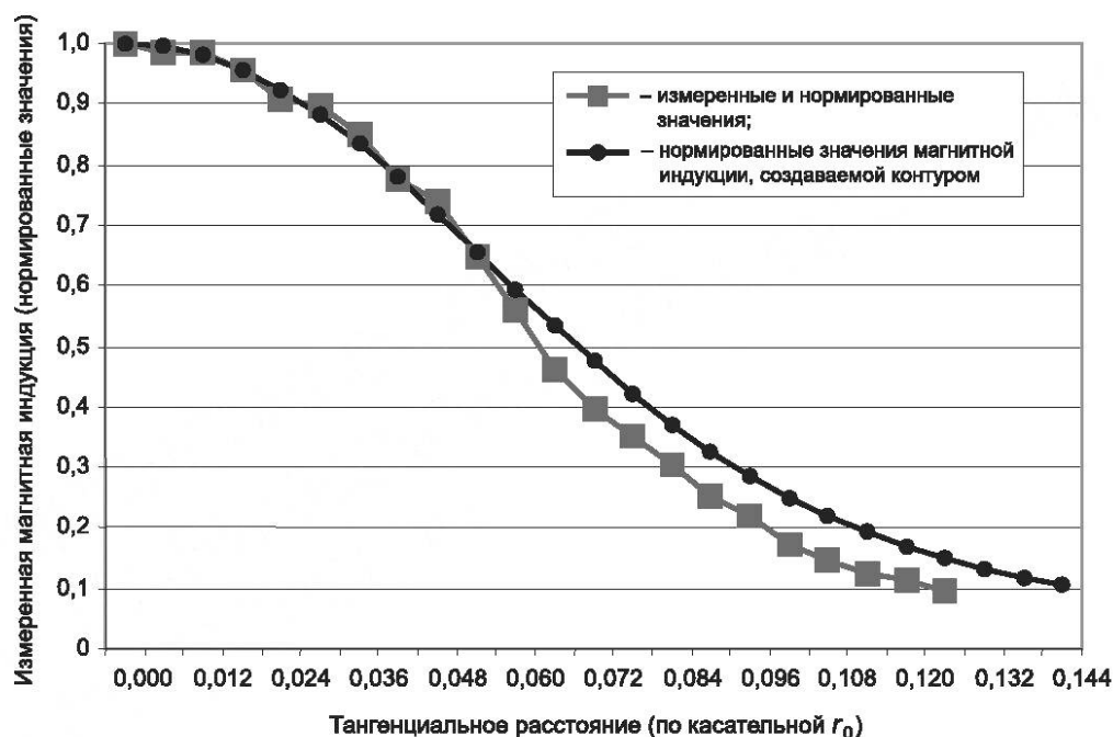
Рисунок D.2 — Нормированное распределение поля вдоль расстояния r_0 по касательной
