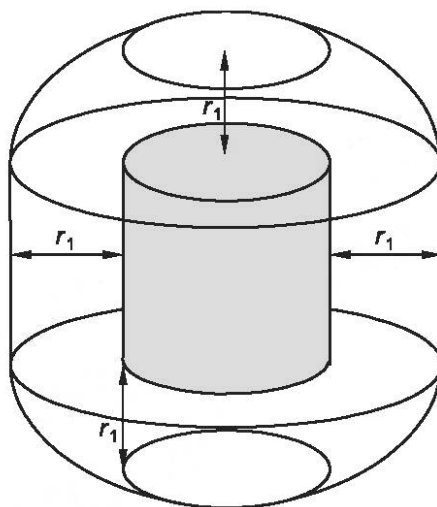
Рисунок А.2 — Измерительное положение вокруг (см. 3.2.7)
