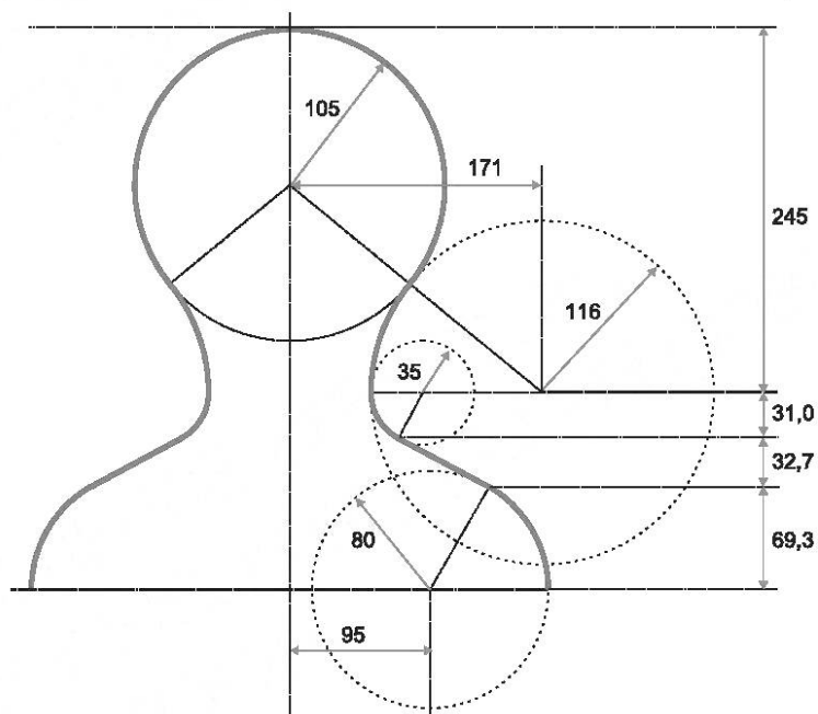
Рисунок D.4 — Деталировочный чертеж модели головы и плеч
