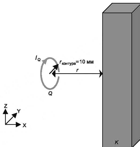
Рисунок D.5 — Схема размещения источника Q по отношению к модели K
