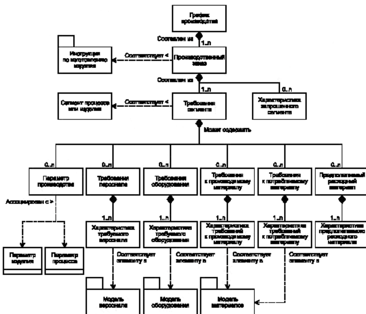
Рисунок 9 — Модель производственного графика
