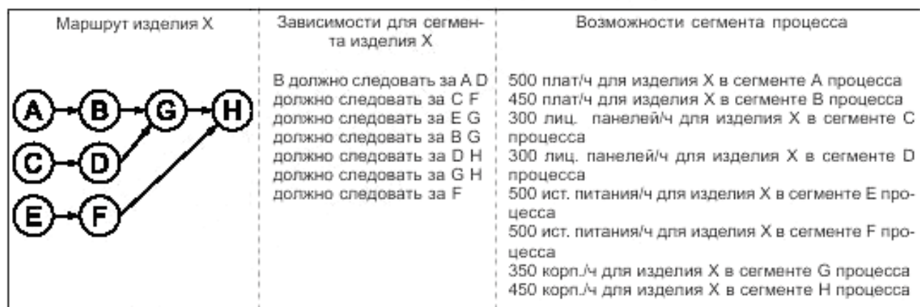
Рисунок С.3 — Технологический маршрут изделия
