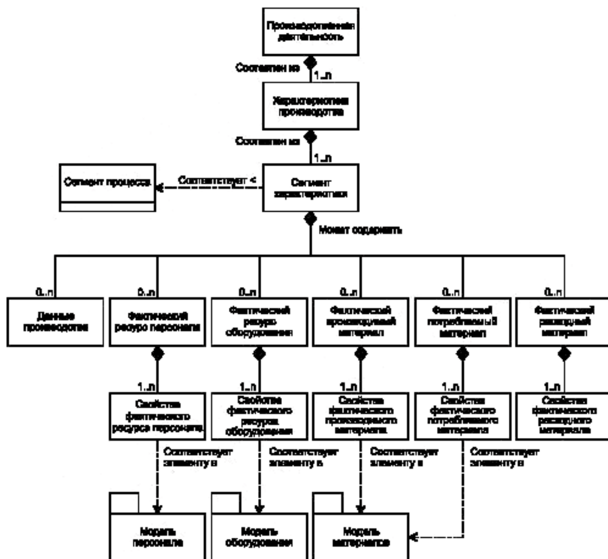
Рисунок 10 — Модель функционирования производства
