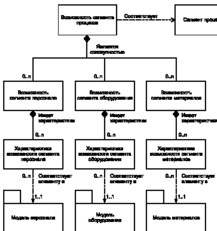
Рисунок 7 — Модель производственных возможностей сегмента процесса
