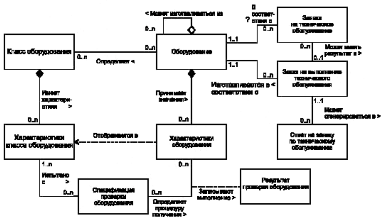
Рисунок 3 — Модель оборудования
