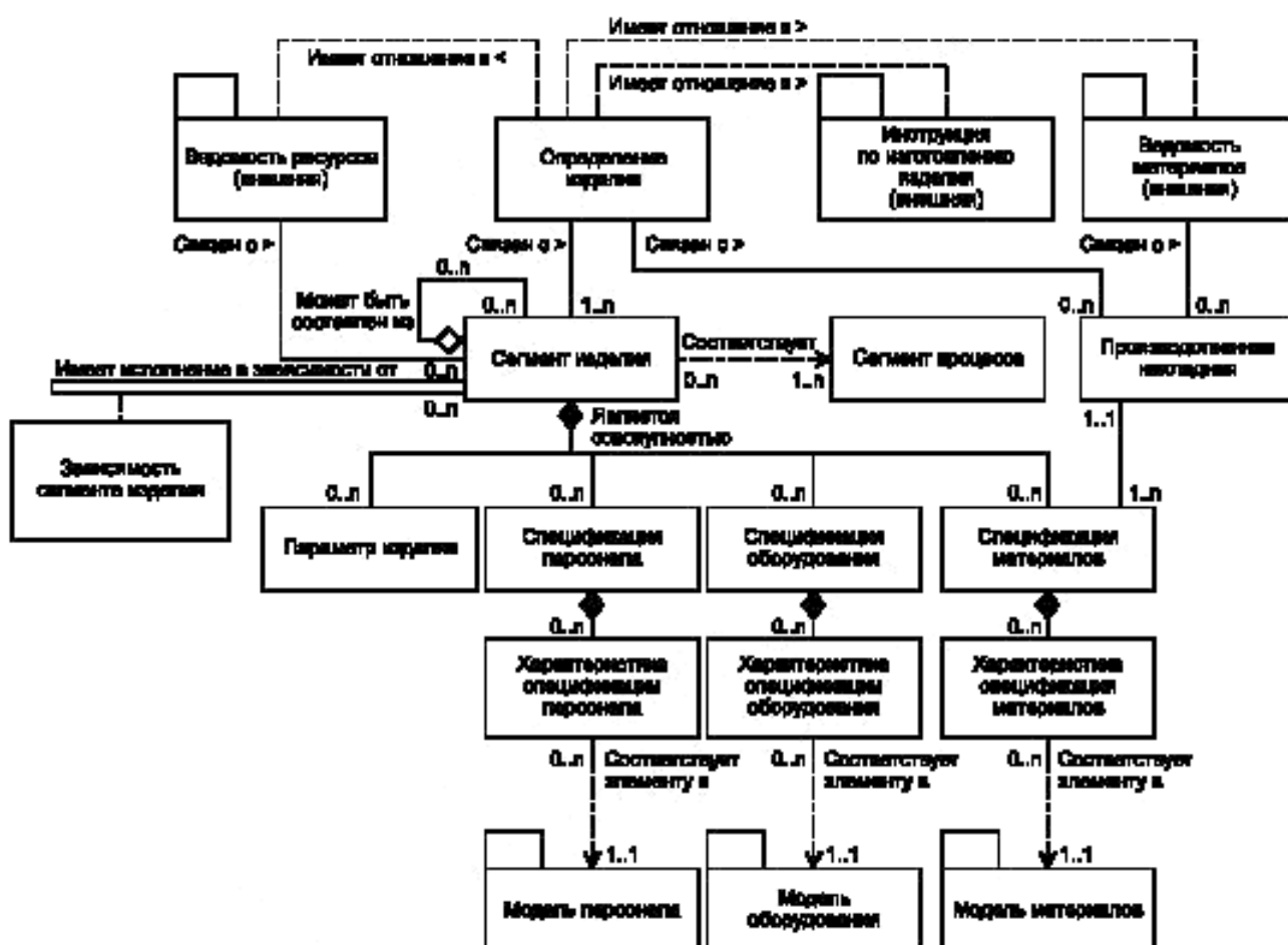
Рисунок 8 — Модель определения изделия
