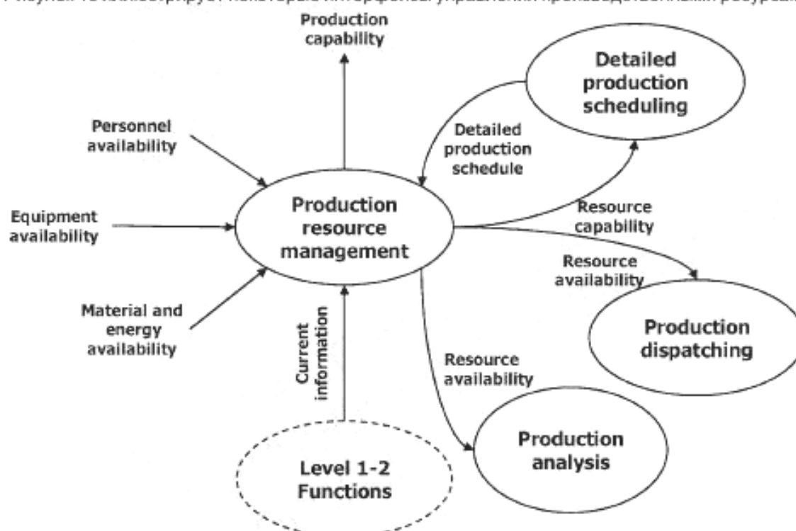
Рисунок 16 — Интерфейсы модели управления производственными ресурсами
