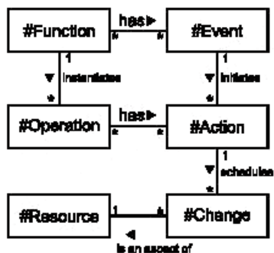
Рисунок G.2 — Онтология PSLX, часть 2
