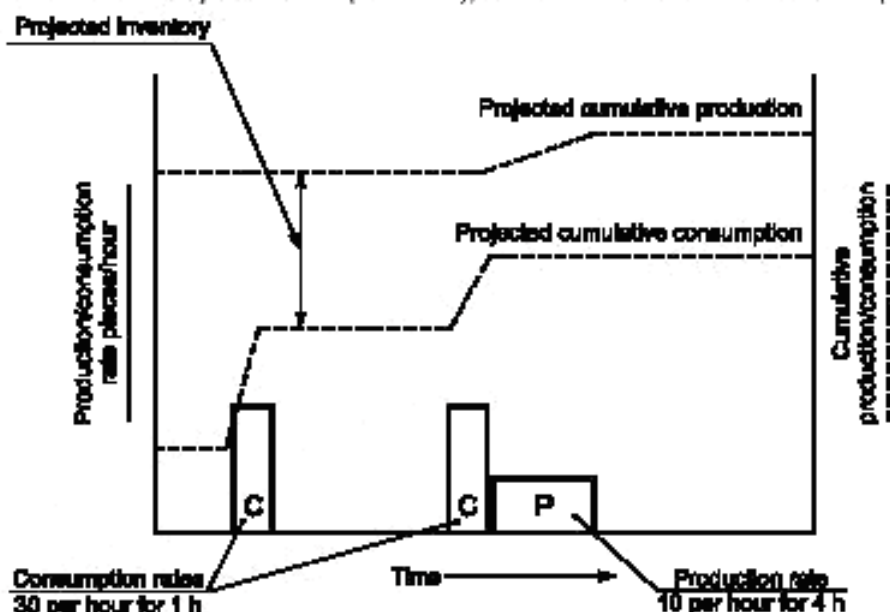
Рисунок 13 — Прогнозируемые производственные ресурсы для расходуемого ресурса
