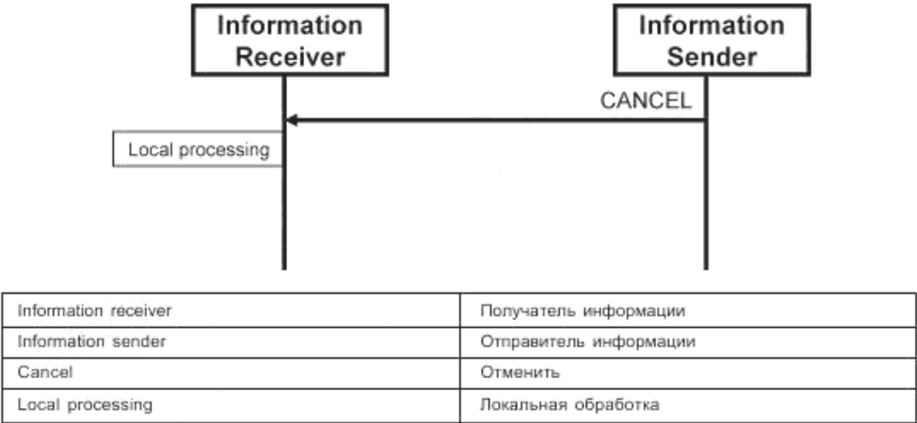
Рисунок 10 — Сообщение CANCEL
