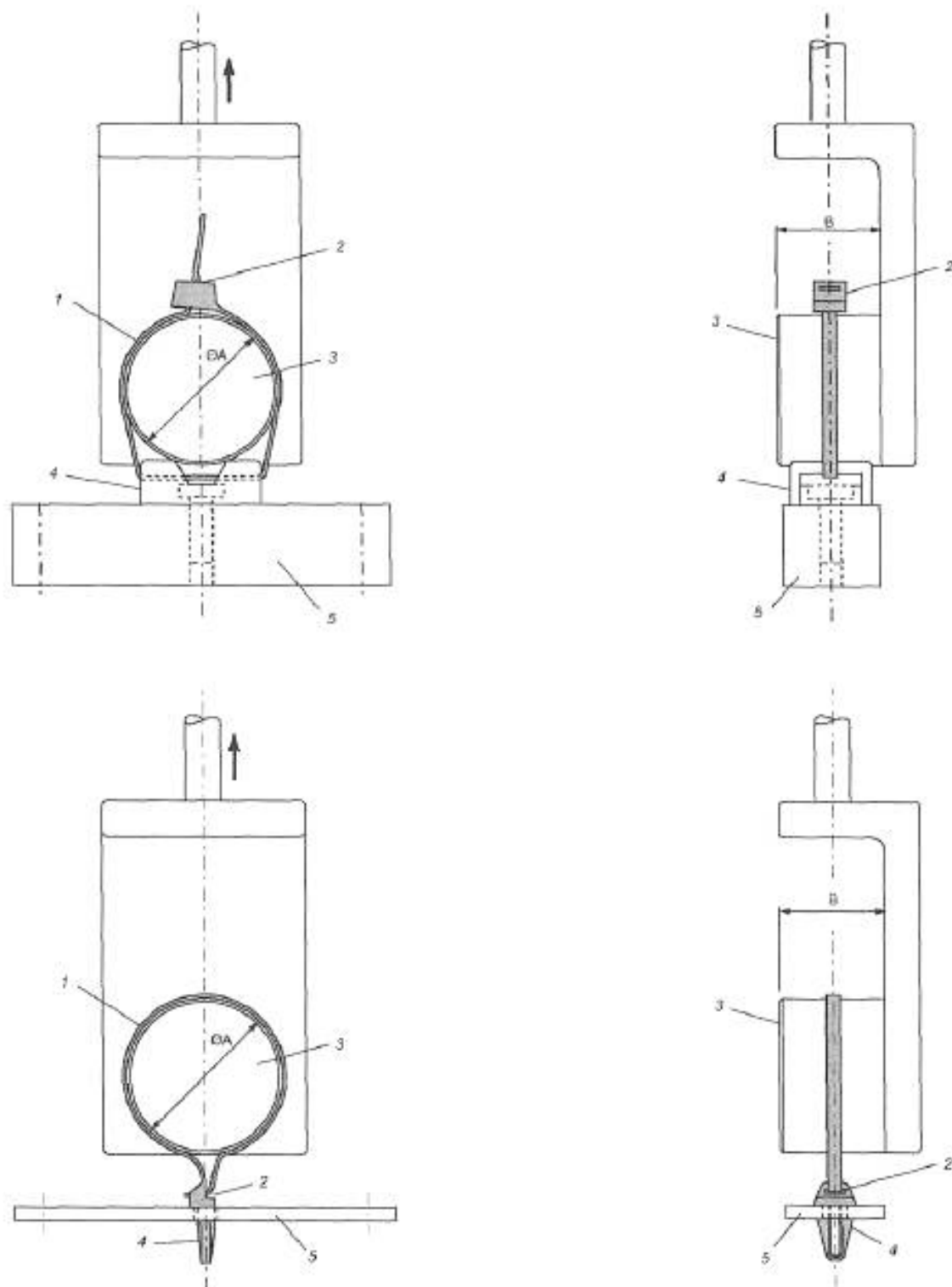
1 — кабельная стяжка; 2 — устройство захвата; 3 — оправка; 4 — устройство для фиксации; 5 — твердое основание; A — диаметр испытательной оправки; B — ширина испытательной оправки
