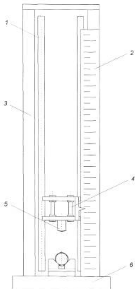
Рисунок 3а) — Испытательный стенд
