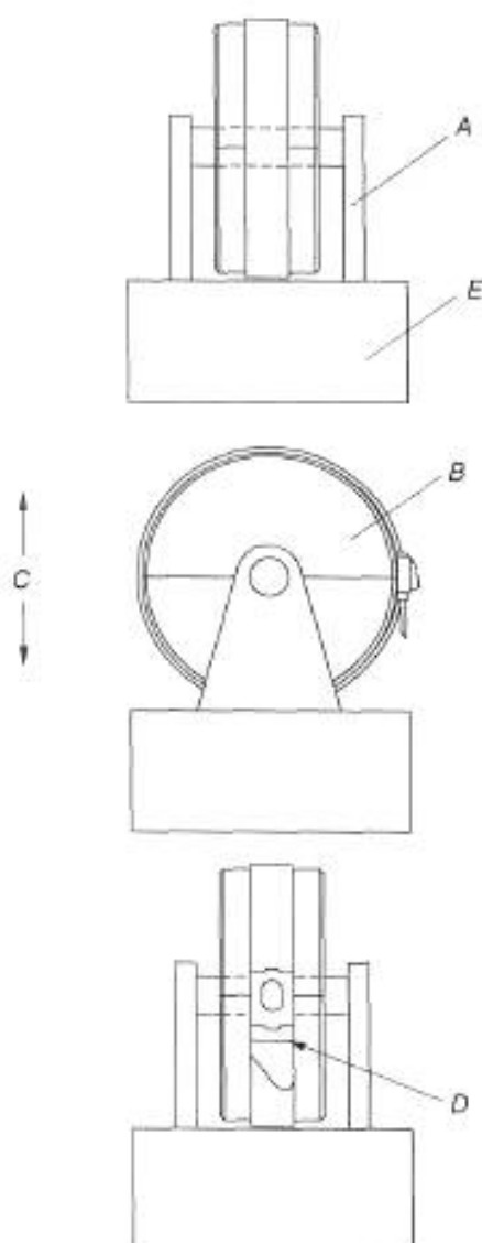
A — монтажный кронштейн; B — раздвижная оправка; C — направление вибрации; D — справочная отметка на ремешке; E — вибрационный стол
