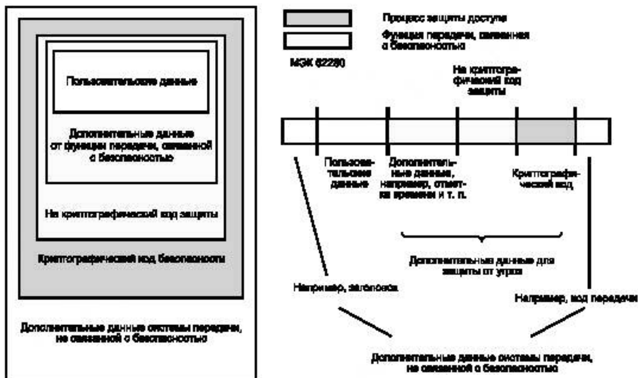
Рисунок С.5 — Модель представления сообщения в системе передачи (тип В1)
