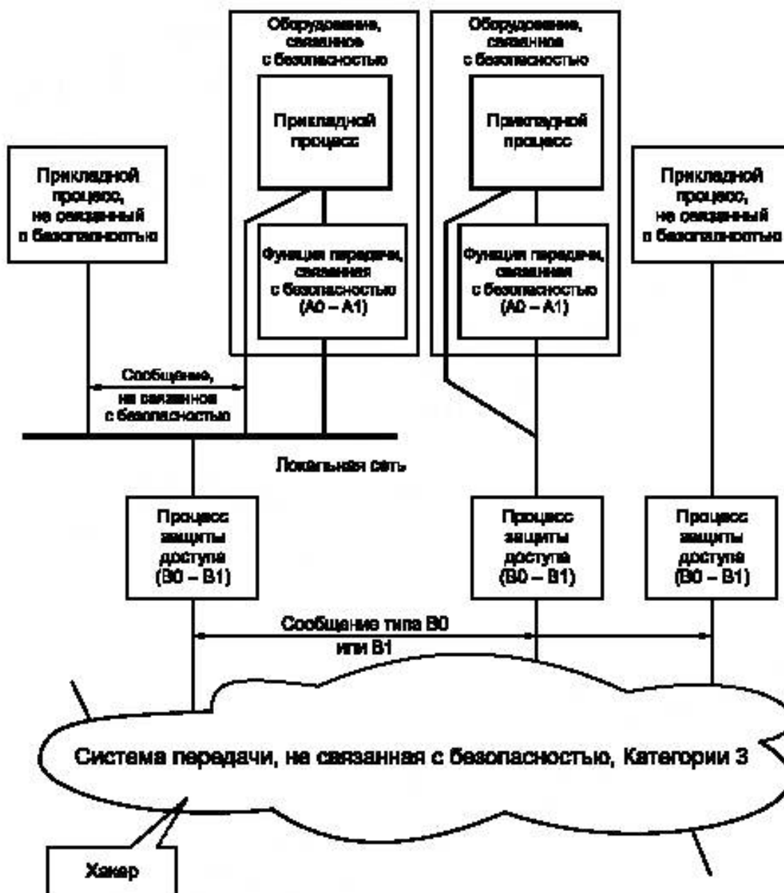
Рисунок С.7 — Коммуникация между связанными и не связанными с безопасностью приложениями
