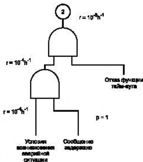
Рисунок D.3 — Дерево отказов для случая 2
