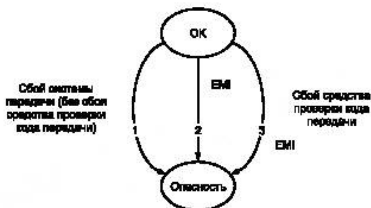
Рисунок С.6 — Базовая модель ошибки
