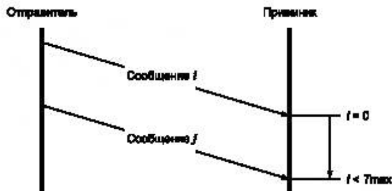
Рисунок 2 — Циклическая передача сообщений
