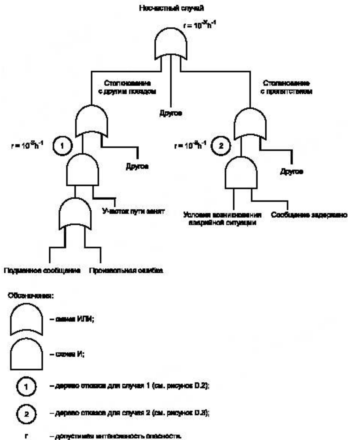
Рисунок D.1 — Дерево отказов для опасности «авария»
