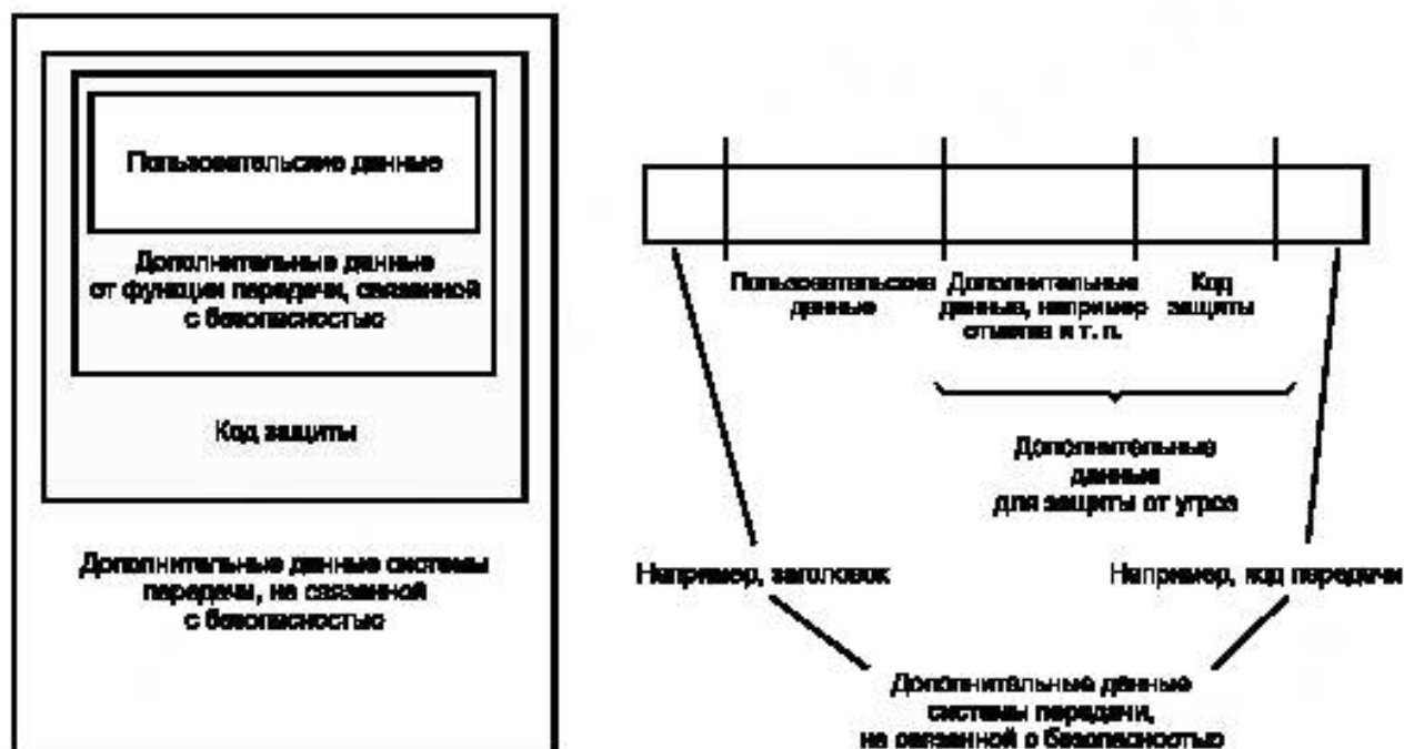
Рисунок С.2 — Модель представления сообщения в системе передачи (тип A0, A1)
