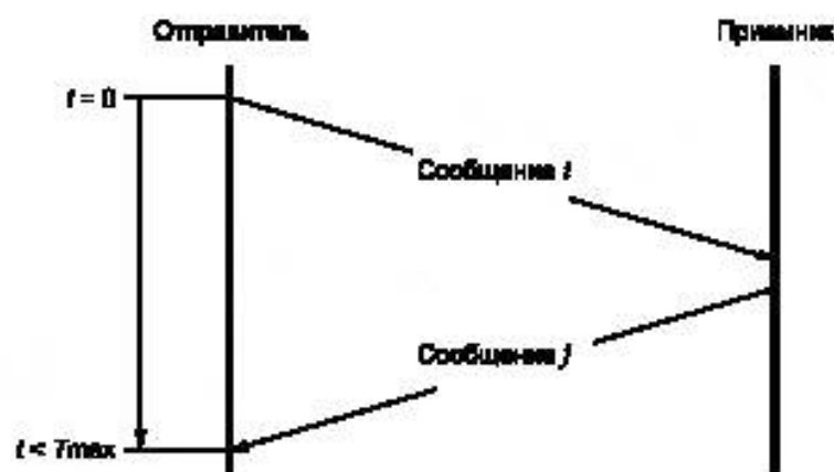
Рисунок 3 — Двухнаправленная передача сообщений
