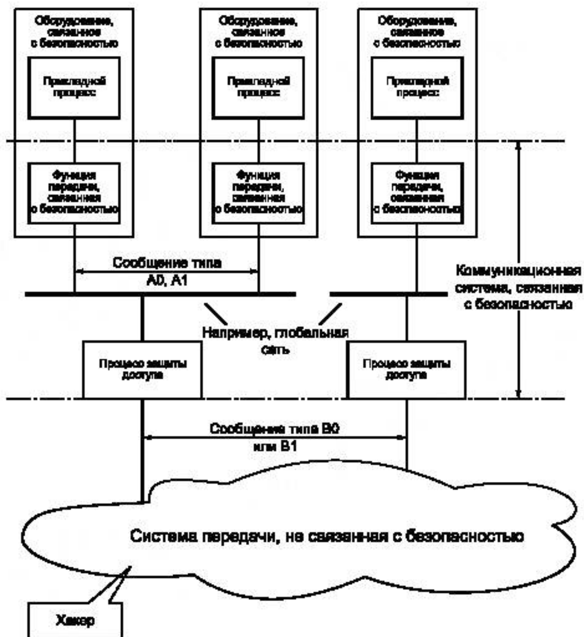
Рисунок С.3 — Использование отдельного слоя защиты доступа
