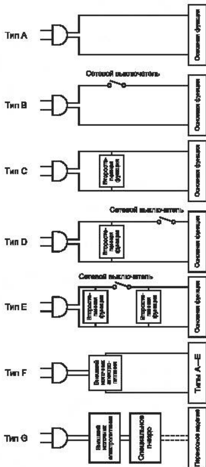
Рисунок A.1 — Принципиальные схемы типов приборов
