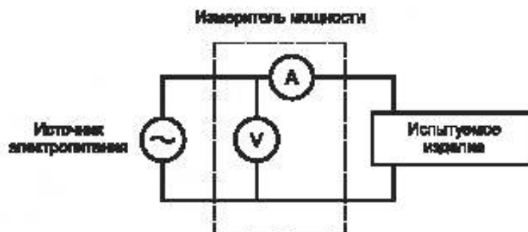
Рисунок В.3 — Схема расположения для прибора, питаемого непосредственно от сети питания переменного тока для нагрузок большой мощности
