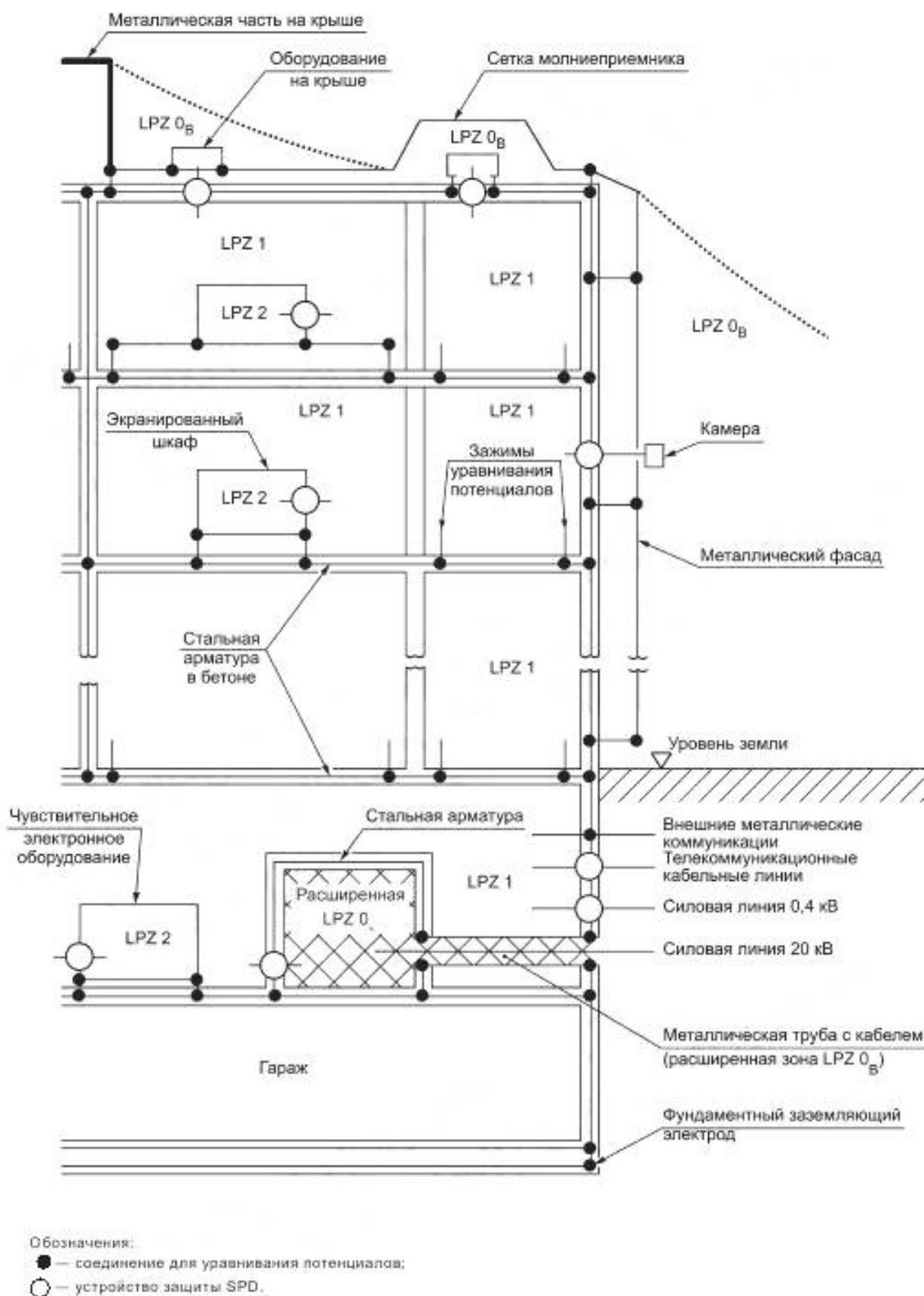
Рисунок А.6 — Пример применения мер защиты SPM офисного здания
