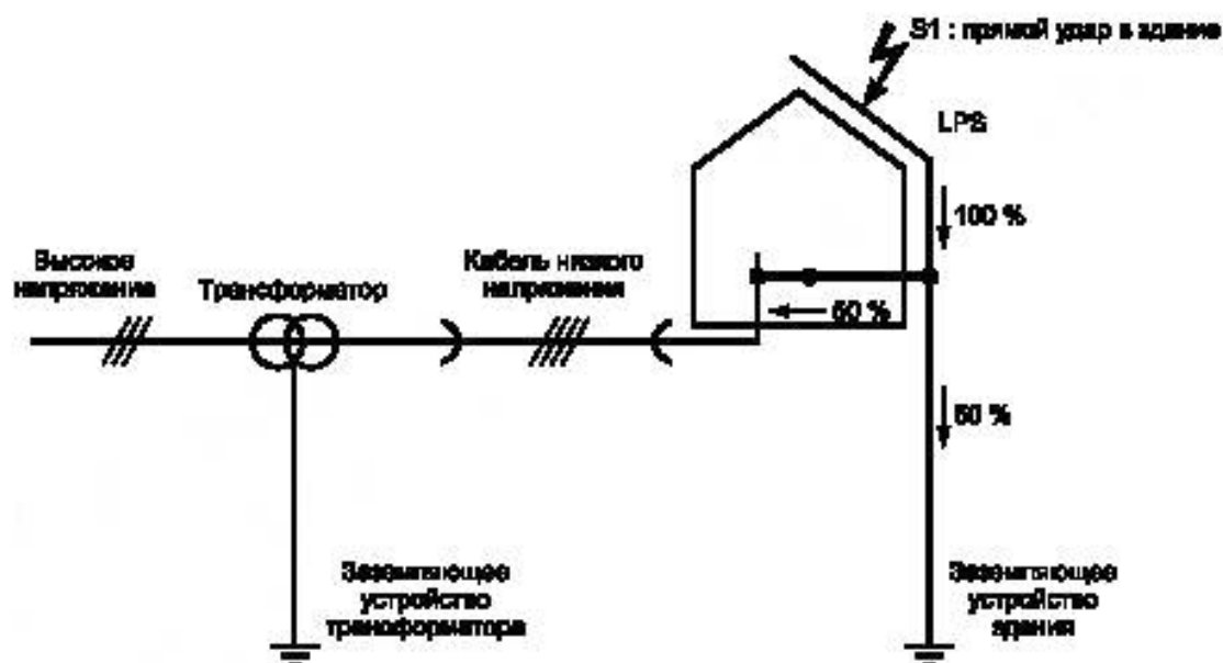
Рисунок D.3 — Характерный пример сбалансированного распределения тока
