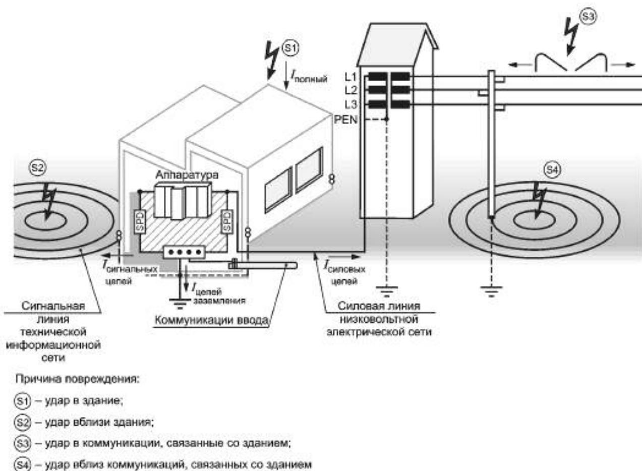
Рисунок D.2 — Характерный пример различных причин повреждения здания и распределения тока молнии внутри системы
