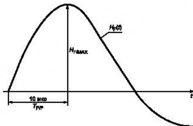
Рисунок А.2а — Моделирование нарастания магнитного поля первого положительного удара молнии (10/350 мкс) при помощи одиночного импульса 8/20 мкс (затухающее колебание 25 кГц)
