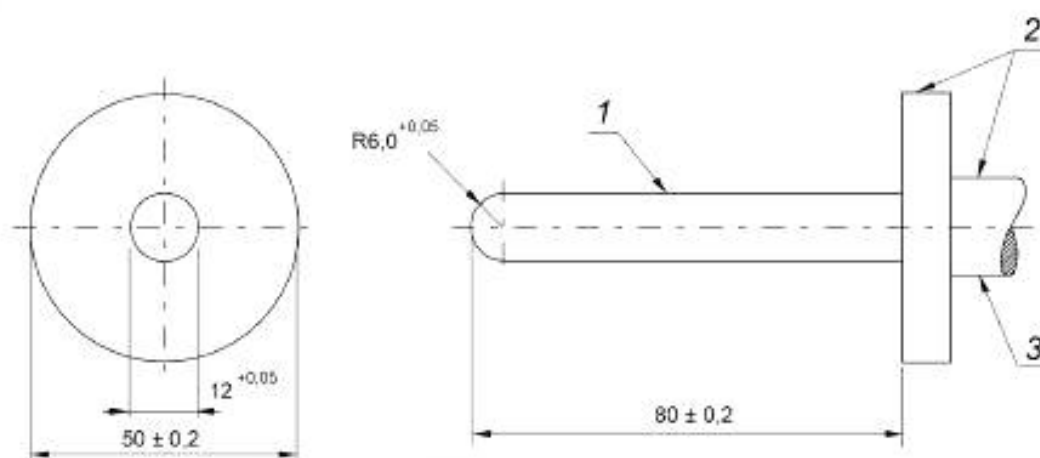
Рисунок 2 — Испытательный штырек
