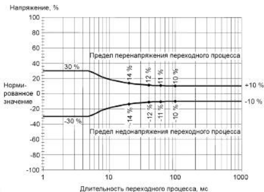
Рисунок В.1 — Допустимые отклонения источника классификации 1
