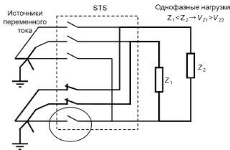
Рисунок D.1 — Изменение напряжения нагрузки при отказе переключателя нейтралей
