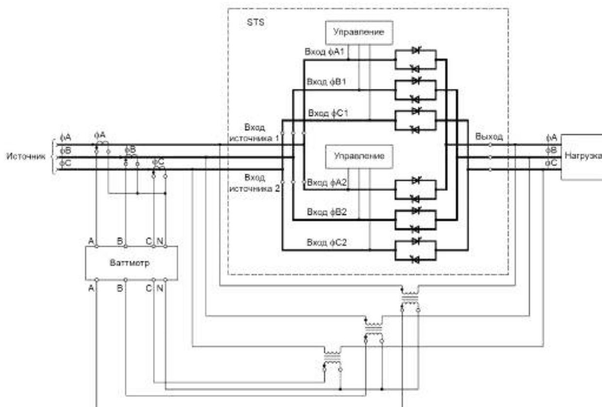
Рисунок 4 — Типовая схема для измерения потерь проводимости
