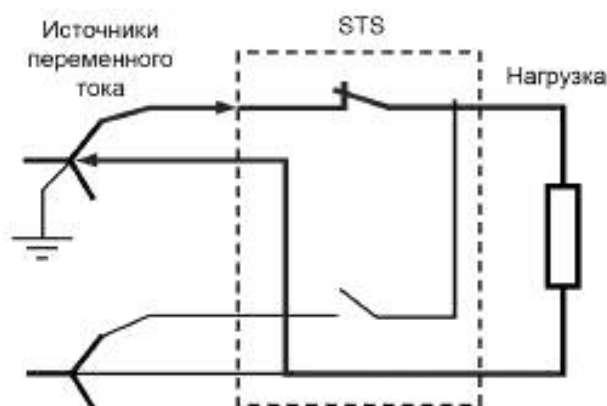
Рисунок С.1 — Замкнутые нейтраль STS с общим заземлением входных источников переменного тока (соответствующих протеканию тока нагрузки)
