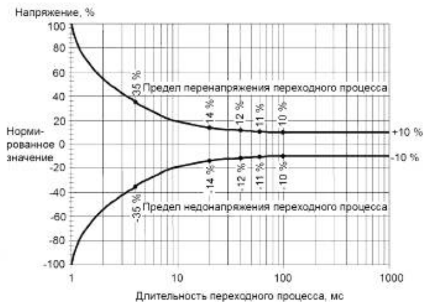
Рисунок В.2 — Допустимые отклонения источника классификации 2
