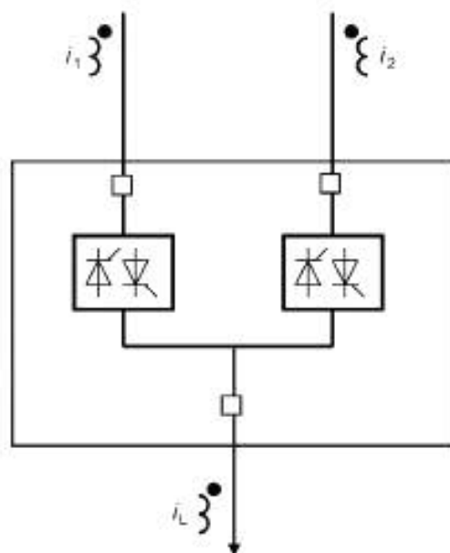
Рисунок 3 — Испытание поперечного тока STS
