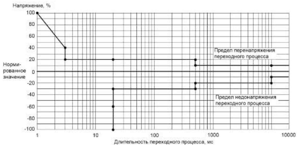
Рисунок В.4 — Допустимые отклонения источника классификации 4
