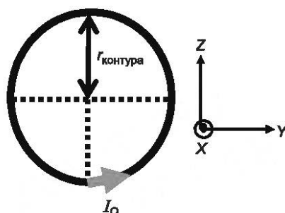
Рисунок С.5 — Схематическое изображение контура круглой формы
