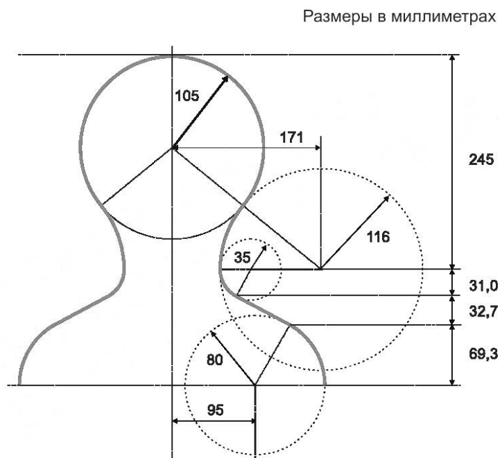
Рисунок С.3 b) — Детальный чертеж модели головы и плеч
