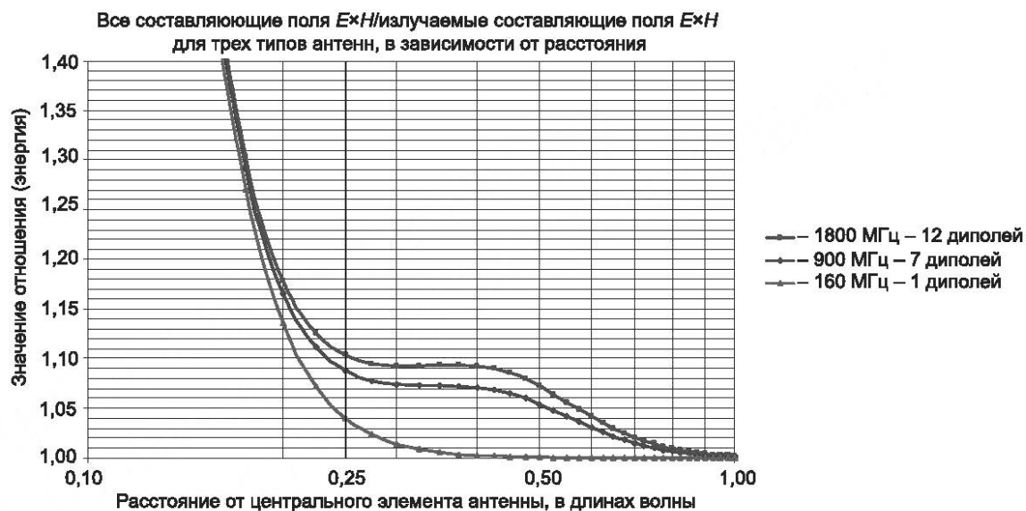
Рисунок А.4 — Соотношение компонентов поля E \cdot H для трех типов антенн
