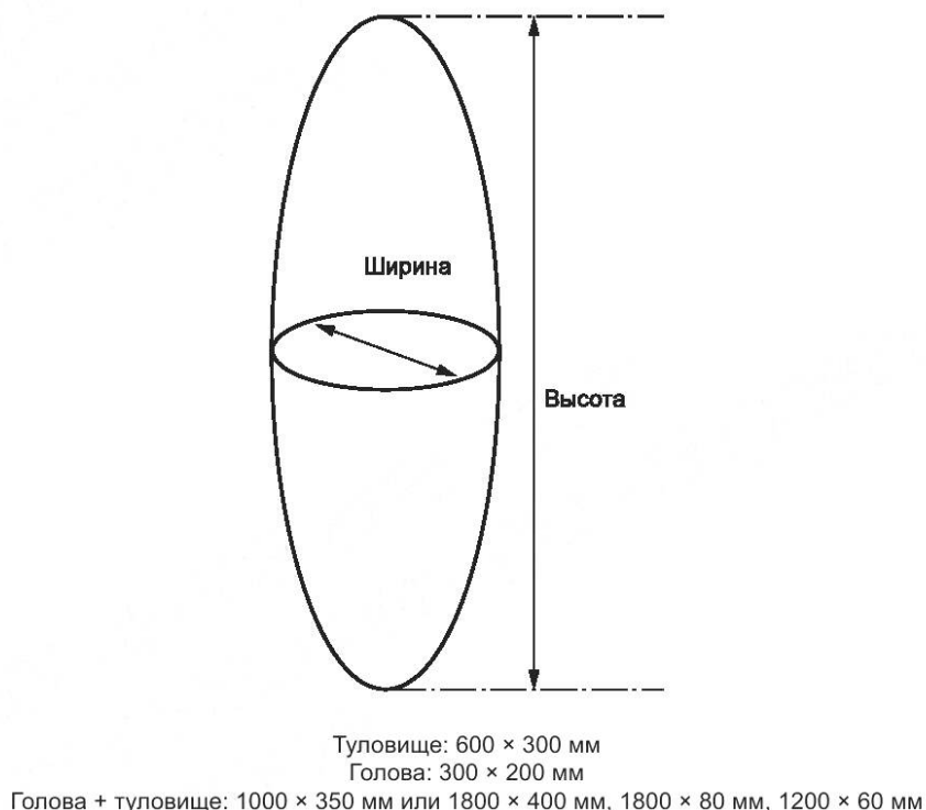
Рисунок С.1 — Цифровая модель однородного сфероида
