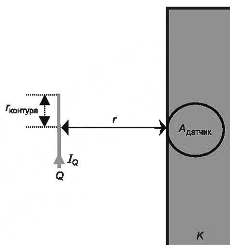
Рисунок С.15 — Расположение источника Q, датчика и модели K
