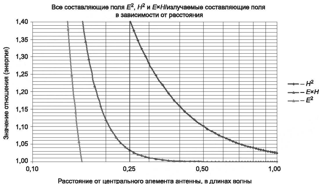
Рисунок А.3 — Соотношение компонентов поля E^2 , H^2 и E \cdot H
