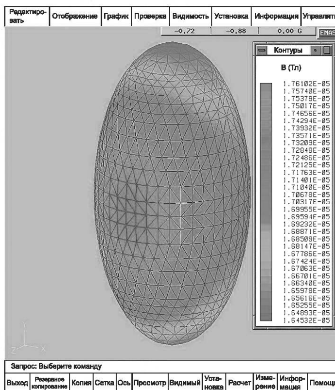
Рисунок С.12 а) — Магнитное поле
