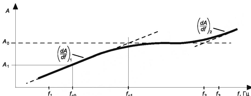
Рисунок 4 — Передаточная функция A
