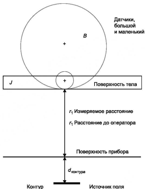
Рисунок С.20 — Расстояния между источником поля, корпусом прибора и поверхностью тела человека
