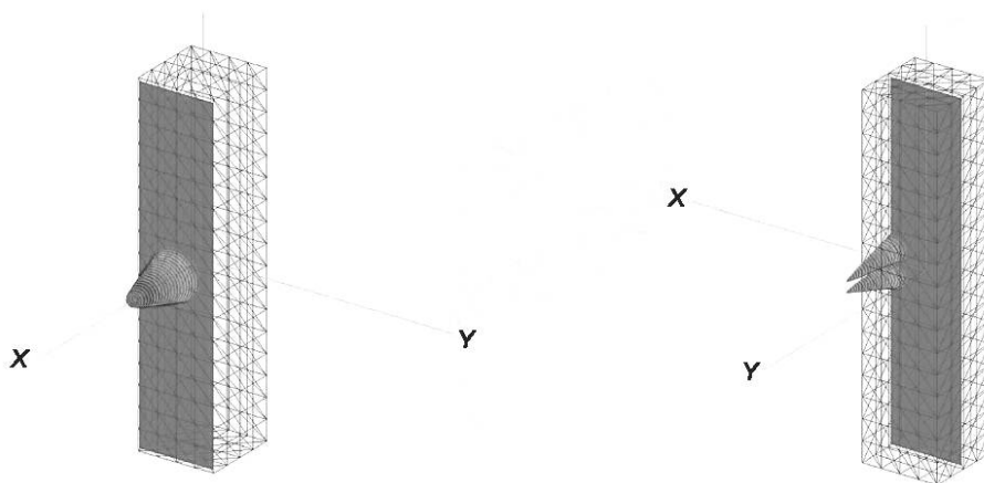
Рисунок C.8 — Распределение плотности электрического тока J в плоскостях x = +0,2 м (левая часть рисунка) и y = 0,0 м (правая часть рисунка)
