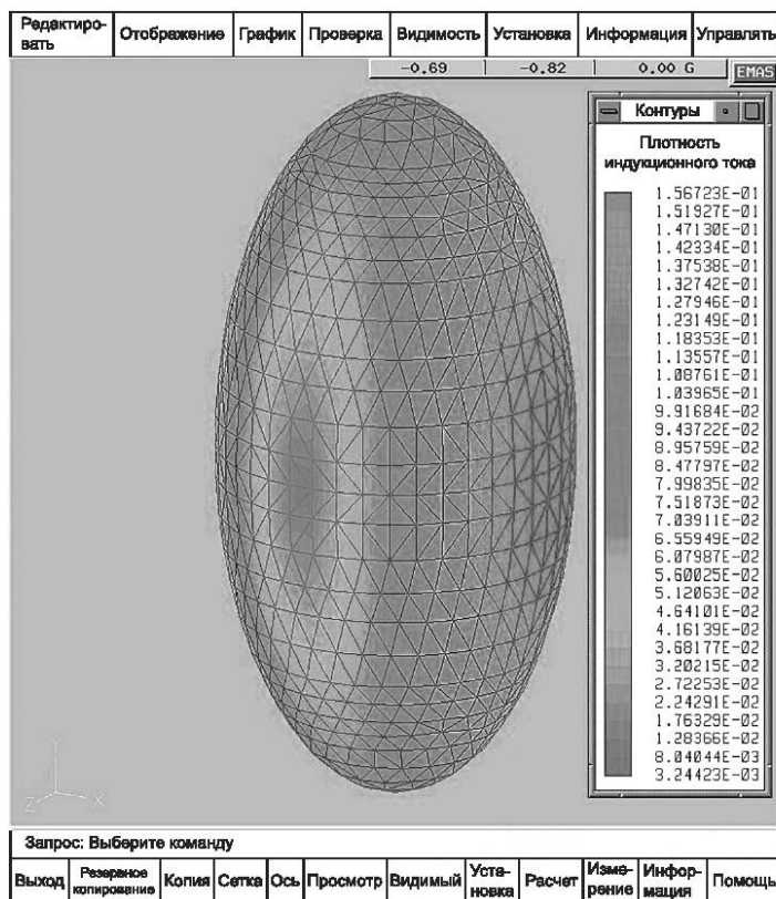
Рисунок С.12 б) — Плотность индуцированного тока
