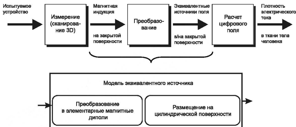
Рисунок С.6 — Блок-схема метода
