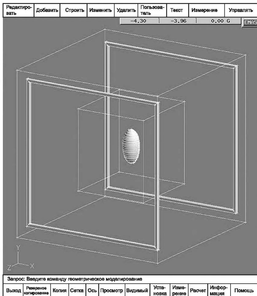
Рисунок С.9 — Катушки Гельмгольца и вытянутый сфероид
