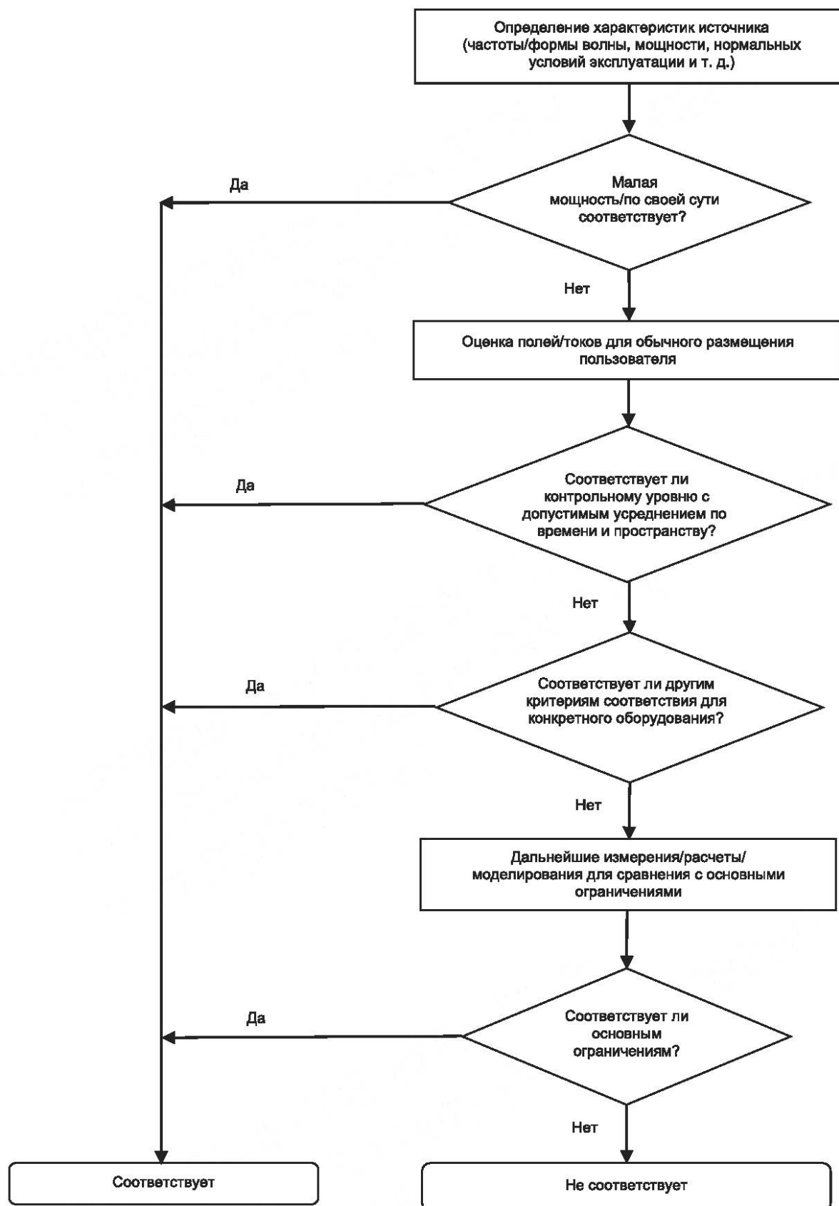
Рисунок 1 — Блок-схема процесса оценки соответствия
