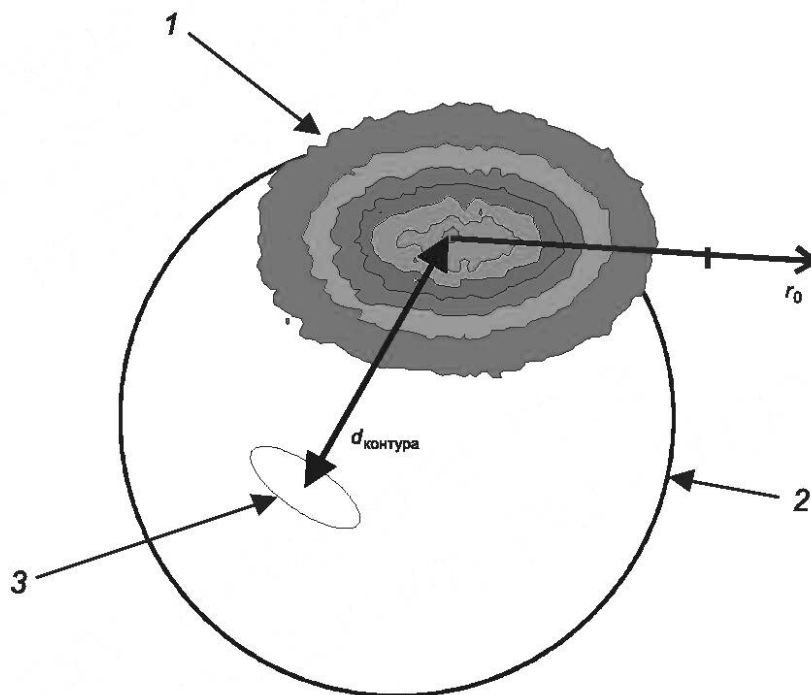
1 — измерение по касательной плоскости вблизи точки с максимальным значением магнитной индукции; 2 — модель бытового прибора в виде сферы; 3 — катушка как эквивалент источника поля
