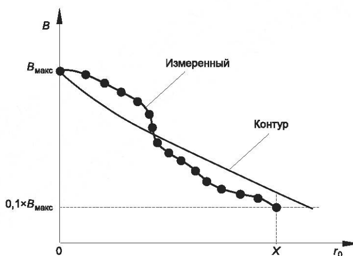
Рисунок С.19 — Градиент измеренной магнитной индукции и магнитной индукции, создаваемой контуром
