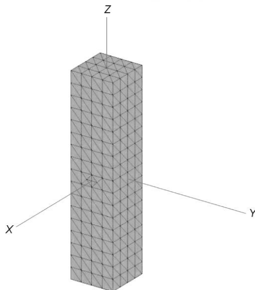
Рисунок С.2 — Цифровая модель однородного кубоида
