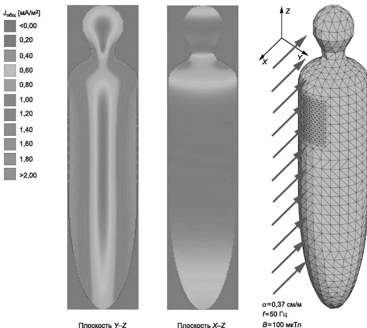
Рисунок С.13 — Распределение плотности индуцированного электрического тока
