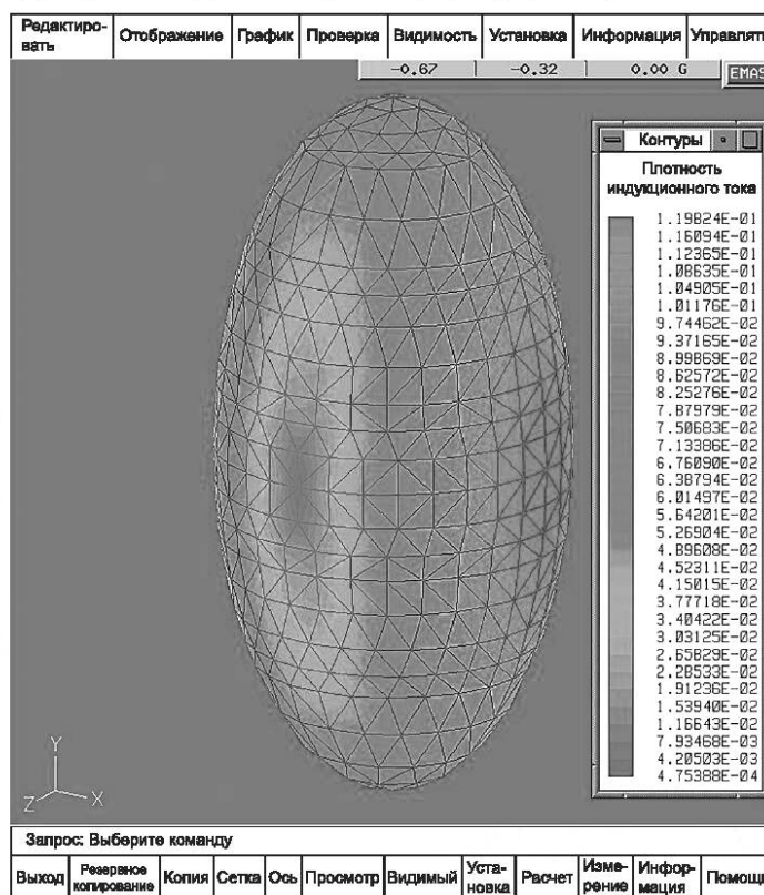
Рисунок С.11 — Плотность индуцированного тока
