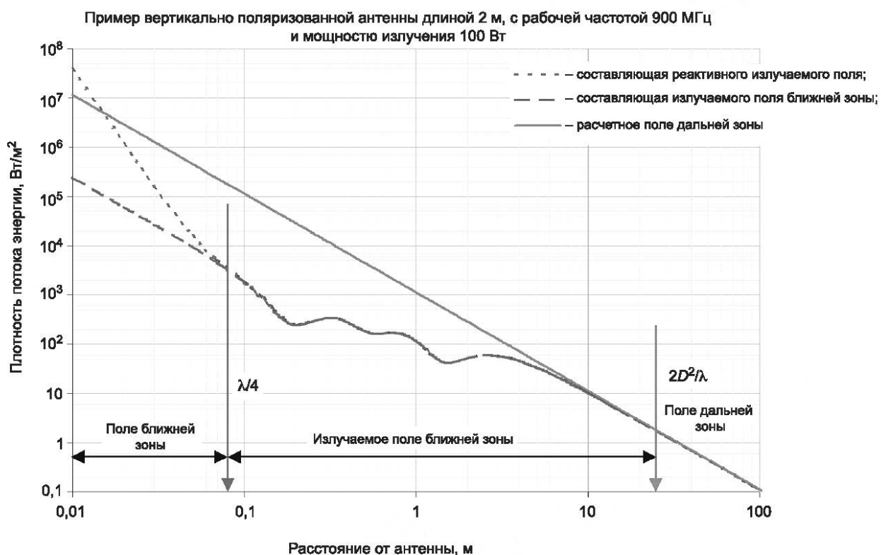
Рисунок А.5 — Поле дальней зоны — прямая линия, излучаемое поле ближней зоны — нижняя линия, поле ближней зоны — другая нижняя линия
