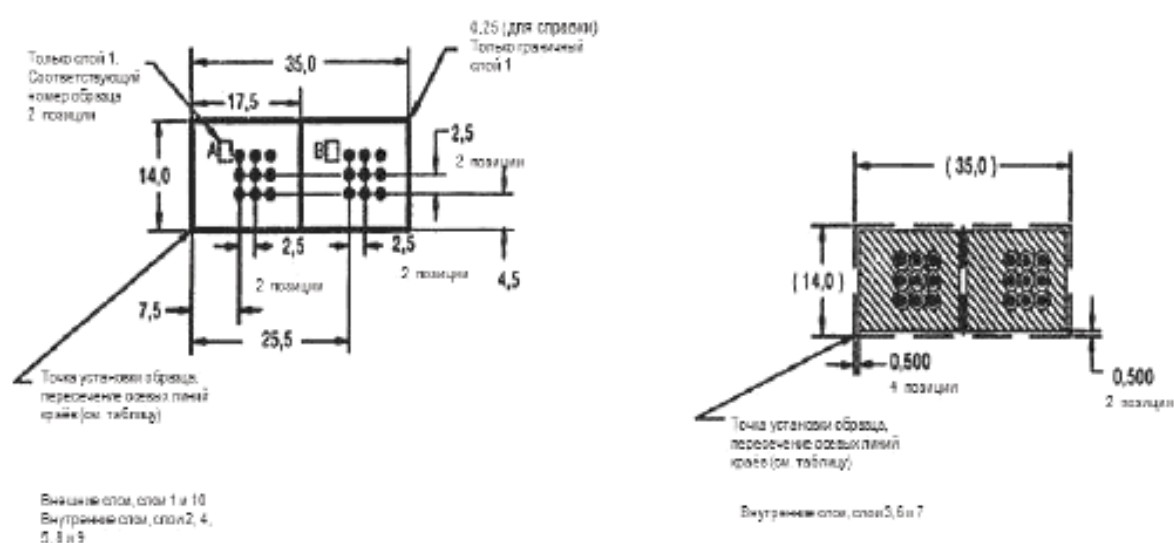
Рисунок 1а – Образцы для испытания А и В
