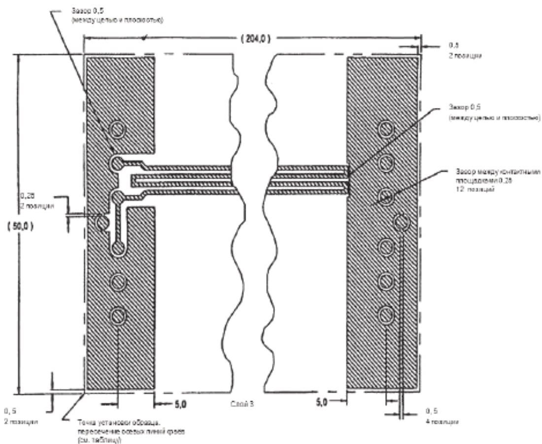
Рисунок 1h – Образцы для испытания N2 и N3 – продолжение
