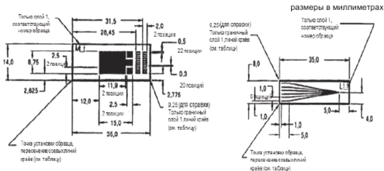
Рисунок 1m— Образцы для испытания L и M
