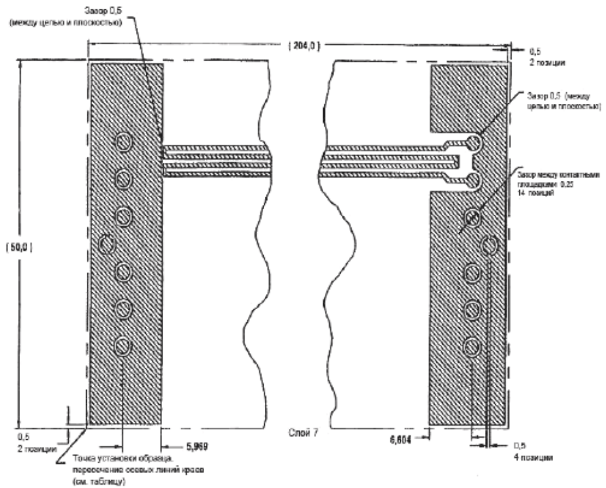
Рисунок 11 – Образцы для испытания H2 и H3 – продолжение
