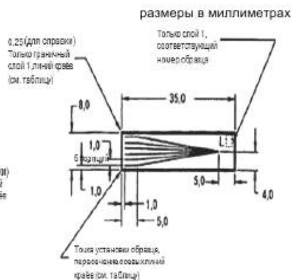
Рисунок 1m— Образцы для испытания L и M
