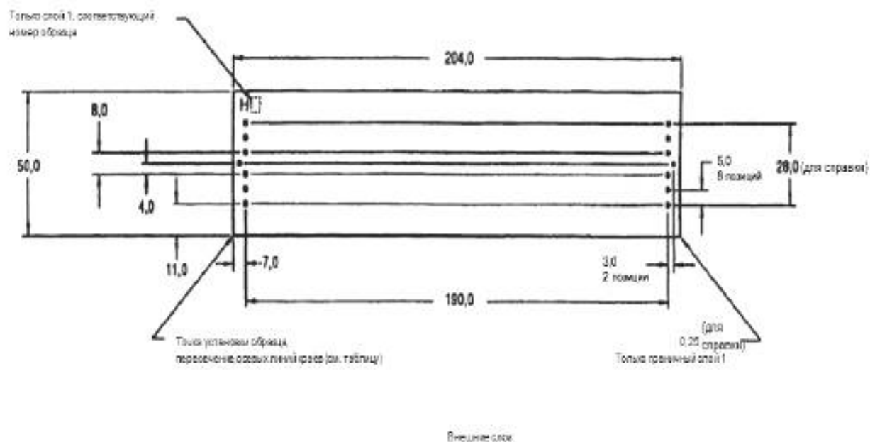
Рисунок 1f— Образец для испытания H
