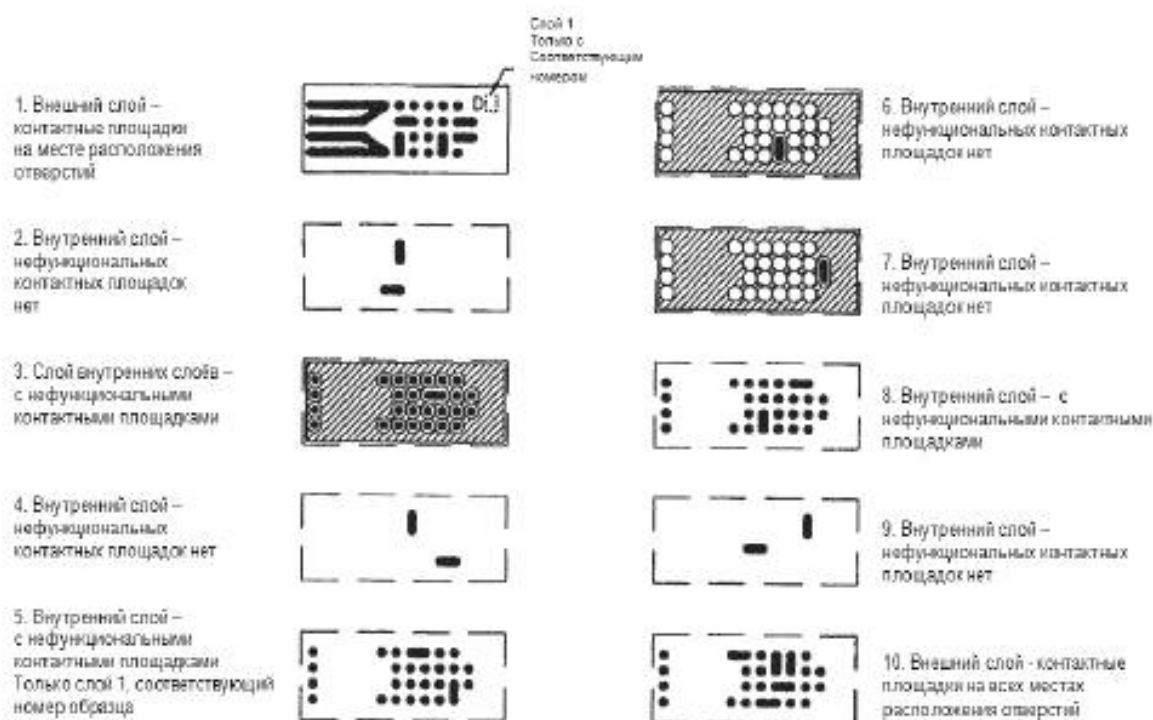
Рисунок 1с – Образец для испытания D (окончание)
