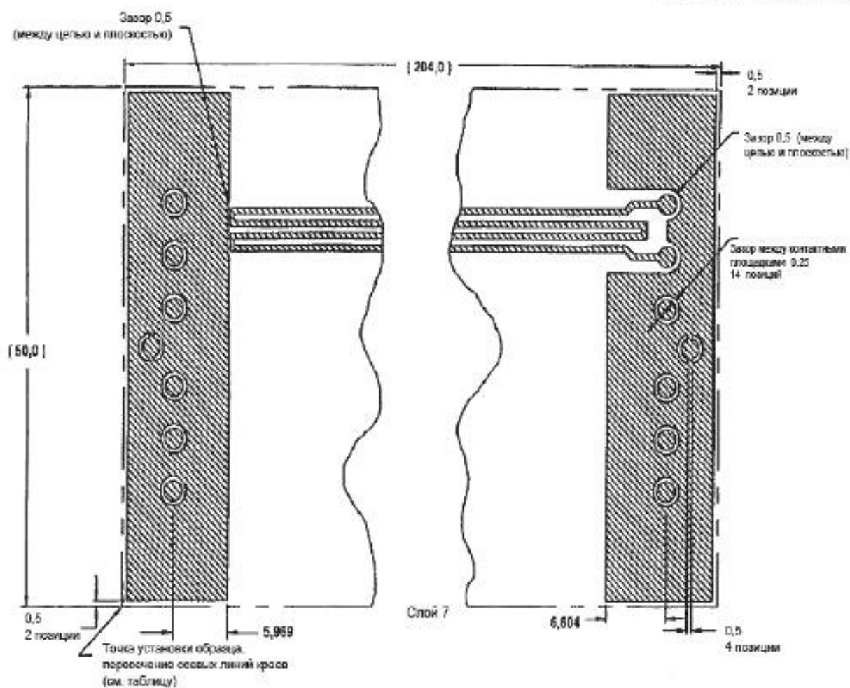
Рисунок 11 – Образцы для испытания Н2 и Н3 – продолжение
