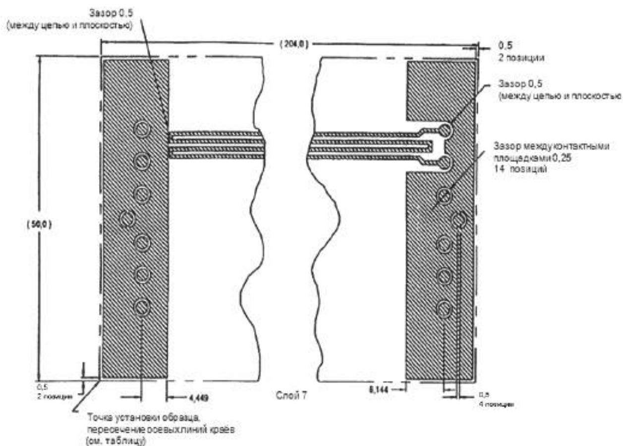
Рисунок 1к – Образец для испытания Н1 – продолжение
