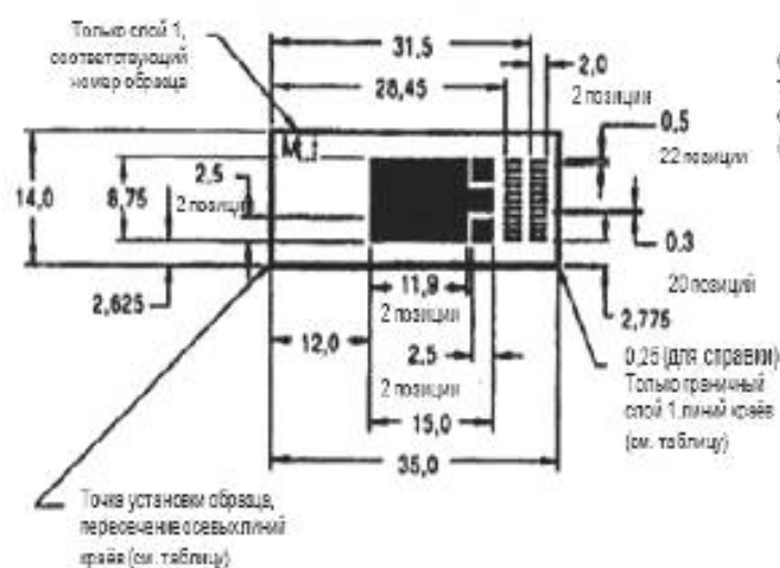
Рисунок 1m— Образцы для испытания L и M
