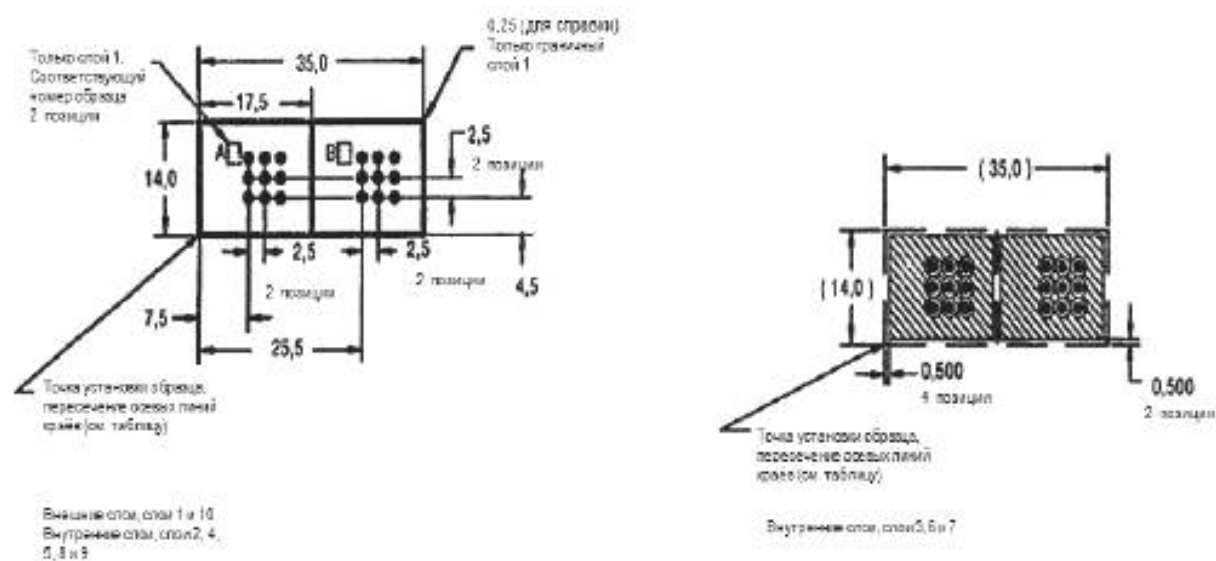
Рисунок 1а – Образцы для испытания А и В
