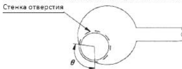
Рисунок 5 – Минимальная ширина W_2 кольца внутренней контактной площадки
