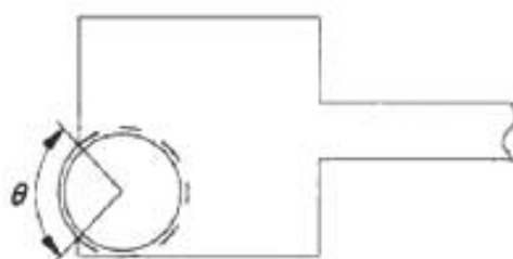
Рисунок 6 – Разрыв в отверстии (обрезание контактной площадки)
