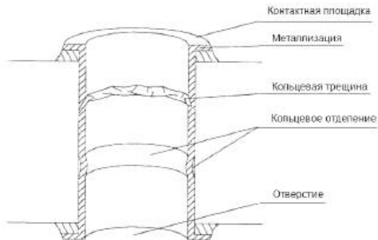
Рисунок 2 – Кольцевые дефекты
