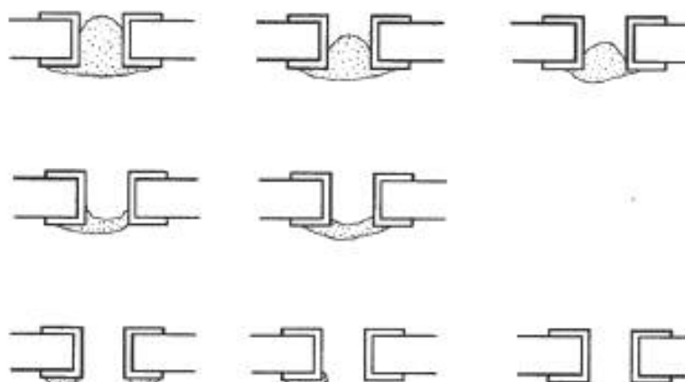
Рисунок 7 – Примеры паяных отверстий
