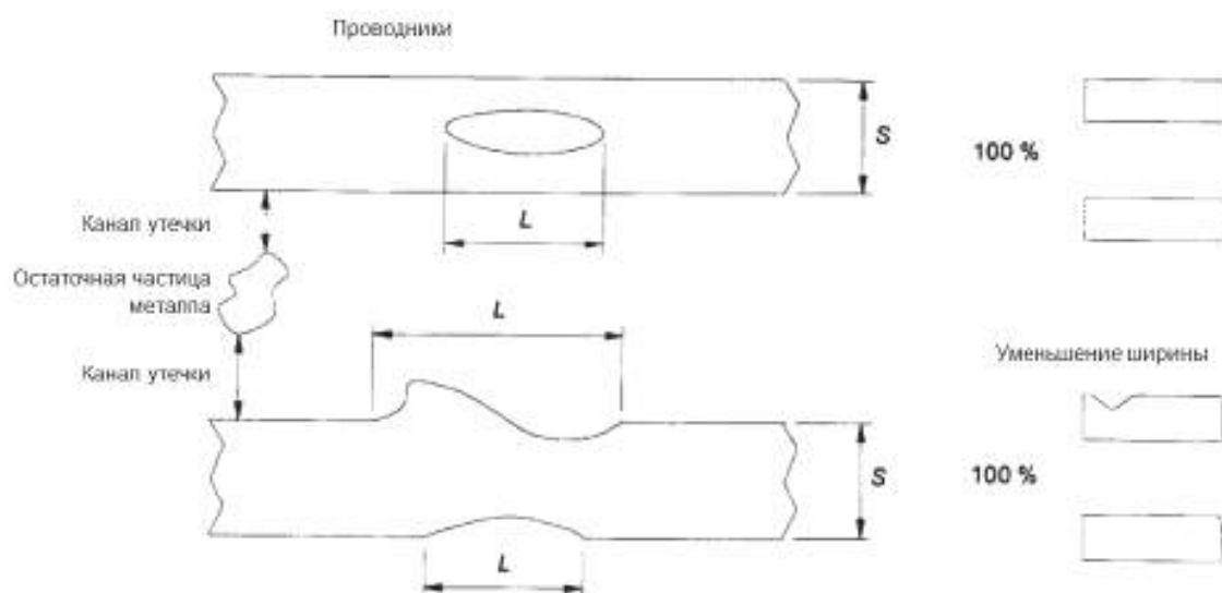
Рисунок 3 – Дефекты проводящего рисунка
