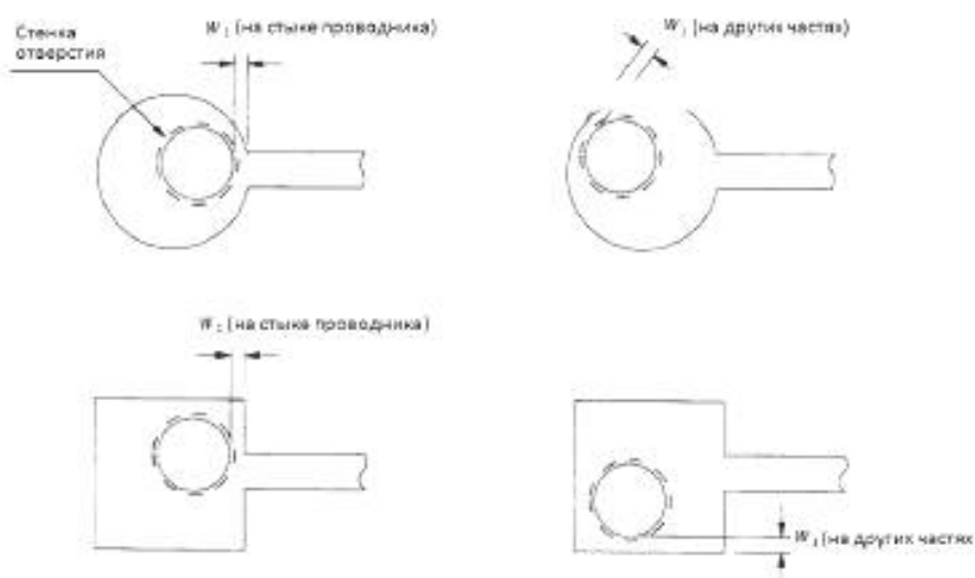
Рисунок 3 – Дефекты проводящего рисунка
