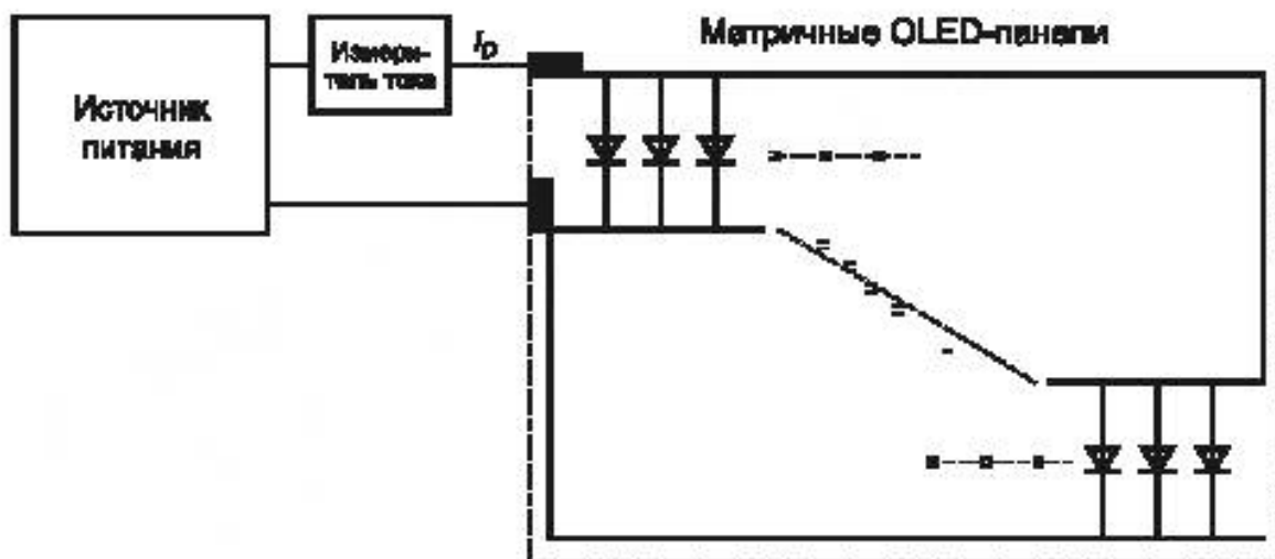
Рисунок В.1 — Пример конфигурации оборудования при измерении эффективности яркости по току
