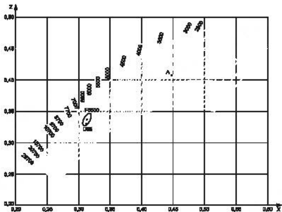
Рисунок D.2 — Кривая абсолютно черного тела (кривая Планка) и изотермические линии согласно CIE 1931 XYZ
