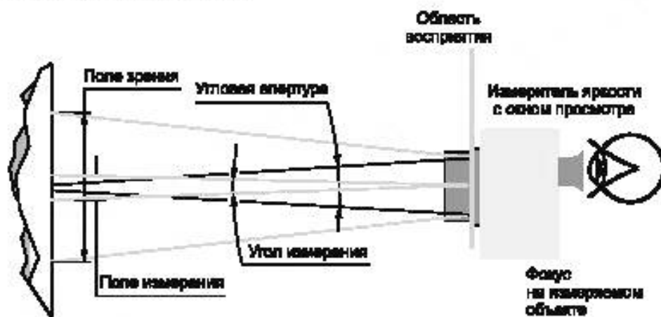
Рисунок 1 — Схема компоновки измерительной установки
