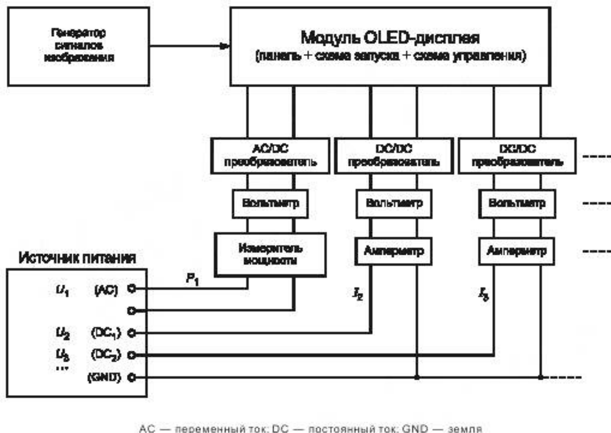
Рисунок 6 — Пример установки для измерения потребляемой мощности
