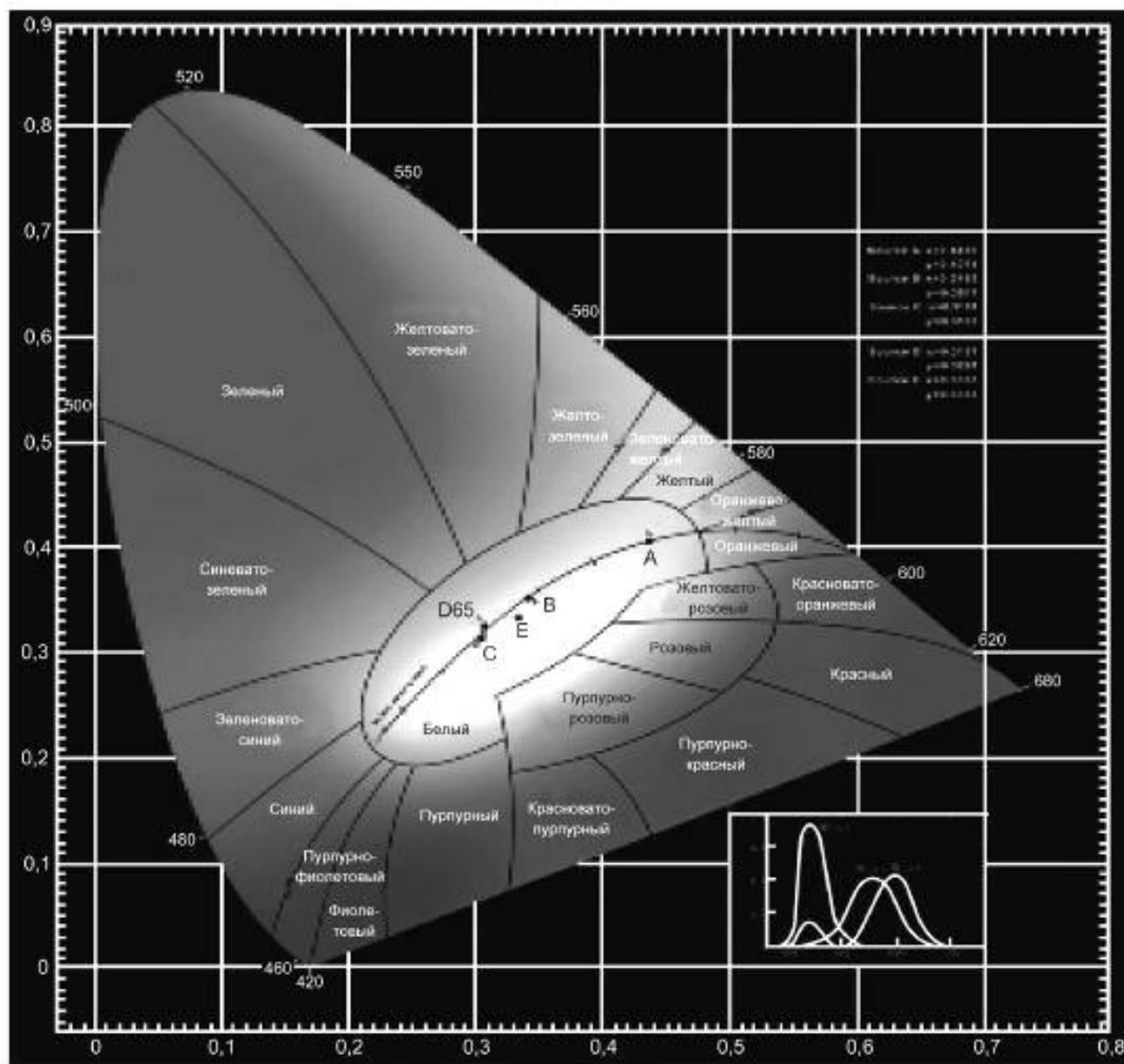
Рисунок D.1 — График цветности XYZ CIE 1931
